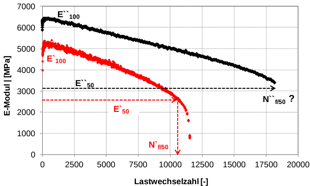
Abbildung 6. Verlauf des E-Moduls in Abhängigkeit von der Lastwechselzahl, festgestellt in Zug-Schwellversuchen durchgeführt bei 10 °C (schwarz) und 20 °C (rot).
