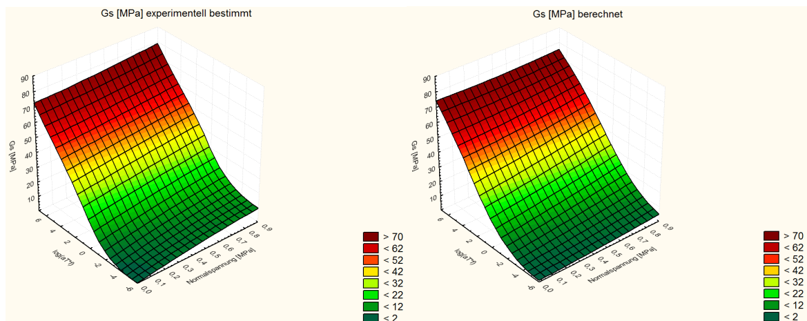
Abbildung 4.8: Flächenplot aus den versuchstechnisch ermittelten Schersteifigkeitswerten (links) und mit Gleichung 24 bestimmtes Flächendiagramm (rechts)
