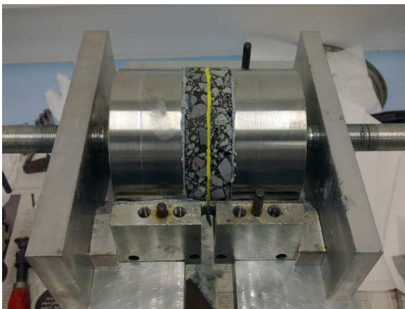
Abbildung 5.9: Einkleben eines 30 mm langen zweischichtigen Asphaltprobekörpers und zwei Stahldummies
