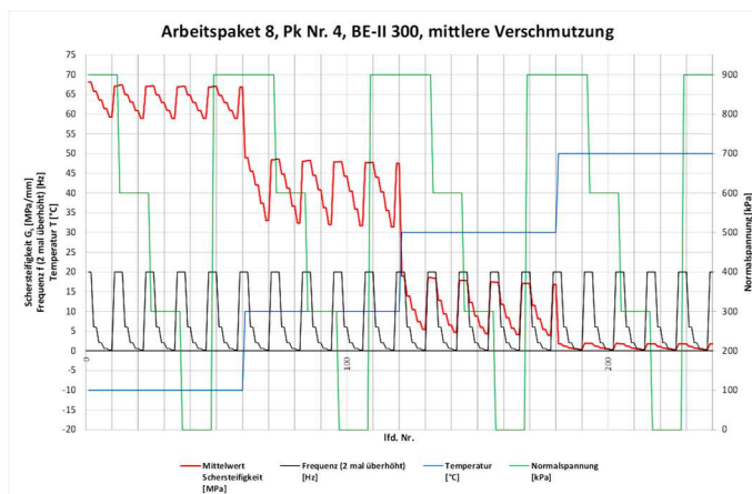
Abbildung 4.4: Beispiel einer Schersteifigkeit, die durch die Normalspannung nicht beeinflusst wird
