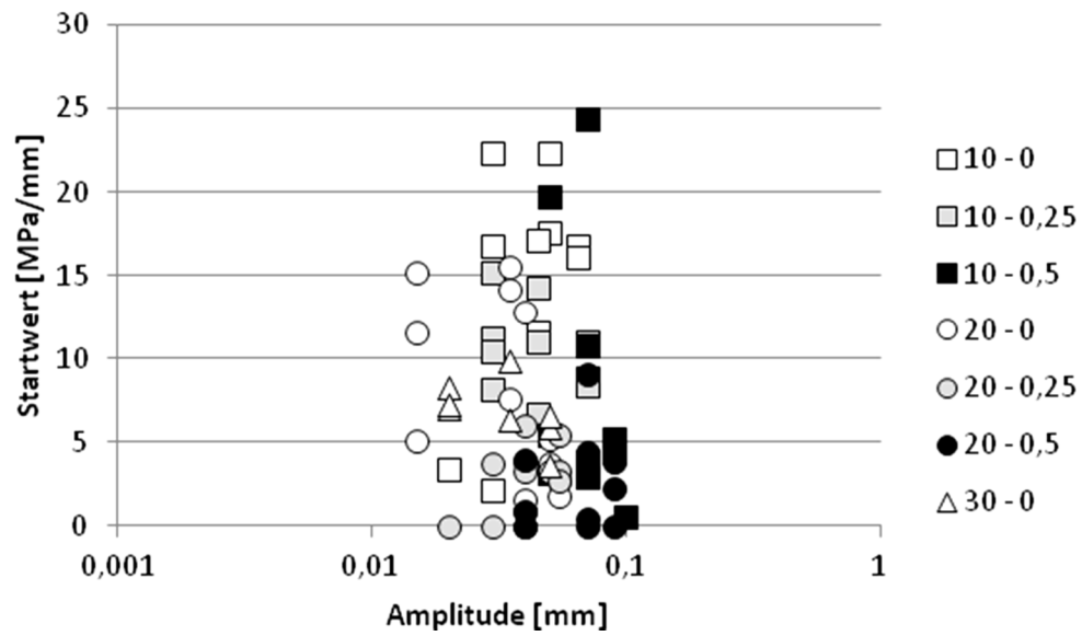
Abbildung 82. Verbundvariante C: Darstellung der Werte des Parameters a_1 über die Scher-amplitude.
