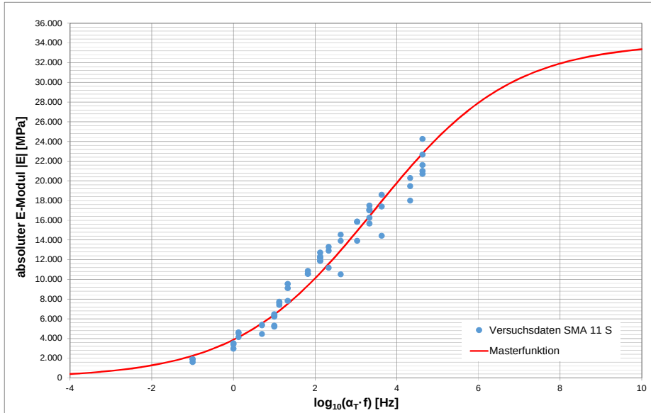
Abbildung 5.70: Masterfunktion des absoluten E-Moduls für SMA 11 S in Abhängigkeit von der korrigierten Frequenz ( f_{\text{korr}} )
