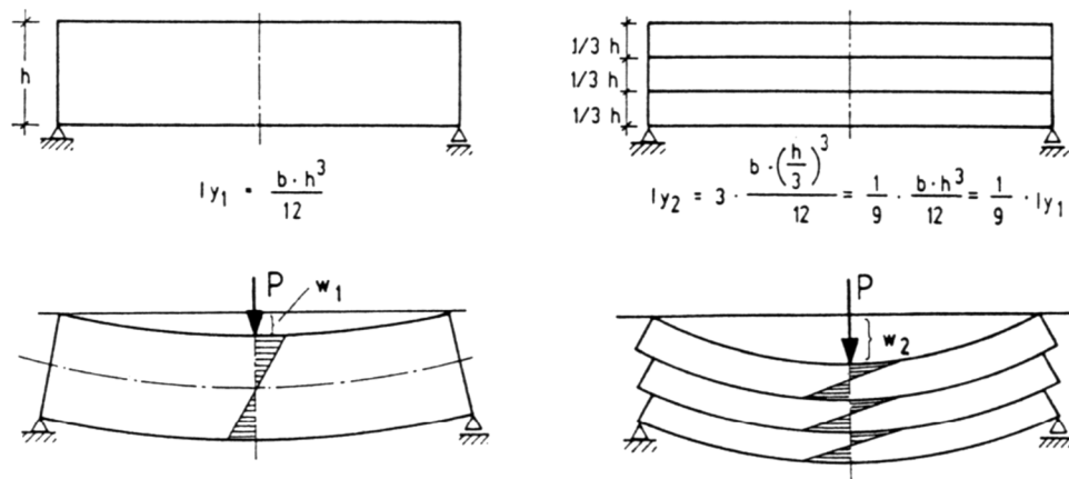
Abbildung 1.3: Darstellung des Spannungsverlaufes unterschiedlicher Verbundsysteme: (links) voller Verbund zwischen den Schichten und (rechts) Auflösung des Verbundes an den Schichtgrenzen (Weber, 1991).
