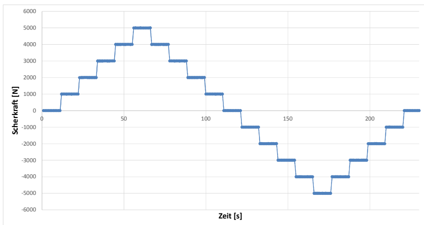
Abbildung 5.4: Verlauf der statisch aufgetragenen Scherkraft eines Zyklus
