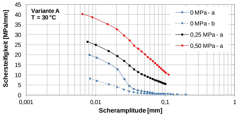
Abbildung 33. Verbundvariante A: Verläufe der Schersteifigkeiten bei drei Normalspannungen (0 MPa, 0,25 MPa und 0,50 MPa) während des Amplitudensweeps bei 30 °C.
