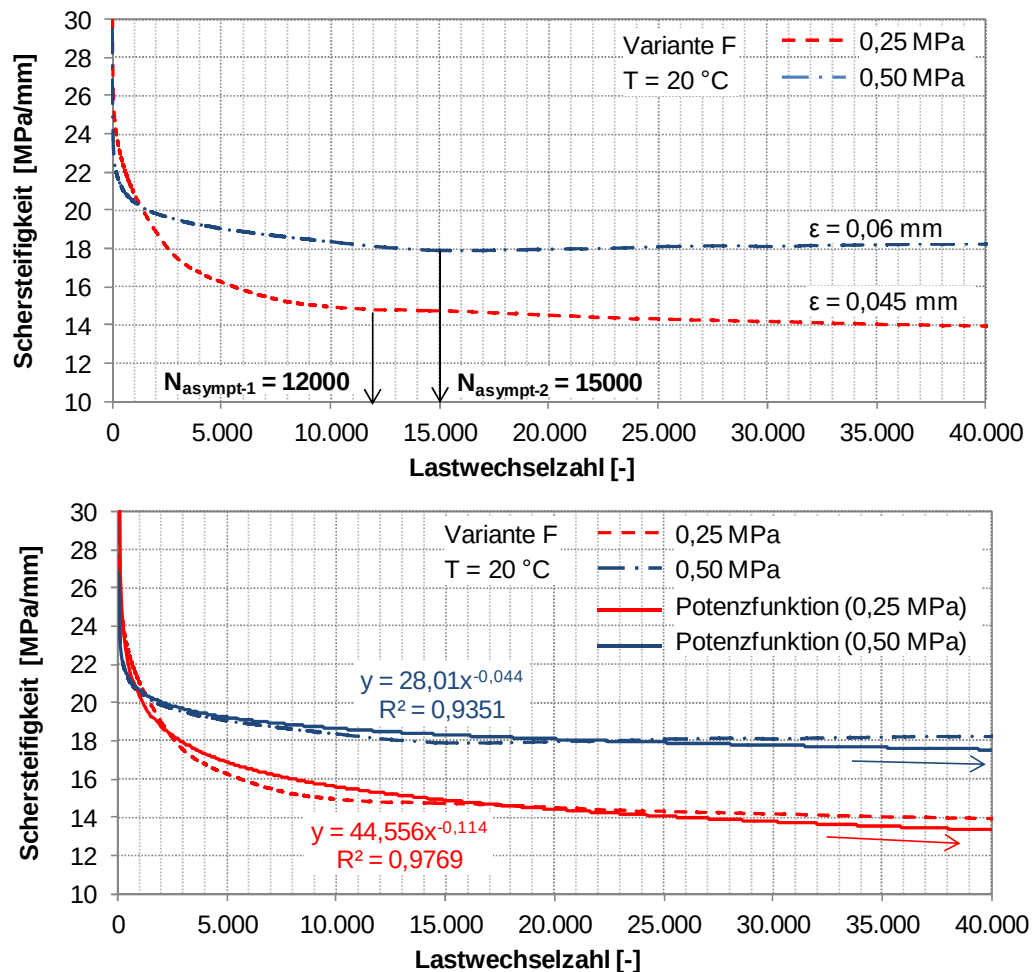
Abbildung 41. Verbundvariante F: Verläufe der Schersteifigkeit während des zyklischen Scherversuchs bei 20 °C und 0,25 MPa und 0,50 MPa Normalspannung (oben). Approximation der Steifigkeitsverläufe mittels Potenzfunktion (unten).
