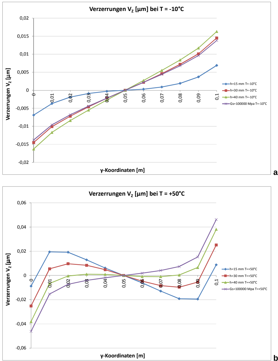
Abbildung 5.12: Verzerrungen V_z [ \mu\text{m} ] bei G_s = 100\,000 \text{ MPa/mm} bei -10^\circ\text{C} (a) und 50^\circ\text{C} (b)
