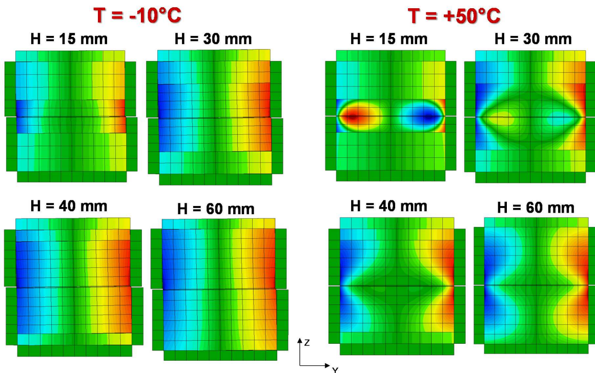
Abbildung 5.13: Verlauf der Verzerrungen V_z bei -10^\circ\text{C} (links) und 50^\circ\text{C} (rechts) für alle vier Schichtdicken
