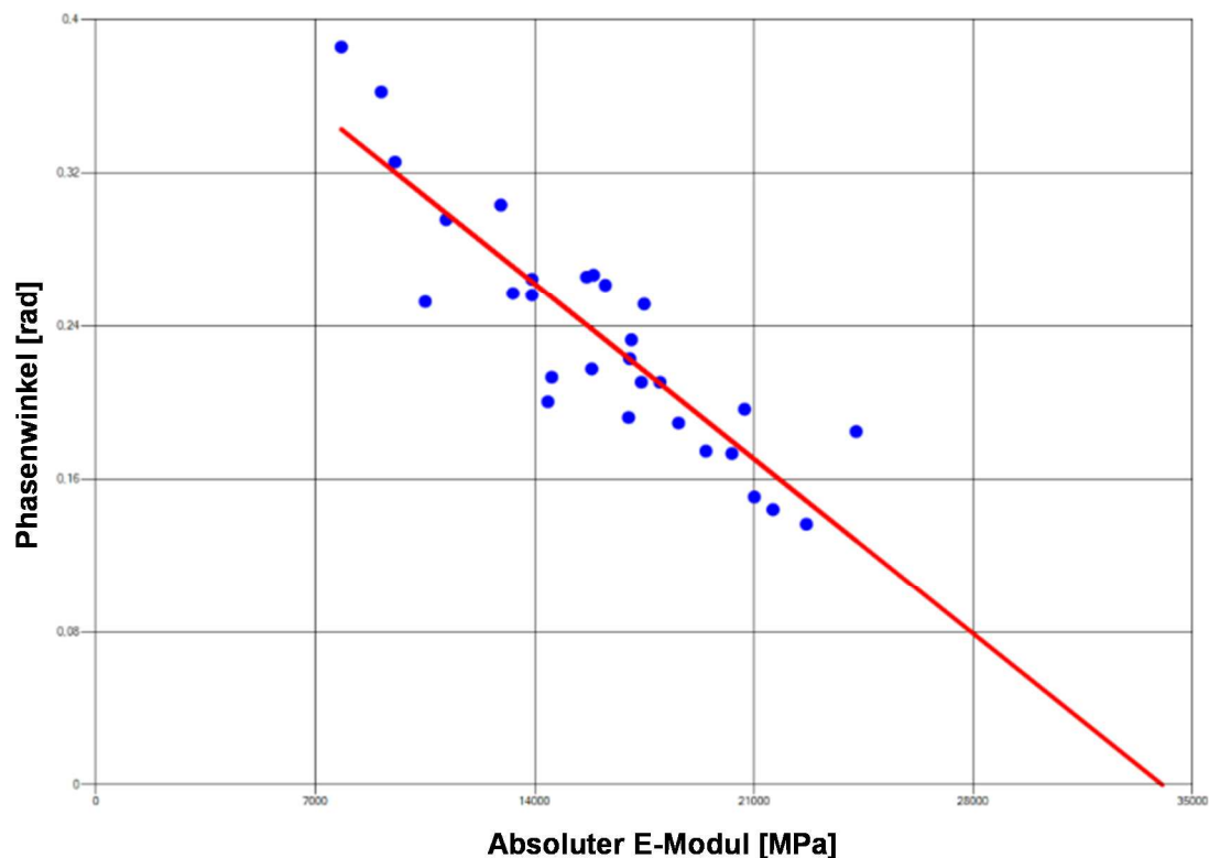
Abbildung 5.69: Abhängigkeit des Phasenwinkels \delta vom absoluten E-Modul zur Abschätzung des Grenzmoduls |E|_{\max} für SMA 11 S
