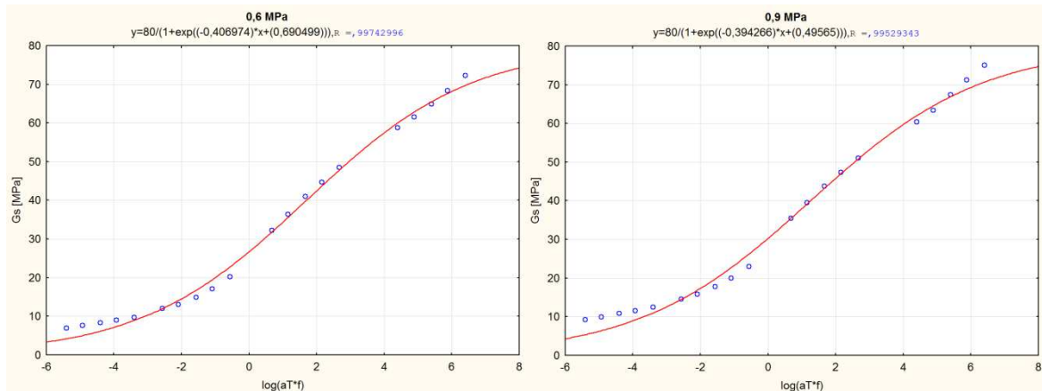
Abbildung 4.6: Funktionale Abhängigkeit zwischen experimentell bestimmter Schersteifigkeit und Temperatur-Frequenz-Äquivalenz-Parameter zur Bestimmung der Parameter a und b (C60BP1-S, 400 g/m 2 )
