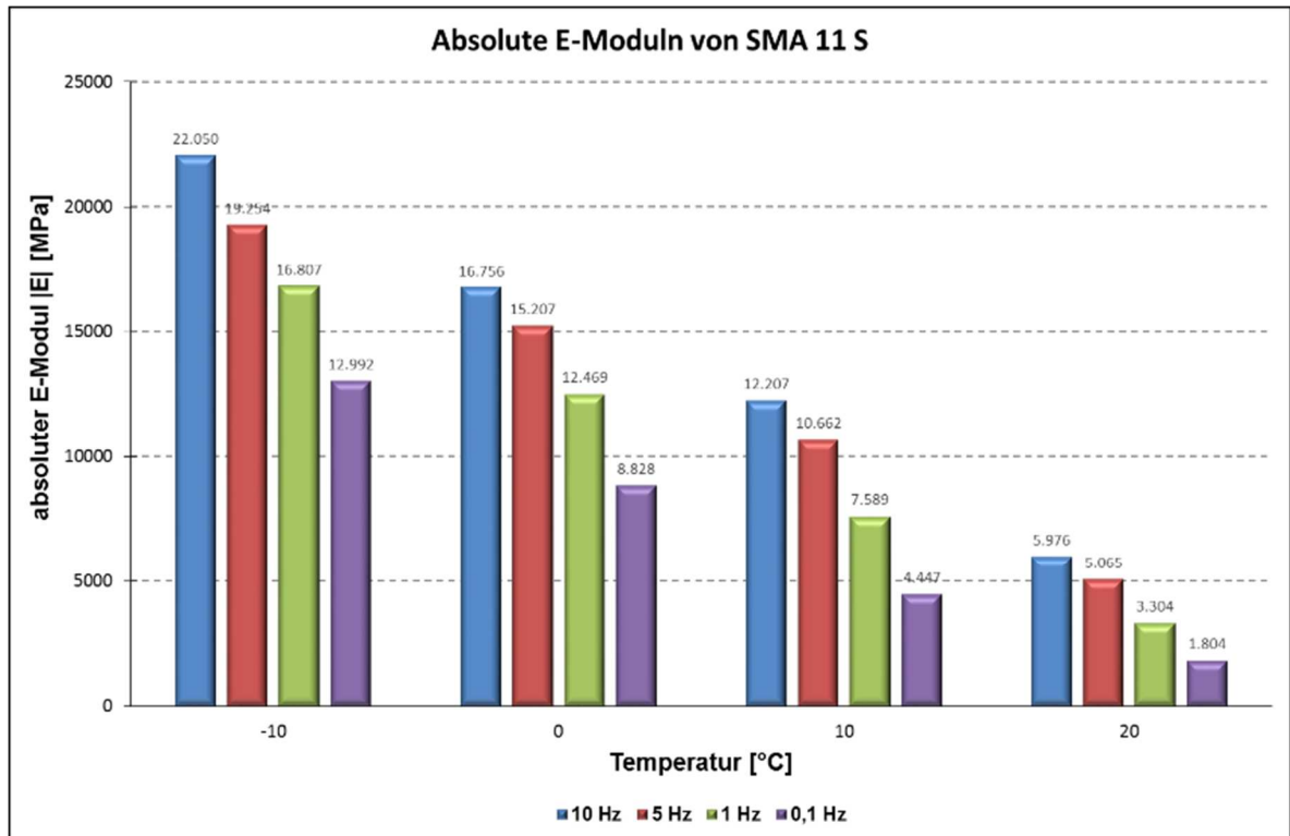
Abbildung 5.74: Vergleich der absoluten E-Moduln des Asphaltdeckschichtmaterials SMA 11 S bei vier Belastungsfrequenzen und vier Temperaturen
