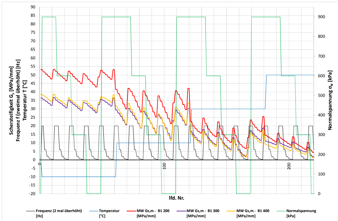
Abbildung 5.39: Mittelwerte der versuchstechnisch ermittelten Schersteifigkeiten bei Anwendung der Bitumenemulsion C60 BP1-S von dem Hersteller Nr. 1 auf fein geschliffenen Oberflächen
