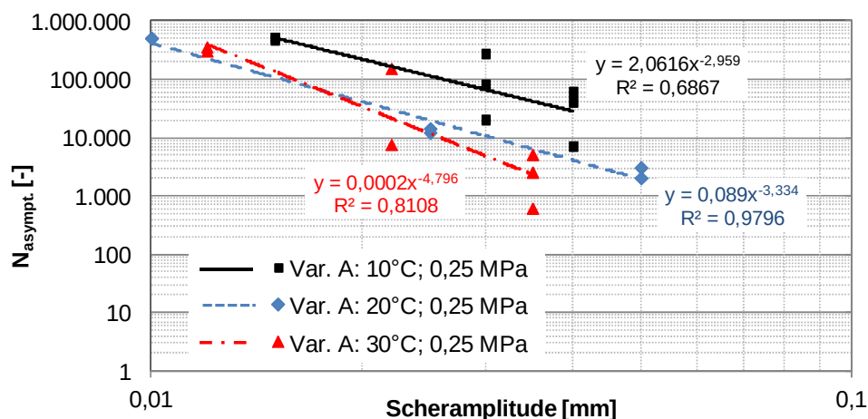
Abbildung 59. Wöhler-Linien für Verbundvariante A bei 0,25 MPa Normalspannung und bei den Prüftemperaturen 30 °C, 20 °C und 10 °C.
