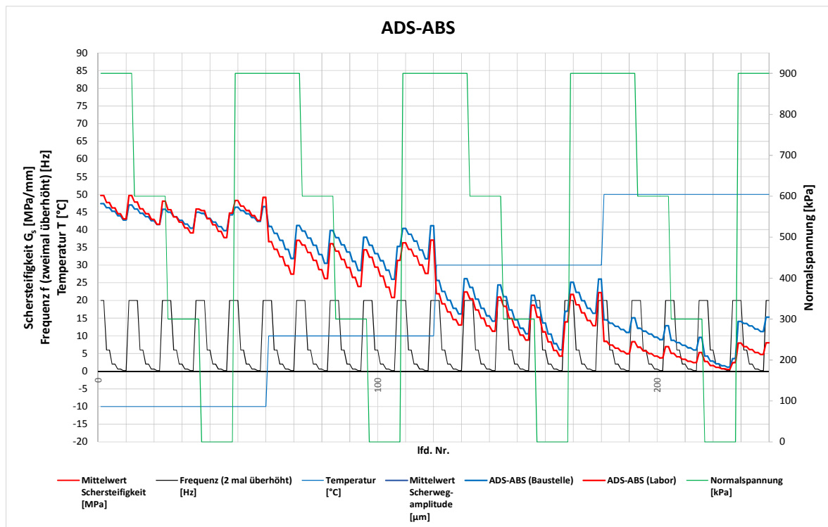
Abbildung 5.37: Vergleich zwischen den versuchstechnisch ermittelten Schersteifigkeiten für die Kombination ADS-ABS zwischen Baustelle und Laborium
