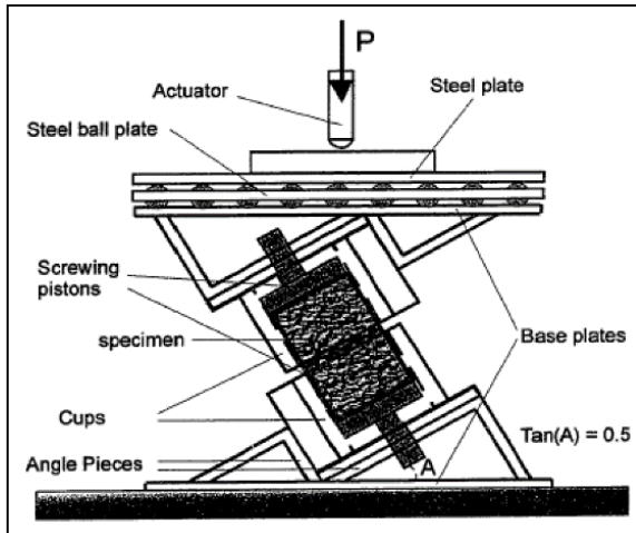
Abbildung 2.17: Schematische Darstellung der SFT Prüfvorrichtung nach Romanoschi (1999)
