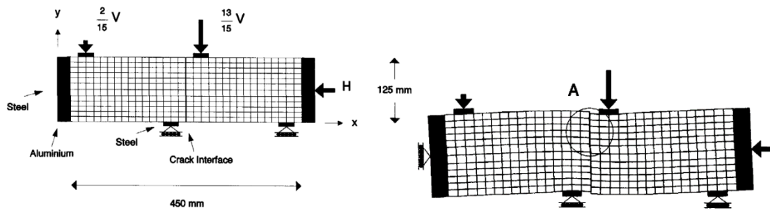
Abbildung 2.22: FEM-Model des Versuches und verformter Probekörper (überhöht) nach de Bondt (1999)
