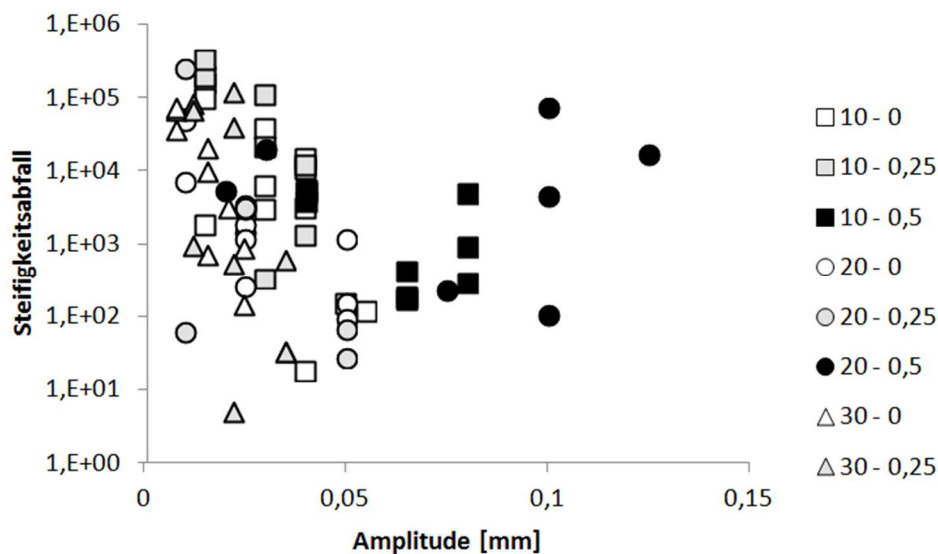
Abbildung 69. Verbundvariante A: Alle Werte des Schersteifigkeitsabfalls a_3 in Abhängigkeit von der Scheramplitude.
