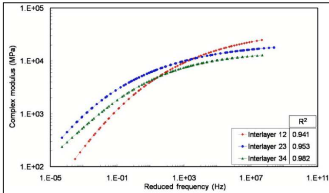
Abbildung 2.30: Vergleich zwischen den Masterkurven von den drei Trennschichten nach Kim u.a. (2011)
