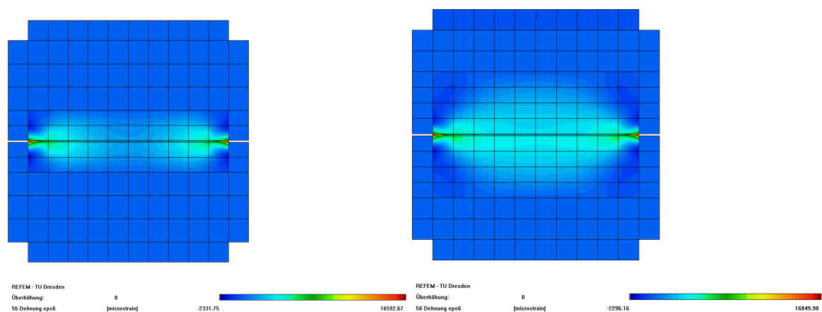
Abbildung 5.15: Dehnungen \epsilon_{ZY} bei G_S = 100\,000 MPa/mm, T = -10^\circ\text{C} bei einer Schichtdicke von 15 mm (links) und 30 mm (rechts)
