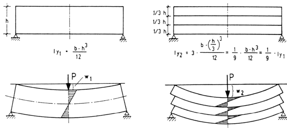
Abbildung 2. Darstellung des Spannungsverlaufes unterschiedlicher Verbundsysteme: (links) voller Verbund zwischen den Schichten und (rechts) Auflösung des Verbundes an den Schichtgrenzen (Weber, 1991).
