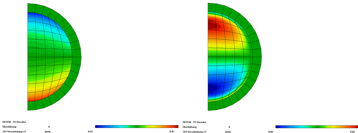
Abbildung 5.14: Verlauf der Verzerrungen bei einer Schichtdicke von 15 mm, GS = 100\,000 MPa/mm, sw = 0,03 mm bei -10^\circ\text{C} (links) und 50^\circ\text{C} (rechts)
