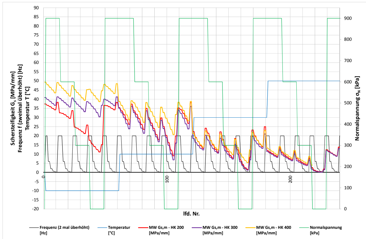
Abbildung 5.43: Mittelwerte der versuchstechnisch ermittelten Schersteifigkeiten bei Anwendung der Bitumenemulsion C40BF1-S (Haftkleber) auf fein geschliffenen Oberflächen
