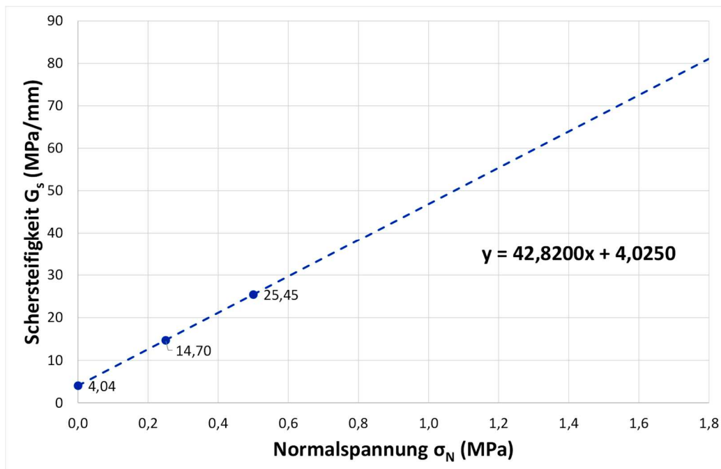
Abbildung 5.63: Zusammenhang zwischen verbleibender Schersteifigkeit bei vollständig ermüdetem Schichtenverbund und Normalspannung
