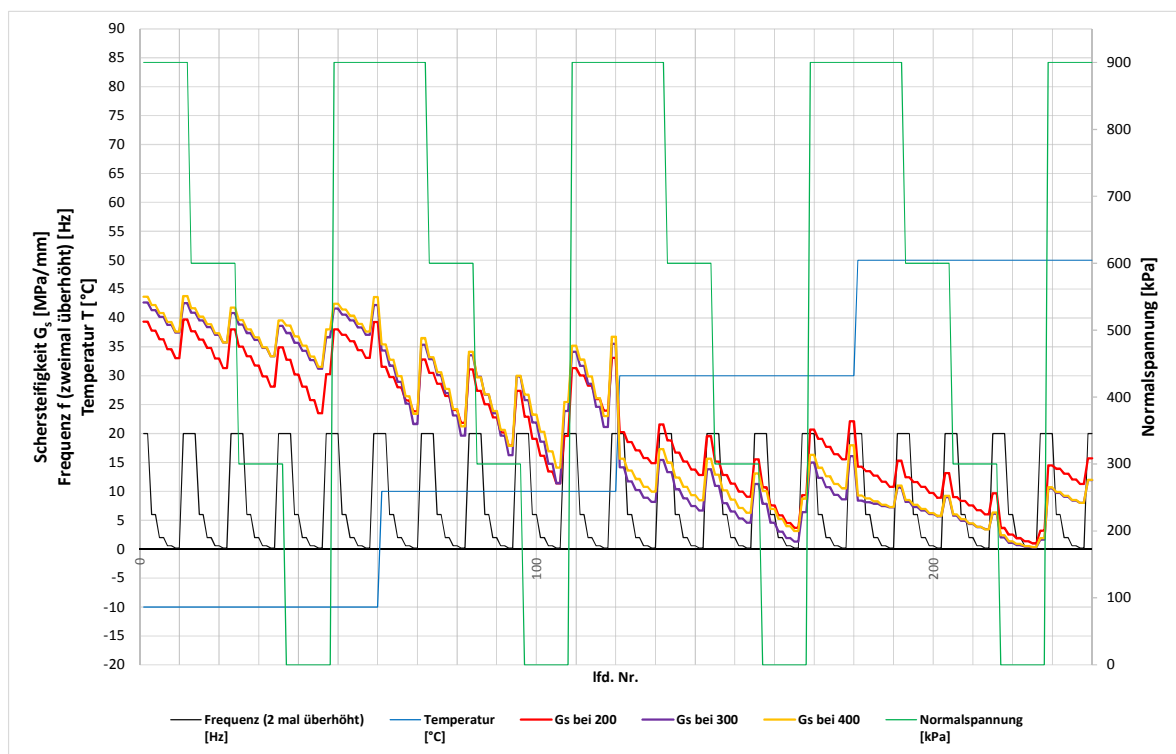
Abbildung 5.26: Mittelwerte der versuchstechnisch ermittelten Schersteifigkeiten des Schichtenverbundes zwischen geschliffenen Oberflächen bei 200 g/m 2 , 300 g/m 2 und 400 g/m 2
