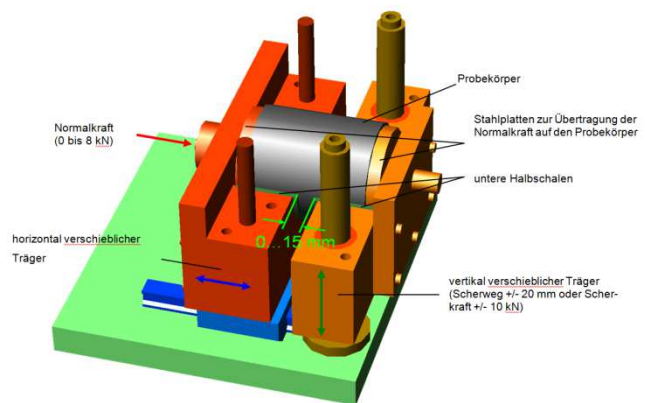
Abbildung 2.23: Prüfvorrichtung nach Wellner / Ascher (2007)
