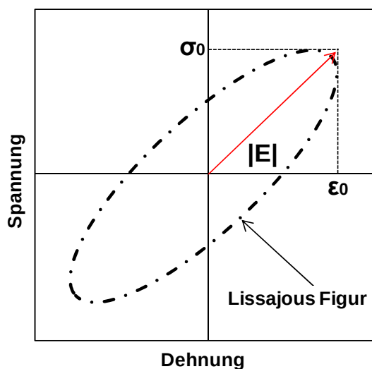
Abbildung 7. Darstellung von einem Belastungszyklus in Spannungs-Dehnungsdiagramm bei einem visko-elastischen Material wie Asphalt.
