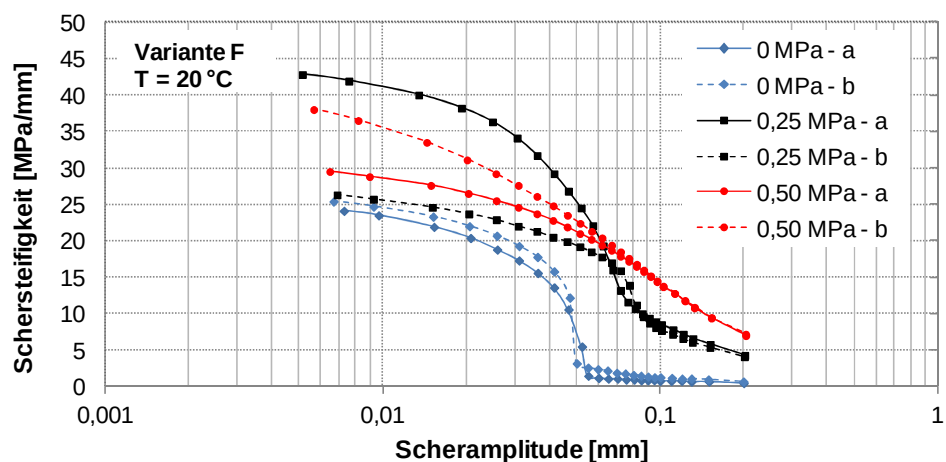
Abbildung 32. Verbundvariante F: Verläufe der Schersteifigkeiten bei drei Normalspannungen (0 MPa, 0,25 MPa und 0,50 MPa) während des Amplitudensweeps bei 20 °C.
