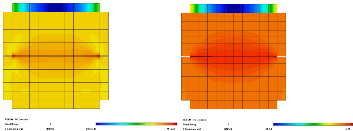
Abbildung 5.21: Scherspannungen \tau_{zy} bei vollem (links) und bei fehlendem Verbund (rechts)
