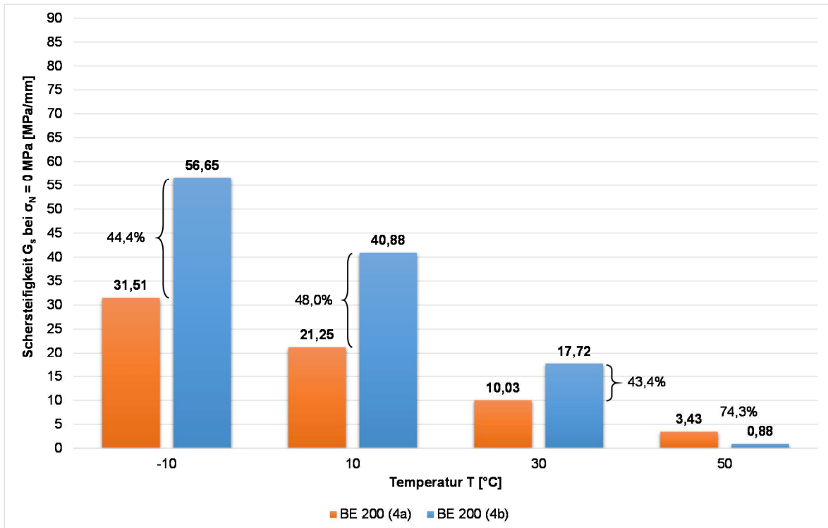
Abbildung 5.32: Vergleich der optimalen Schersteifigkeiten bei reiner Verklebung und bei dem kombinierten Effekt aus Verklebung, Verzahnung und Reibung (200 g/m 2 C60 BP1-S, \sigma_N = 0 MPa und f = 10 Hz)
