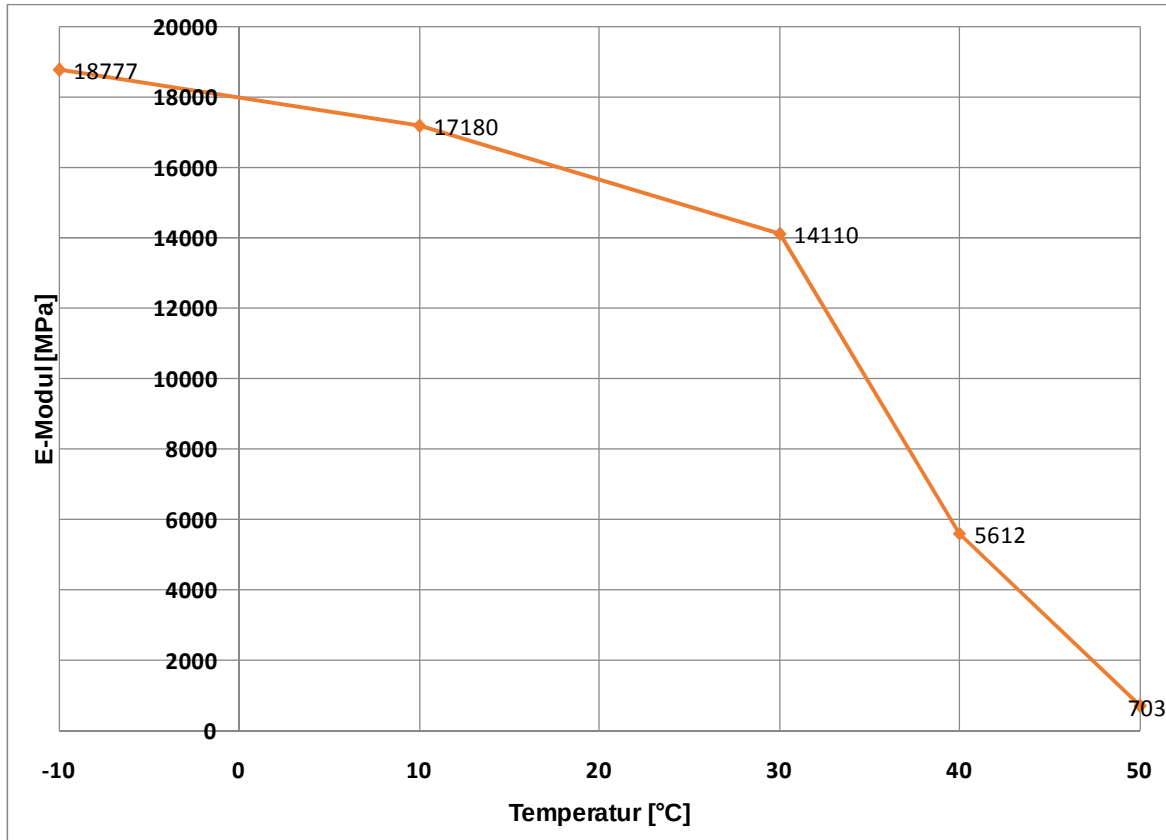
Abbildung 3.22: Steifigkeitsmodul des in den Versuchen verwendeten Epoxidharzklebers Sikadur®-30 in Abhängigkeit von der Temperatur
