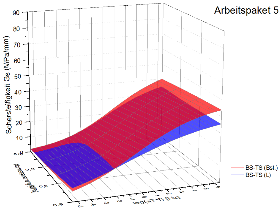
Abbildung 5.36: Vergleich zwischen den Flächenfunktionen der berechneten Schersteifigkeiten für die Kombination ABS-ATS zwischen Baustelle und Laborium
