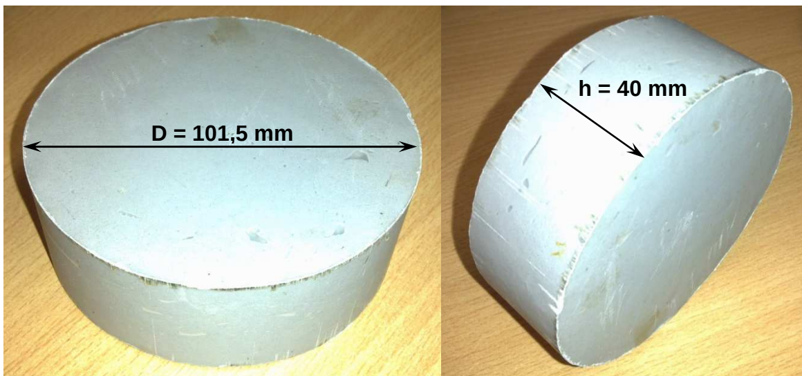
Abbildung 3.21: Fertiger Probekörper aus 2-komponenten-Epoxidharzkleber Sikadur®-30
