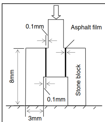
Abbildung 2.34: Darstellung der Probekonfiguration nach Mo u.a. (2006)
