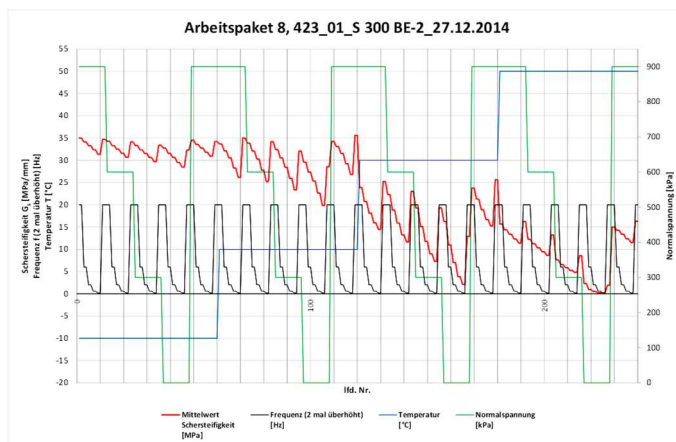
Abbildung 4.2: Beispiele einer konstant bleibenden Schersteifigkeit bei -10^{\circ}\text{C} und 10^{\circ}\text{C}
