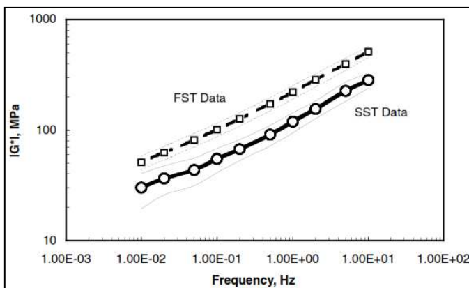
Abbildung 2.13: Komplexer Schermodul in Abhängigkeit von der Prüffrequenz ermittelt mit SST und FST bei 40°C nach Harrigan (2002)
