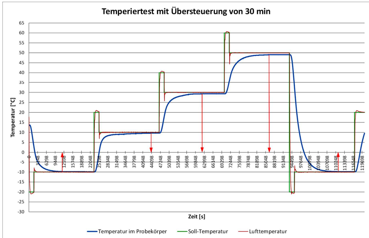
Abbildung 3.11: Verlauf der Temperatur im Asphaltprobekörper, der Soll- und der Lufttemperatur beim Versuch mit 30-minütigen Temperaturübersteuerung um 10^{\circ}\text{C} (Temperiertest Nr. 2)
