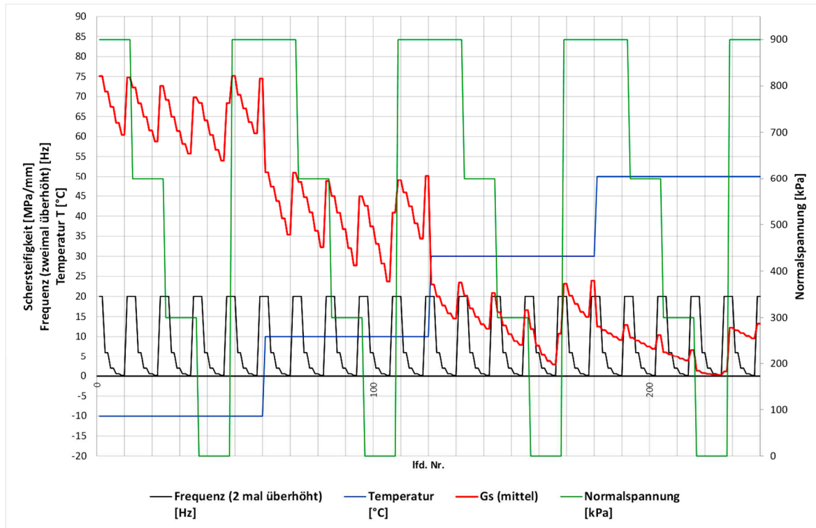
Abbildung 4.1: Verlauf der Schersteifigkeit in Abhängigkeit von der Prüftemperatur, der Belastungsfrequenz und der Normalspannung
