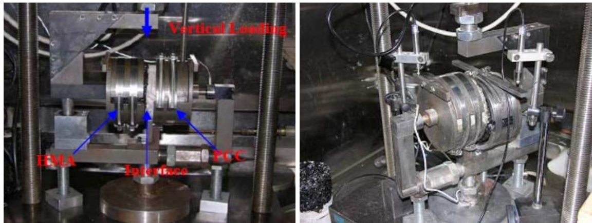
Abbildung 2.15: „Direct Shear Test“ Prüfgerät nach Al-Qadi u.a. (2008)
