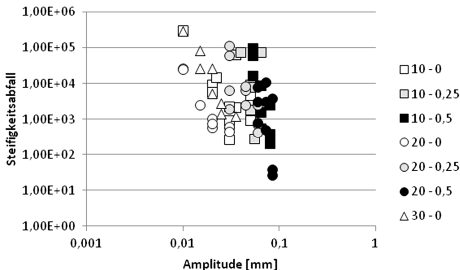
Abbildung 90. Verbundvariante F: Alle Werte des Schersteifigkeitsabfalls a_3 in Abhängigkeit von der Scheramplitude.
