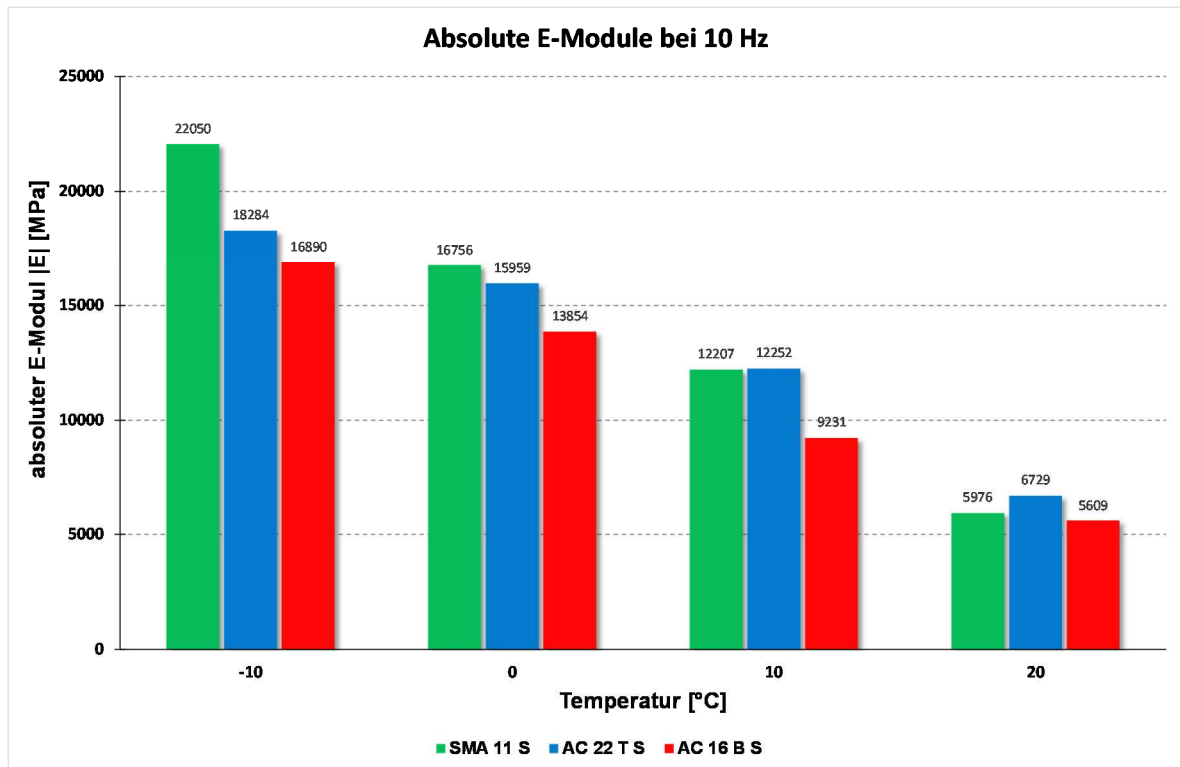
Abbildung 5.73: Vergleich der absoluten E-Moduln der drei Asphaltmaterialien bei einer Belastungsfrequenz von 10 Hz und vier Temperaturen
