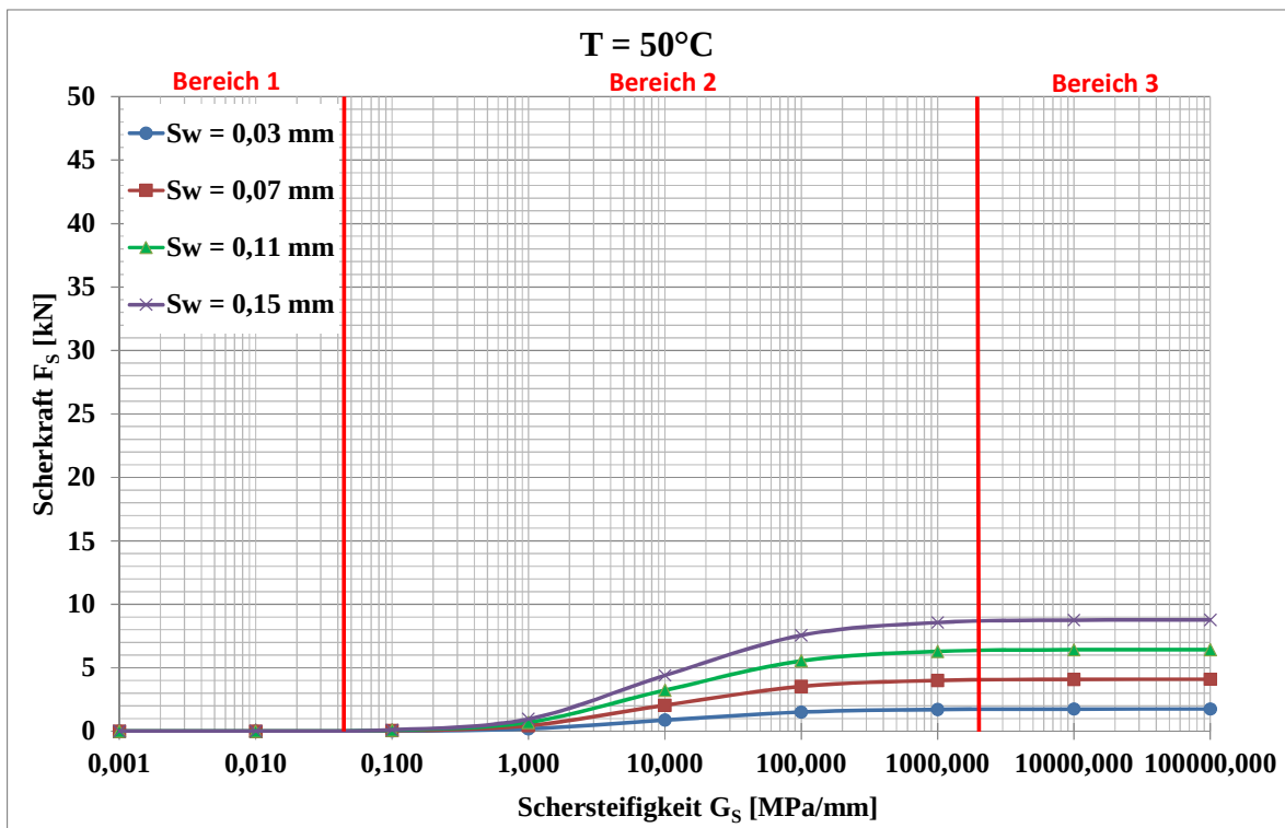
Abbildung 4.11: Funktionaler Zusammenhang zwischen Scherkraft und Schersteifigkeit für alle vier untersuchten maximalen Scherwege bei 50°C
