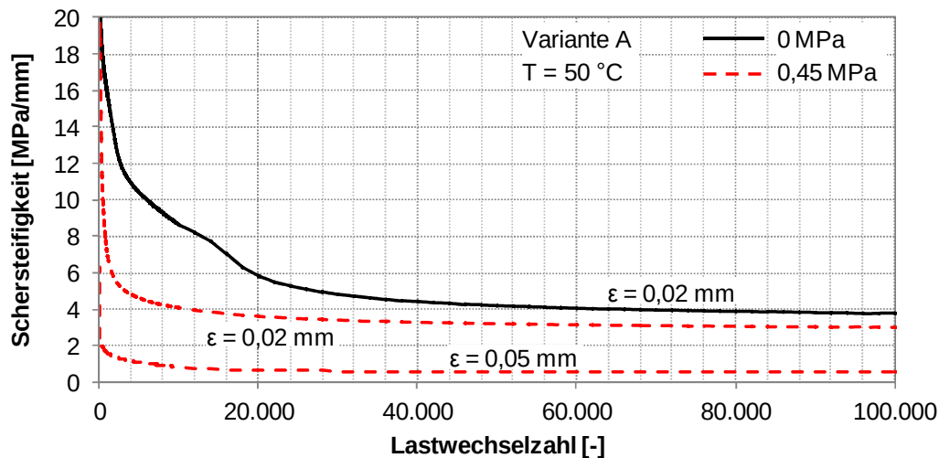
Abbildung 53. Verbundvariante A: Verläufe der Schersteifigkeit während der Scherermüdungsprüfung bei 50 °C, bei zwei Normalspannungen (0 MPa und 0,45 MPa) und bei zwei Scheramplituden (0,02 mm und 0,05 mm).
