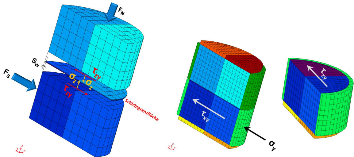
Abbildung 3.29: An der Schichtgrenzfläche wirkende Spannungen
