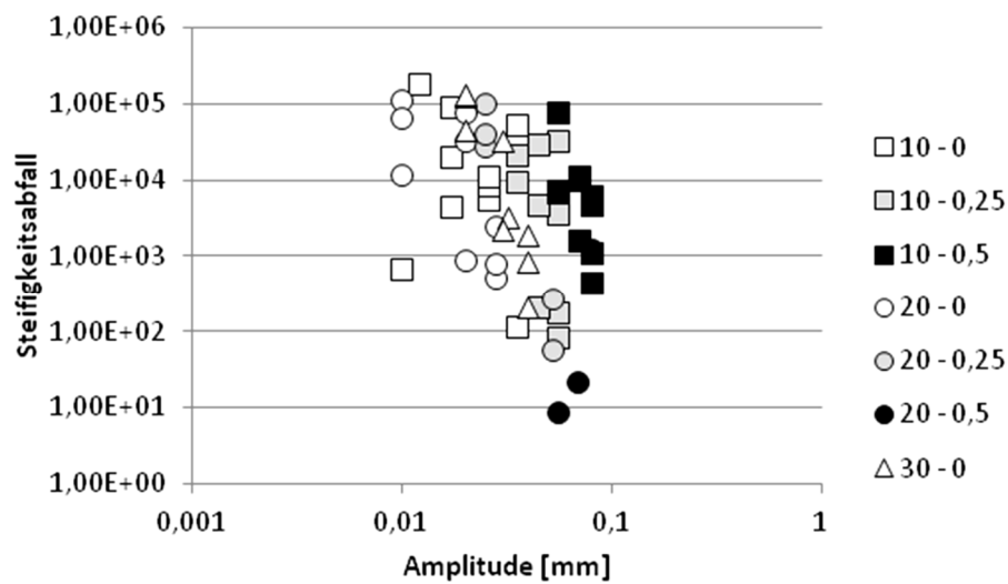
Abbildung 88. Verbundvariante D: Alle Werte des Schersteifigkeitsabfalls a_3 in Abhängigkeit von der Scheramplitude.
