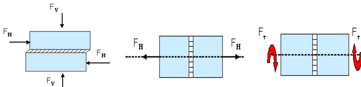
Abbildung 10. Meist verwendete Belastungsvorgänge zur Beurteilung der Qualität des Schichtenverbundes; direktes Abscheren (links), direktes Ziehen (mittig) und Kombination aus Abscheren und Torsion (rechts) (Al-Qadi et al., 2008).
