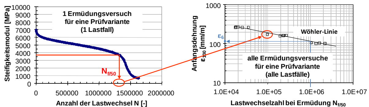
Abbildung 5. Beispiel für eine Ermüdungsfunktion (Wöhler-Linie) als Materialgesetz für das Ermüdungsversagen.
