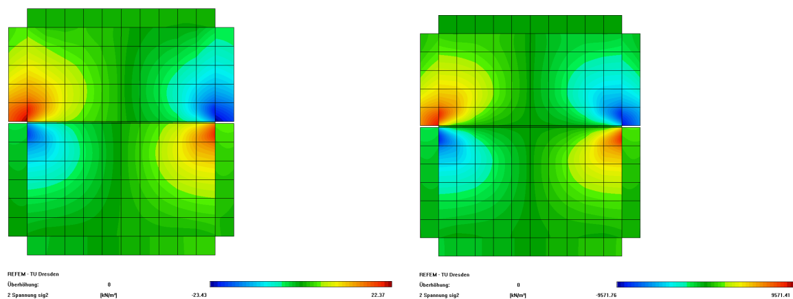
Abbildung 4.13: Verteilung der Spannungen \sigma_y bei T = -10\text{ }^{\circ}\text{C} , s_w = 0,11\text{ mm} , G_s = 100\text{ MPa/mm} (links) und 100000\text{ MPa/mm} (rechts)
