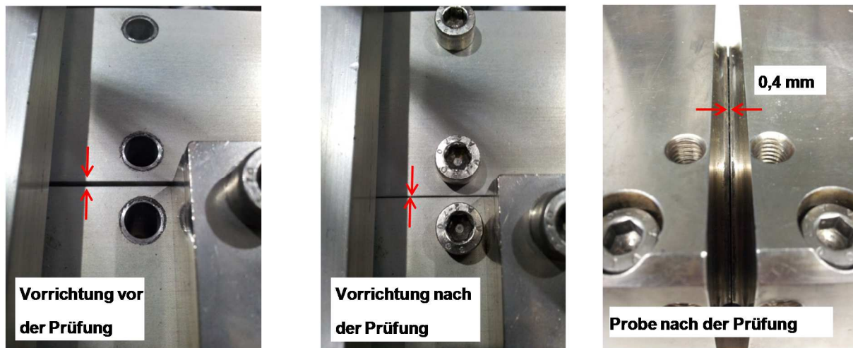
Abbildung 50. Verbundvariante D: Scherbereich der Prüfvorrichtung vor (links) und nach (Mitte) der Scherermüdungsprüfung bei 20 °C, 0,50 MPa Normalspannung und 0,08 mm Scheramplitude mit der Spaltbreite des geprüften Probekörpers (rechts).
