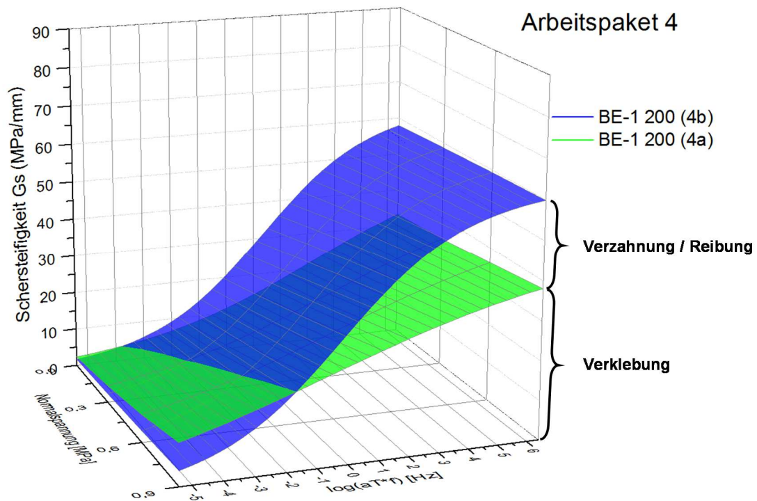
Abbildung 5.31: Vergleich der zwei optimalen Bitumenemulsionsmengen von 200 g/m 2 bei reiner Verklebung zwischen den Asphaltschichten und bei normal hergestelltem Schichtenverbund
