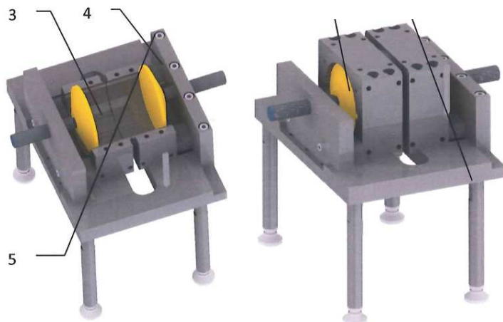
Abbildung 3.4: Modell der Klebevorrichtung (Quelle: Wille)
