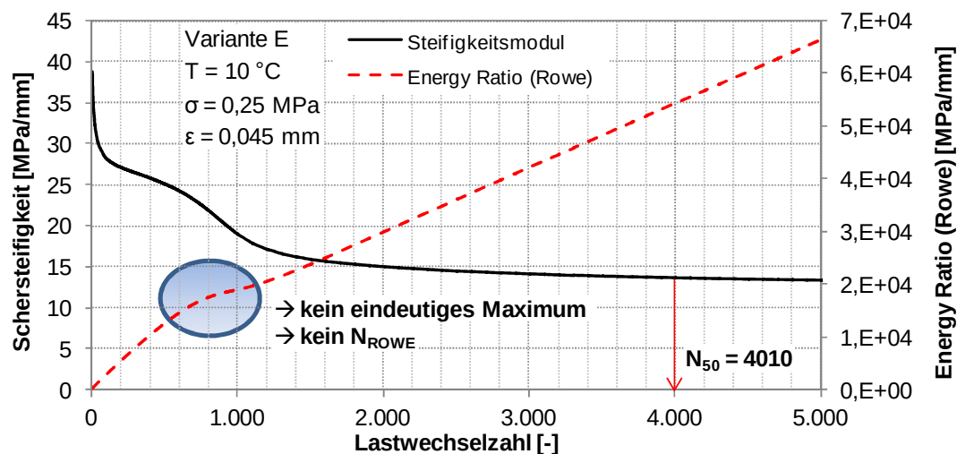
Abbildung 40. Verbundvariante E: Verläufe der Schersteifigkeit und dissipierten Energie nach Rowe während des zyklischen Scherversuchs bei 10 °C, 0,25 MPa Normalspannung und 0,045 mm Scherweg.
