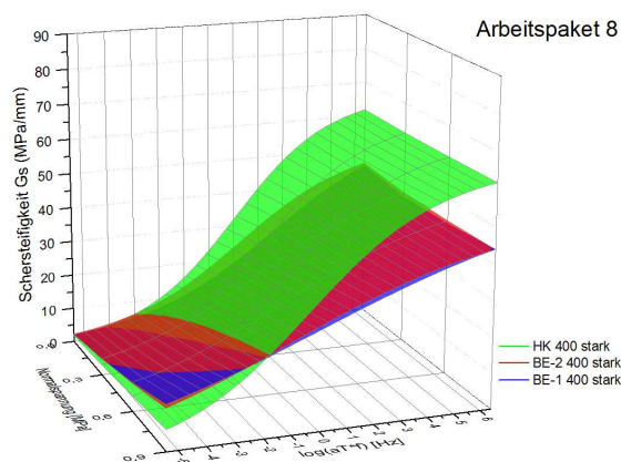
Abbildung 5.55: Flächenfunktionen der berechneten Schersteifigkeiten bei stark verschmutzter Oberfläche und 400 \text{ g/m}^2 Bitumenemulsionsmenge
