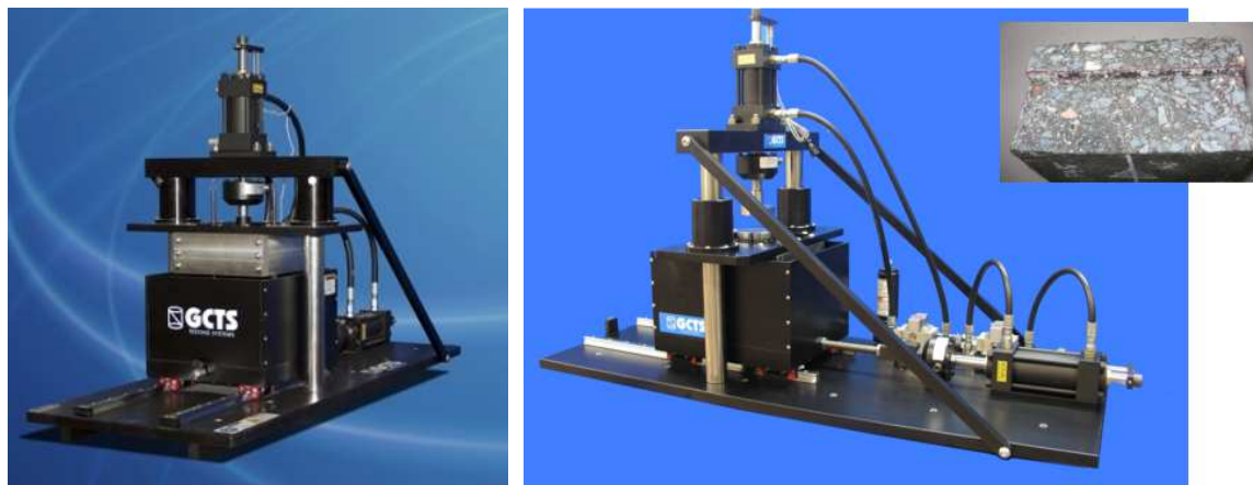
Abbildung 2.16: GCTS-Prüfvorrichtung SDS-150 (Arizona, USA)
