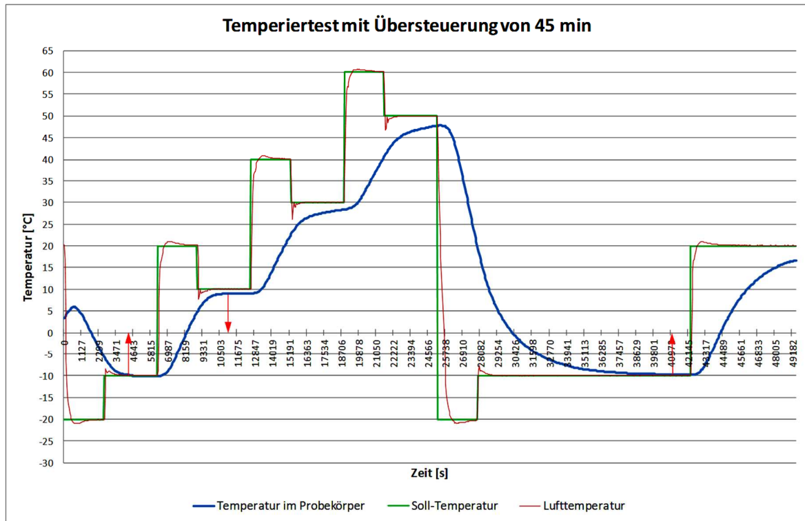
Abbildung 3.13: Verlauf der Temperatur im Asphaltprobekörper, der Soll- und der Lufttemperatur beim Versuch mit 45-minütigen Temperaturübersteuerung um 10^{\circ}\text{C} (Temperiertest Nr. 4)
