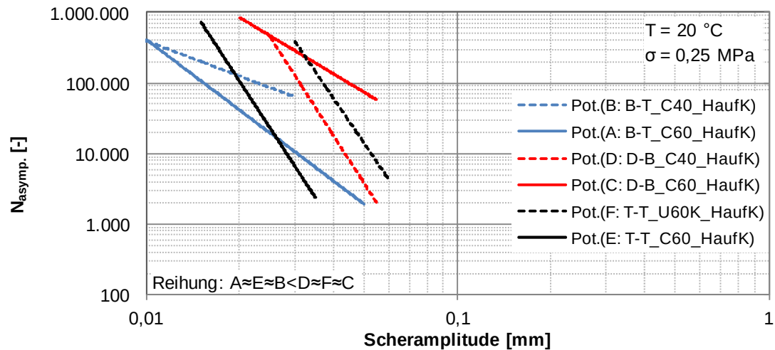
Abbildung 98. Wöhler-Linien für die Verbundvarianten A bis F bei einer Prüftemperatur von 20 °C und bei einer Normalspannung von 0,25 MPa mit einer Reihung der Verbundvarianten bezüglich der Scherermüdungsbeständigkeit.
