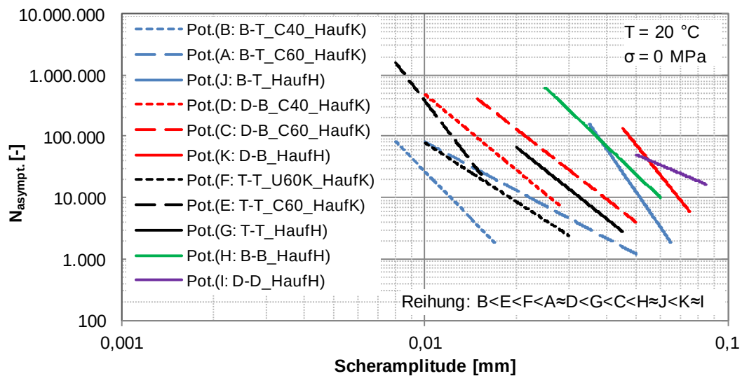
Abbildung 95. Wöhler-Linien für die Verbundvarianten A bis K bei einer Prüftemperatur von 20 °C und ohne Normalspannung mit einer Reihung der Verbundvarianten bezüglich der Scherermüdungsbeständigkeit.
