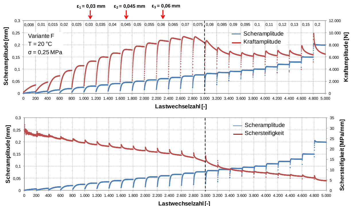
Abbildung 29. Verbundvariante F: Verläufe der Kraft (oben) und der Schersteifigkeit (unten) während des Amplitudensweeps bei 20 °C und 0,25 MPa Normalspannung.
