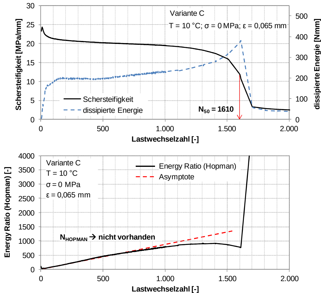
Abbildung 39. Verbundvariante C: Verläufe der Schersteifigkeit, dissipierten Energie (oben) und Energierate nach Hopman (unten) während des zyklischen Scherversuchs bei 10 °C, 0 MPa Normalspannung und 0,065 mm Scherweg.
