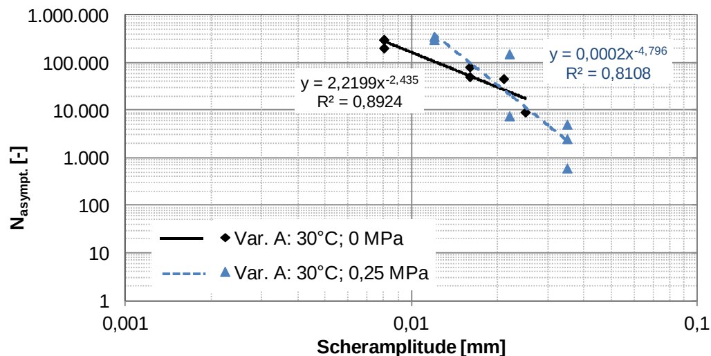
Abbildung 47. Verbundvariante A: Wöhler-Linien bei 30 °C bei den Normalspannungen 0 MPa und 0,25 MPa.
