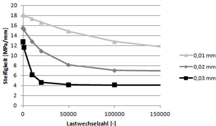
Abbildung 93. Verbundvariante A: Simulation des Schersteifigkeitsverlaufes in Abhängigkeit von der Scheramplitude für \epsilon = 0,01 mm, 0,02 mm und 0,03 mm für eine Prüftemperatur von T = 20^\circ\text{C} und eine Normalspannung von \sigma = 0,0 MPa.
