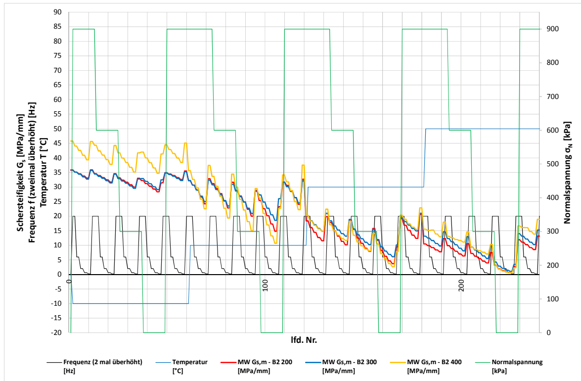
Abbildung 5.41: Mittelwerte der versuchstechnisch ermittelten Schersteifigkeiten bei Anwendung der Bitumenemulsion C60 BP1-S von dem Hersteller Nr. 2 auf fein geschliffenen Oberflächen
