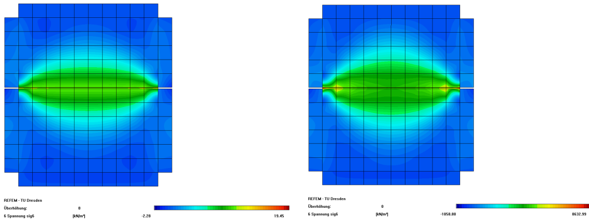
Abbildung 4.14: Verteilung der Scherspannungen \tau_{zy} bei T = -10^\circ\text{C} , s_w = 0,11 \text{ mm} , G_s = 100 \text{ MPa/mm} (links) und 100000 \text{ MPa/mm} (rechts)
