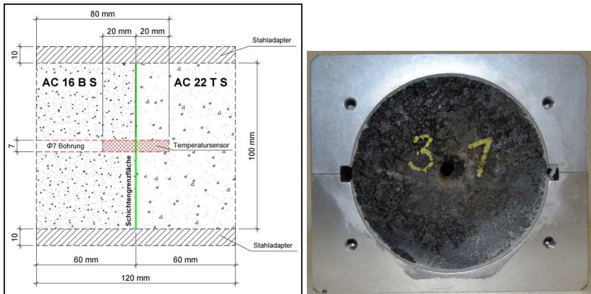
Abbildung 3.8: Schema von dem zweischichtigen Probekörper mit Bohrloch und eingesetzten Temperatursensor (links) und Vorderansicht des Bohrloches (rechts)
