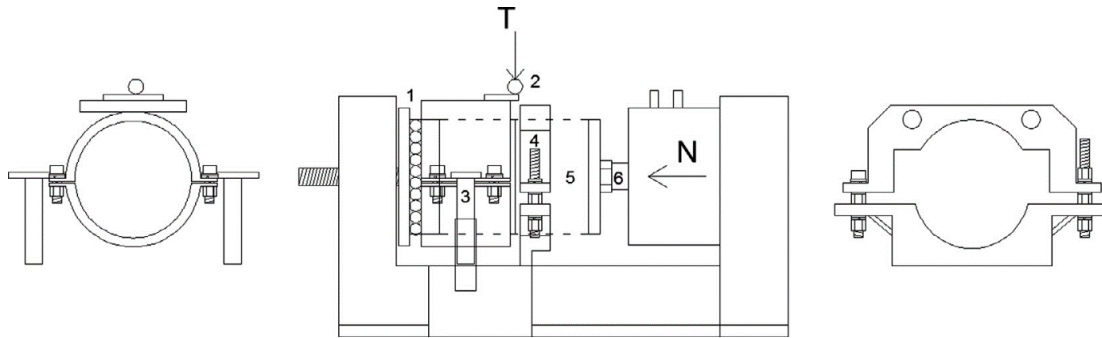
Abbildung 2.36: Prüfvorrichtung Sapienza Dynamic Shear Testing Machine nach D'Andrea u.a. (2014)
