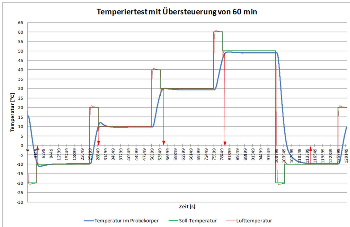
Abbildung 3.12: Verlauf der Temperatur im Asphaltprobekörper, der Soll- und der Lufttemperatur beim Versuch mit 60-minütigen Temperaturübersteuerung um 10^{\circ}\text{C} (Temperiertest Nr. 3)
