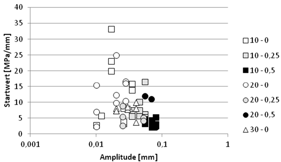
Abbildung 83. Verbundvariante D: Darstellung der Werte des Parameters a_1 über die Scher-amplitude.
