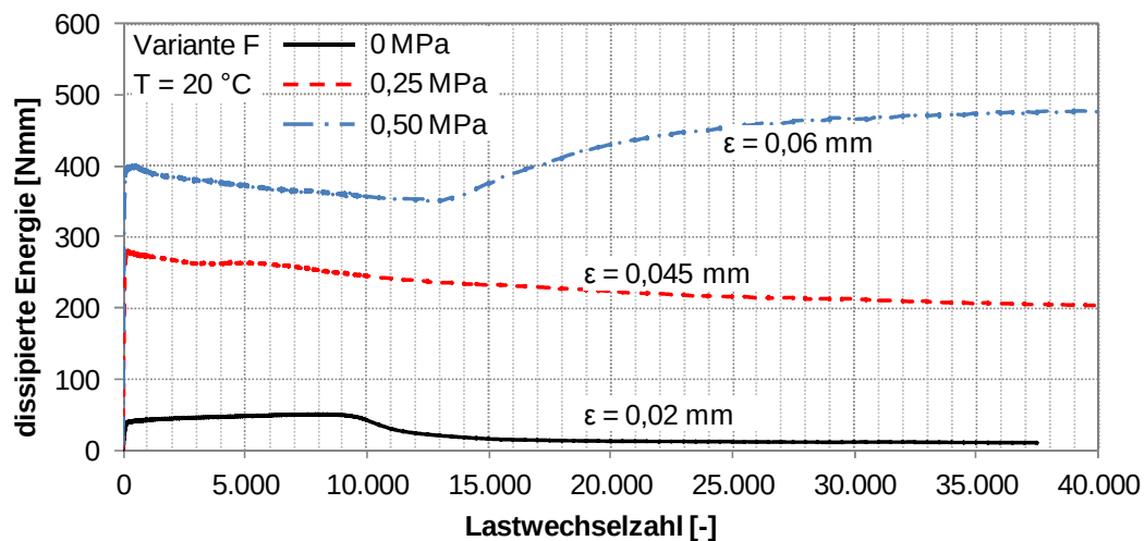
Abbildung 34. Verbundvariante F: Verläufe der Schersteifigkeit (oben), Phasenwinkel (Mitte) und dissipierten Energie pro Lastwechsel (unten) während des zyklischen Scherversuchs bei 20\text{ °C} und 0 MPa, 0,25 MPa und 0,50 MPa Normalspannung.
