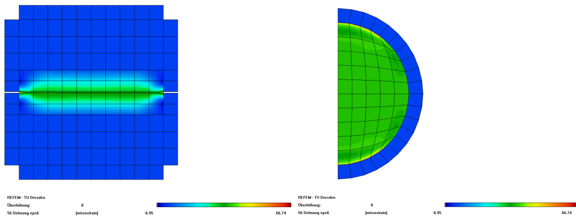
Abbildung 5.18: Dehnungen \epsilon_{zy} bei G_s = 100 MPa/mm, T = 50^\circ\text{C} bei einer Schichtdicke von 15 mm
