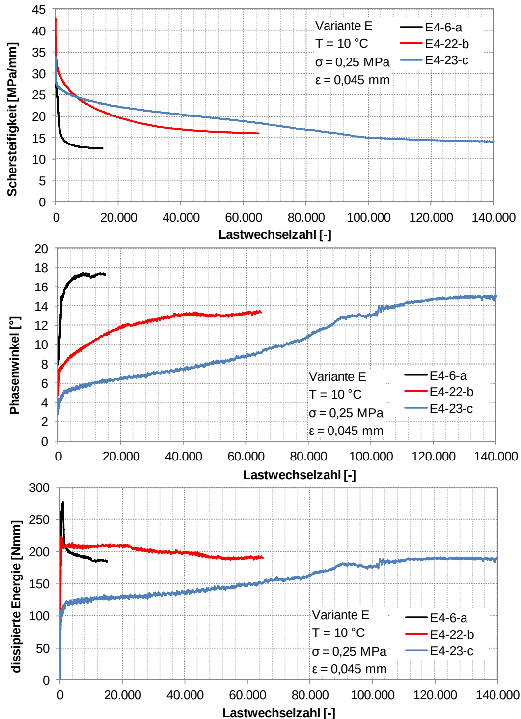
Abbildung 37. Verbundvariante E: Verläufe der Schersteifigkeit (oben), Phasenwinkel (Mitte) und dissipierten Energie pro Lastwechsel (unten) während des zyklischen Scherversuchs bei 10 °C Prüftemperatur, 0,25 MPa Normalspannung und 0,045 mm Scheramplitude.
