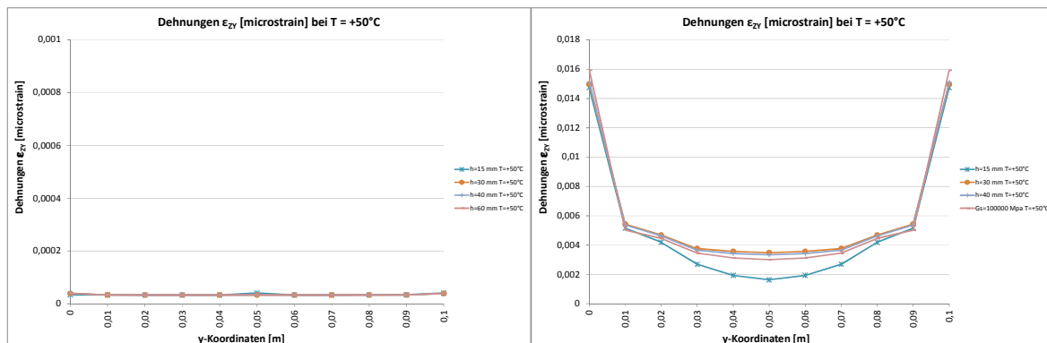
Abbildung 5.20: Dehnungen \varepsilon_{zy} bei fehlendem (links) und vollem (rechts) Verbund, T = 50^\circ\text{C}
