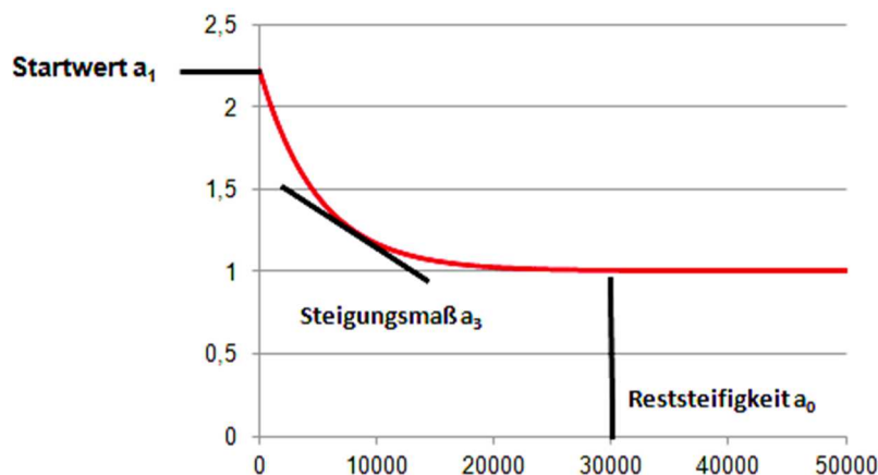
Abbildung 62: Physikalische Interpretation der Parameter a_0 , a_1 und a_3 der Exponentialfunktion zur Simulation des Schersteifigkeitsverlaufes (Gl. 7): verbleibende Restschersteifigkeit infolge Reibung und Verzahnung a_0 , Startwert der Schersteifigkeit a_1 und Schersteifigkeitsabfall a_3 .
