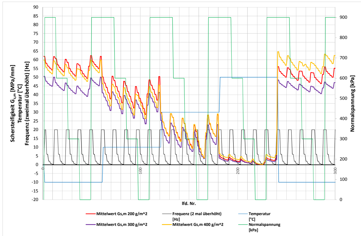
Abbildung 5.30: Mittelwerte der versuchstechnisch ermittelten Schersteifigkeiten des normal hergestellten Schichtenverbundes bei 200 g/m 2 , 300 g/m 2 und 400 g/m 2 bei Wiederholung der tiefsten Temperatur
