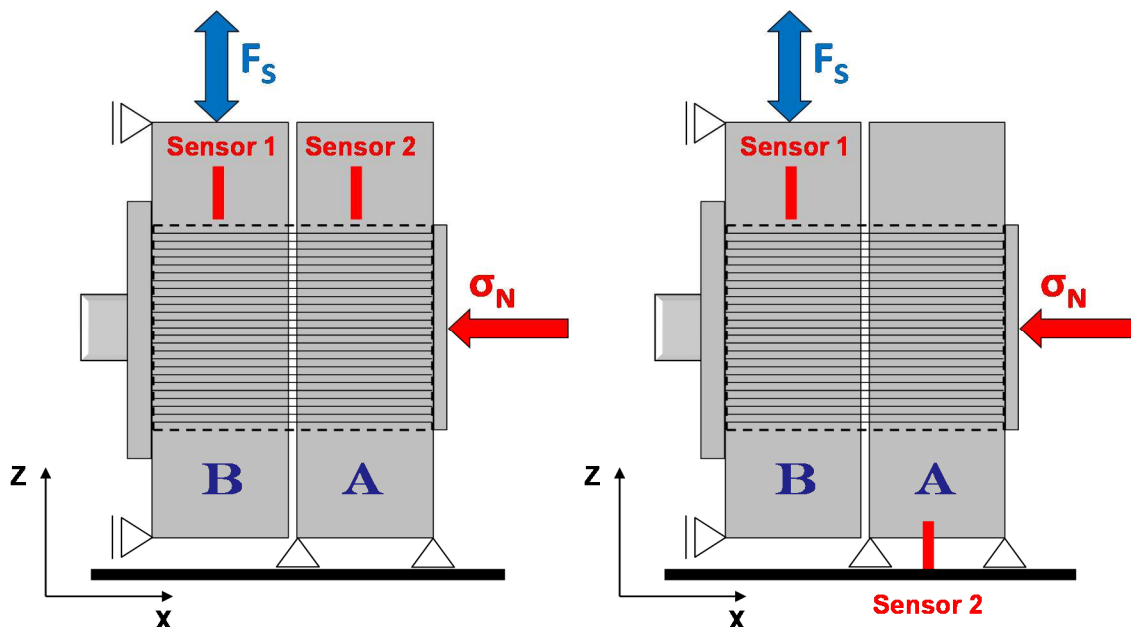
Abbildung 2.1: Anordnung der Wegsensoren zur Überprüfung der Bewegungen der Bauteile der Prüfvorrichtung während der Versuchsdurchführung.
