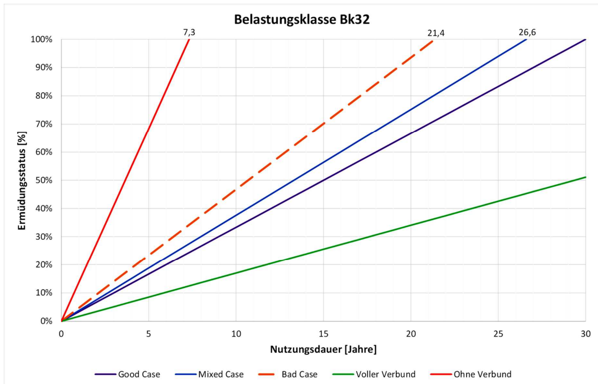
Abbildung 5.66: Verlauf des Ermüdungsstatus bei unterschiedlichen Schichtenverbundfunktionen über die gesamte Nutzungsdauer bei Bk32
