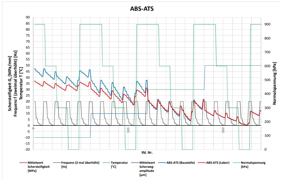
Abbildung 5.38: Vergleich zwischen den versuchstechnisch ermittelten Schersteifigkeiten für die Kombination ABS-ATS zwischen Baustelle und Laborium
