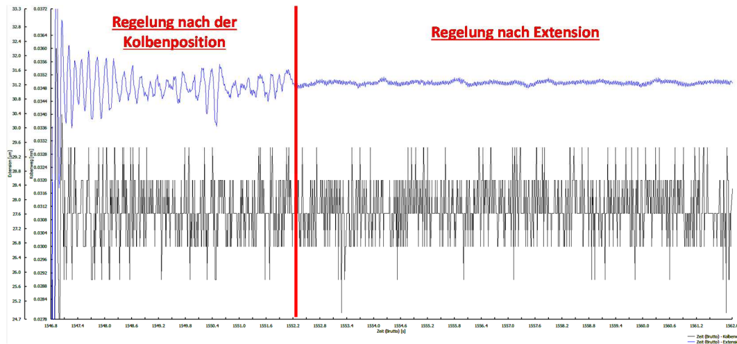
Abbildung 2.1: Verbesserte Präzision der Regelung bei der neu entwickelten Prüfvorrichtung.
