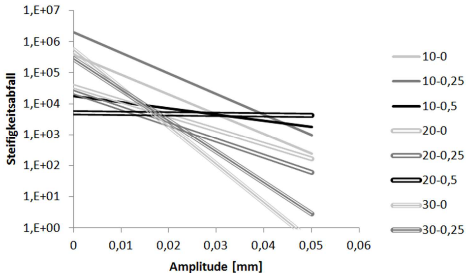
Abbildung 70. Verbundvariante A: Darstellung der ermittelten Regressionen für alle Prüftemperaturen und Normalspannungen.
