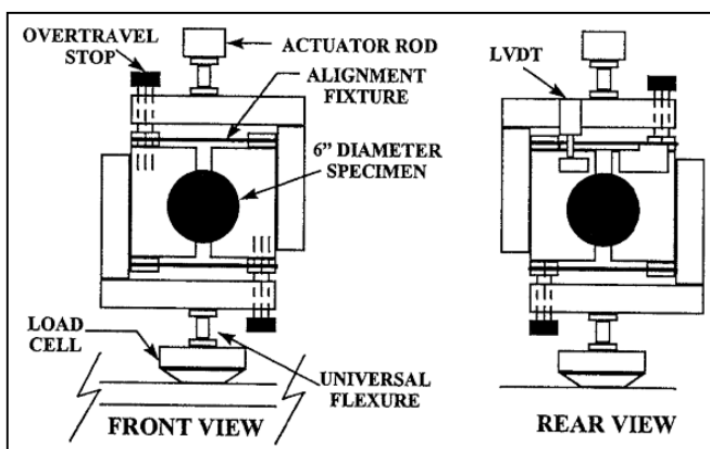
Abbildung 2.11: Schematische Darstellung der FST-Prüfvorrichtung nach Harrigan (2002)
