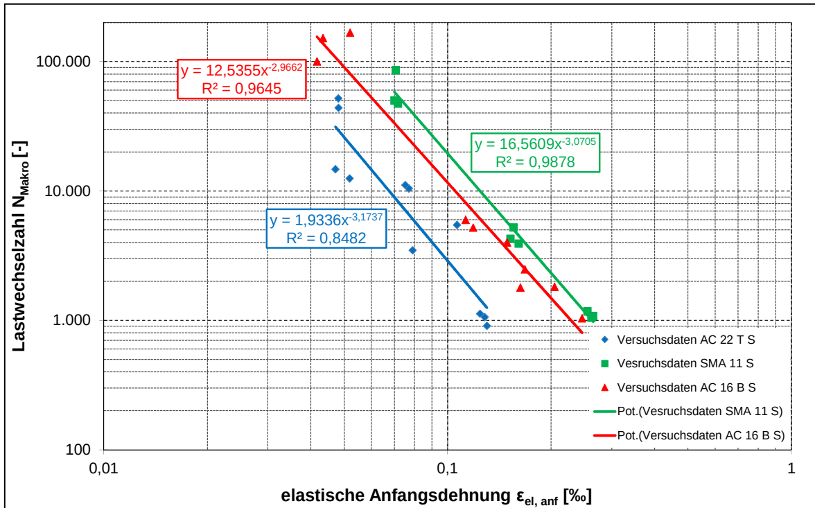
Abbildung 5.76: Ermüdungsfunktionen der Asphaltdeckschicht, Asphaltbinderschicht und Asphalttragschicht bei einer Belastungsfrequenz von 10 Hz und T = 20°C
