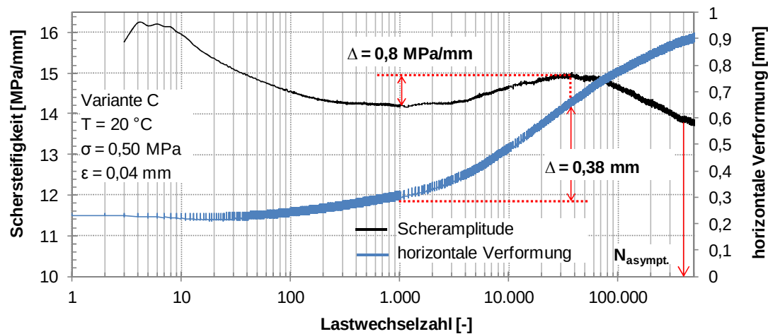
Abbildung 52. Verbundvariante C: Verläufe der Schersteifigkeit und der horizontalen Verformung während der Scherermüdungsprüfung bei 20 °C, 0,50 MPa Normalspannung und 0,04 mm Scheramplitude.
