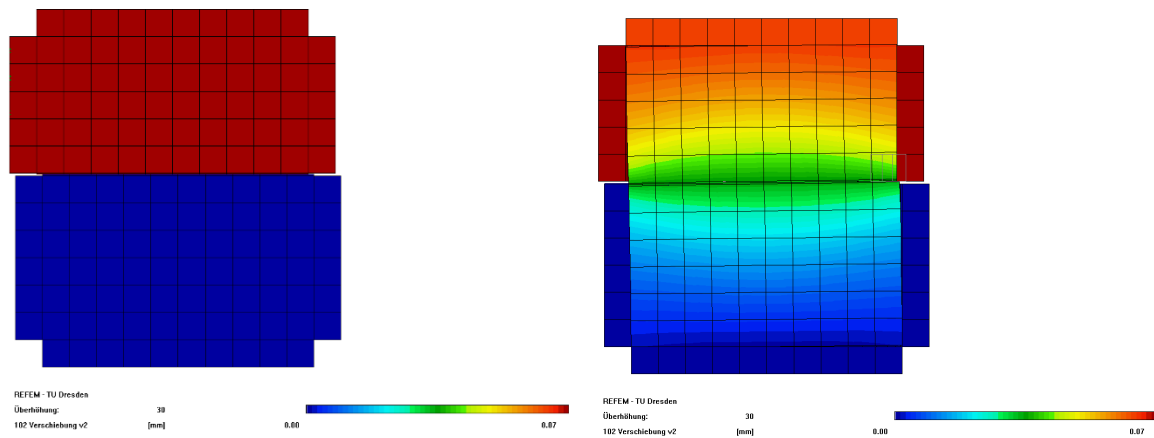
Abbildung 4.12: Horizontale Verschiebungen bei fehlendem (links) und bei vollem Verbund (rechts) bei -10\text{ }^{\circ}\text{C}
