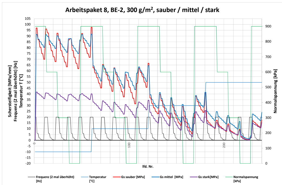
Abbildung 5.57: Vergleich der experimentell ermittelten Schersteifigkeiten bei sauberer, mittel und stark verschmutzter Oberfläche und 300 g/m² Bitumenemulsionsmenge
