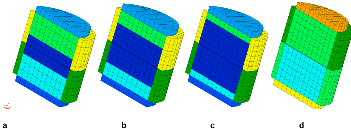
Abbildung 5.10: FE-Modelle der Konfigurationen bei den unterschiedlichen Schichtdicken mit Stahldummies
