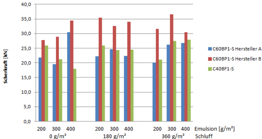
Abbildung 105. Abscherfestigkeiten [kN] ermittelt mit dem statischen Abscherversuch nach den TP Asphalt-StB Teil 80 für die Schicht-Kombination Binderschicht auf Tragschicht (B-T) bei Variation der auf der Unterlage aufgetragenen Schluffmenge (0, 180 oder 360 g/m 2 ) und der Menge an Bitumenemulsion (200, 300 oder 400 g/m 2 ).
