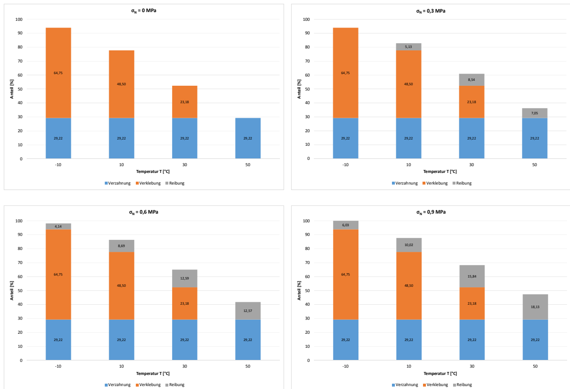
Abbildung 5.46: Anteile von Verklebung (orange), Verzahnung (blau) und Reibung (grau) für Verbundvariante (4) bei den vier Normalspannungen
