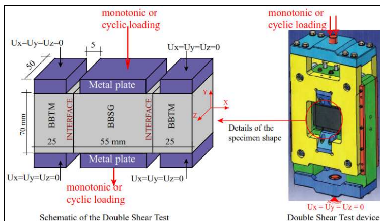
Abbildung 2.6: Probekörper und Prüfvorrichtung DST nach Diakhaté u.a. 2008
