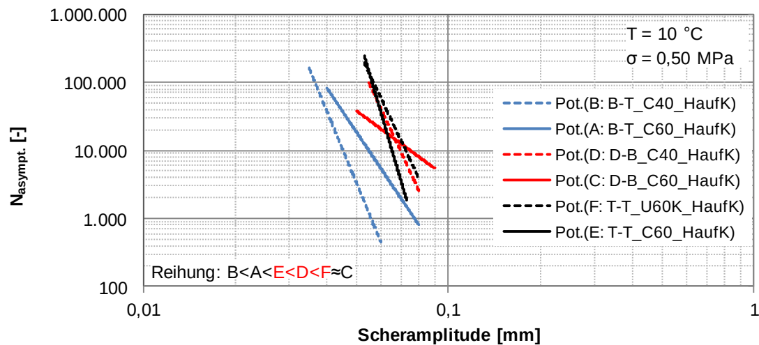
Abbildung 101. Wöhler-Linien für die Verbundvarianten A bis F bei einer Prüftemperatur von 10\text{ °C} und bei einer Normalspannung von 0,50\text{ MPa} mit einer Reihung der Verbundvarianten bezüglich der Scherermüdungsbeständigkeit.
