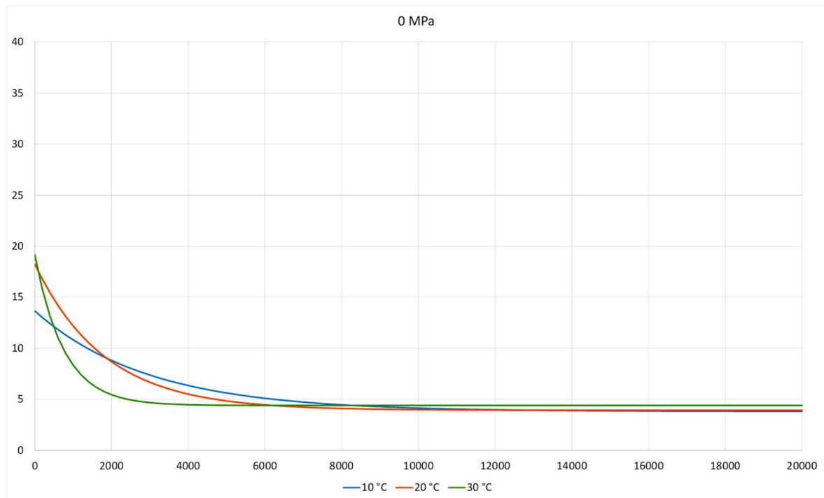
Abbildung 5.60: Ermüdungsfunktionen des Schichtenverbundes für die Temperaturen 10°C, 20°C und 30°C bei fehlender Normalspannung
