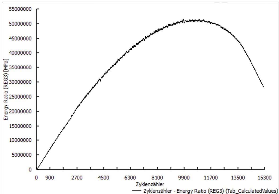
Abbildung 5.75: Bestimmung der Lastwechselzahl N_{\text{Makro}} bis zum Kriterium „Makroriss“ (Probekörper Nr. 7 AC 22 T S, siehe Anhang 10)
