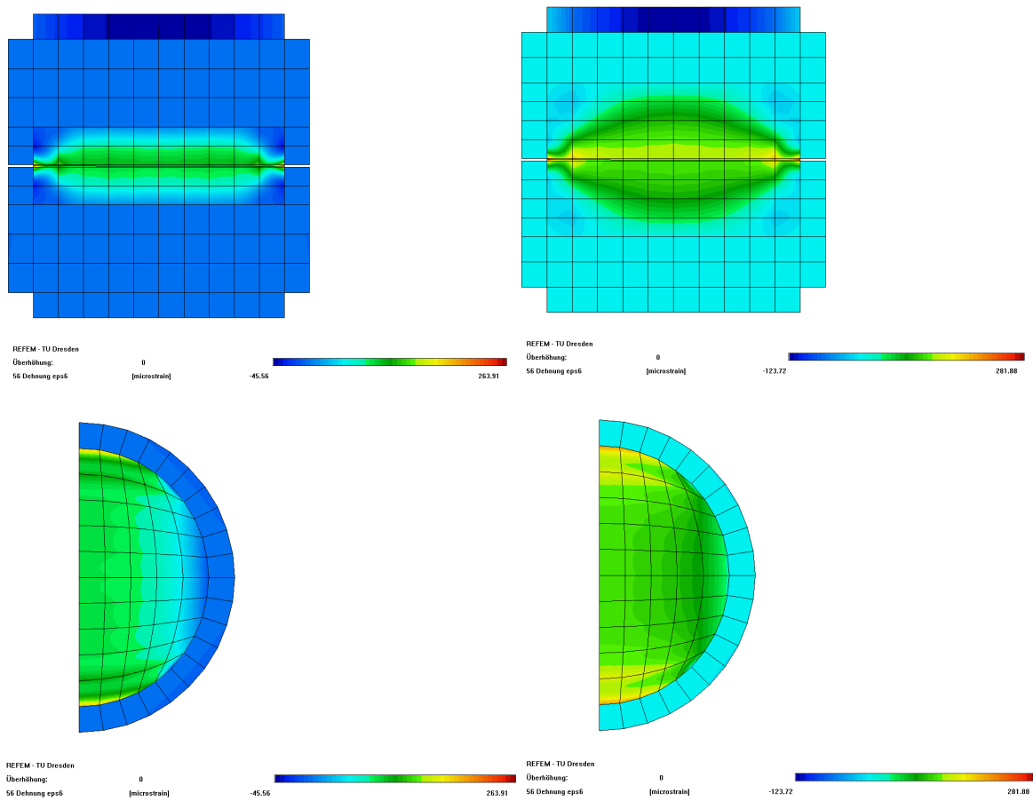
Abbildung 5.15: Dehnungen \epsilon_{ZY} bei G_S = 100\,000 MPa/mm, T = -10^\circ\text{C} bei einer Schichtdicke von 15 mm (links) und 30 mm (rechts)
