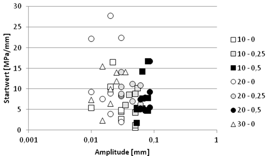
Abbildung 85. Verbundvariante F: Darstellung der Werte des Parameters a_1 über die Scher-amplitude.
