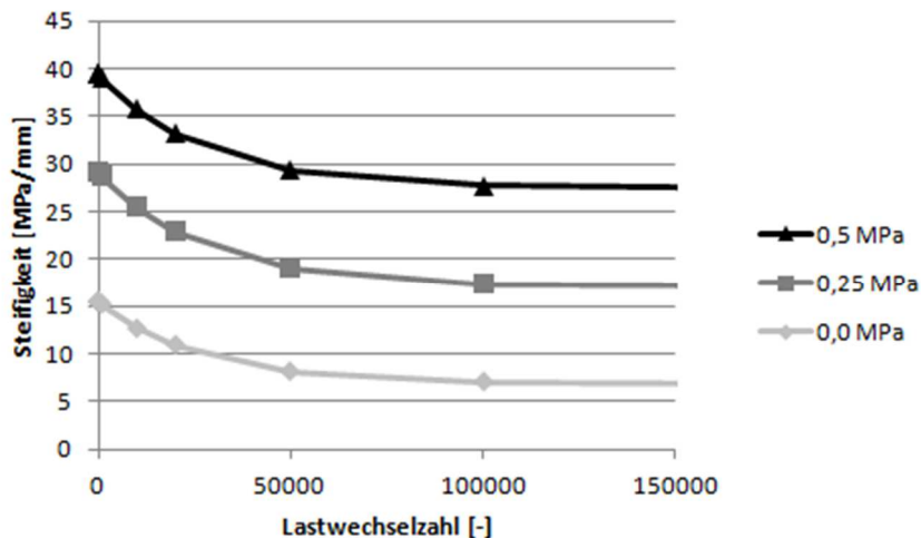
Abbildung 92. Verbundvariante A: Simulation des Schersteifigkeitsverlaufes in Abhängigkeit von der Normalspannung für 0,5 MPa, 0,25 MPa und 0,00 MPa für eine Scheramplitude von \epsilon = 0,02 mm und eine Prüftemperatur von T = 20^\circ\text{C} .
