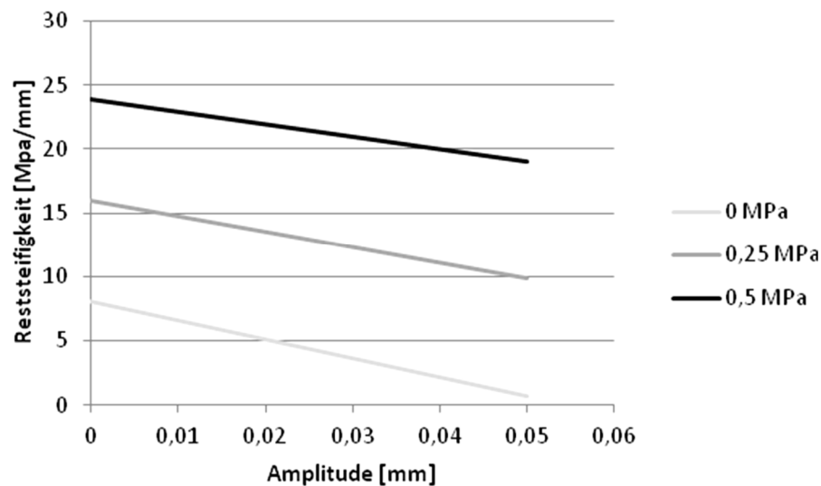
Abbildung 80. Verbundvariante F: Abhängigkeit der Restschersteifigkeit a_0 von der Normalspannung und der Scheramplitude.
