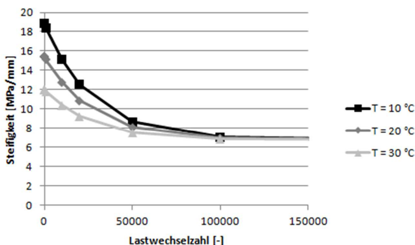
Abbildung 91. Verbundvariante A: Simulation des Schersteifigkeitsverlaufes in Abhängigkeit von der Prüftemperatur für 10 °C, 20 °C und 30 °C für eine Scheramplitude von \varepsilon = 0,02 mm und eine Normalspannung von \sigma = 0,0 MPa.
