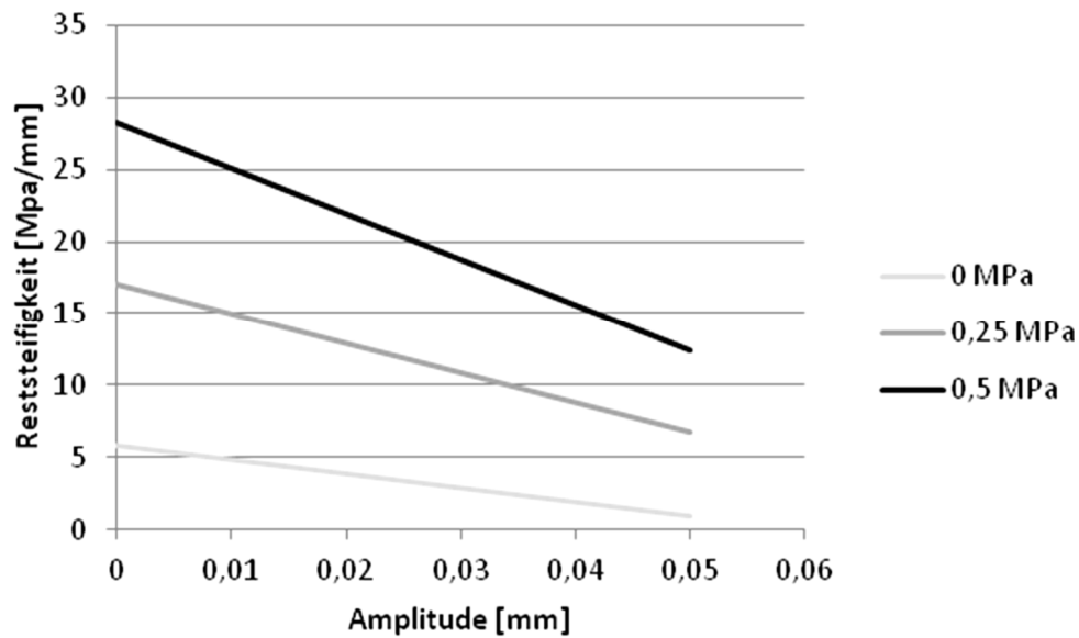
Abbildung 76. Verbundvariante B: Abhängigkeit der Restschersteifigkeit a_0 von der Normalspannung und der Scheramplitude.
