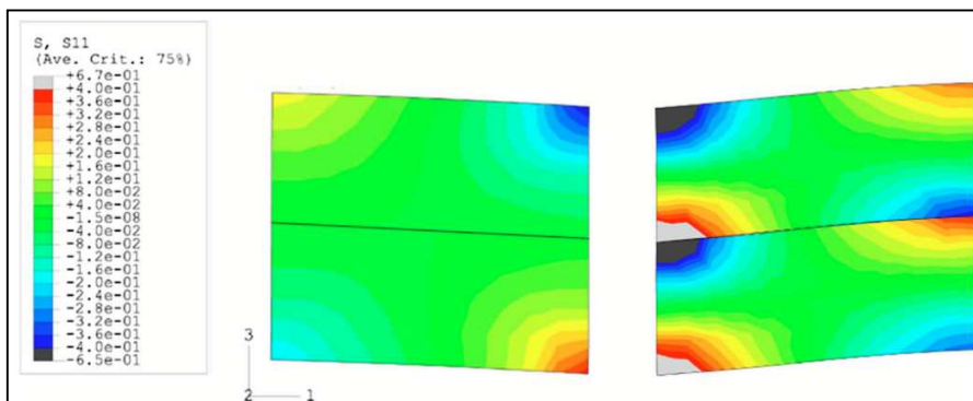
Abbildung 2.29: Spannungen bei vollem Verbund (links) und bei fehlendem Verbund (rechts) nach Kim u.a. (2011)
