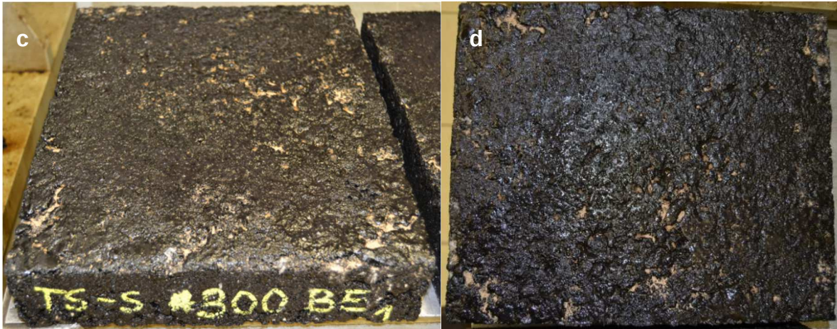
Abbildung 5.52: Beispiel einer stark verschmutzten Oberfläche. a – 15 g/Platte aufgestreuter Schluff, b – mit 10 g Wasser angefeuchtete Oberfläche, c und d – mittelverschmutzte Oberfläche mit aufgetragener Bitumenemulsion (300 g/m 2 )
