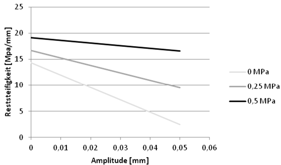
Abbildung 79. Verbundvariante E: Abhängigkeit der Restschersteifigkeit a_0 von der Normalspannung und der Scheramplitude.
