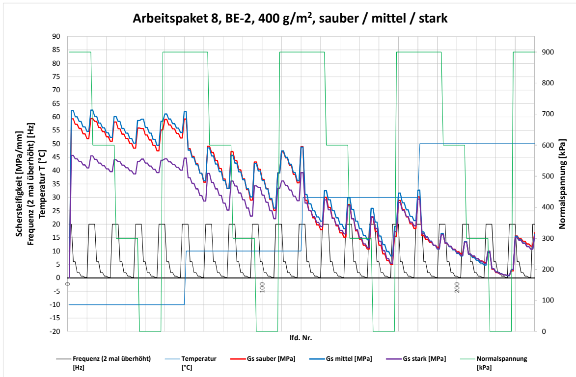
Abbildung 5.58: Vergleich der experimentell ermittelten Schersteifigkeiten bei sauberer, mittel und stark verschmutzter Oberfläche und 400 g/m 2 Bitumenemulsionsmenge
