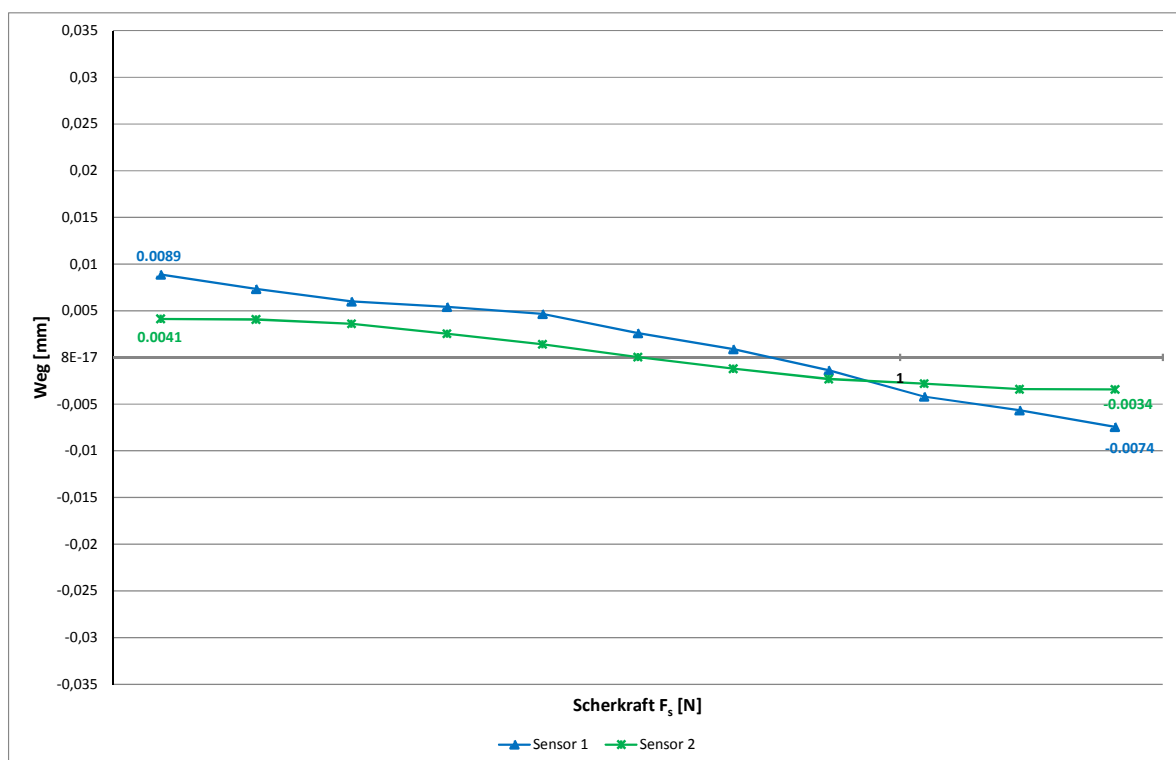
Abbildung 5.6: Vertikale Abweichungen des vertikal beweglichen Trägers B (Sensor 1) und des horizontal beweglichen Trägers A (Sensor 2) beim Wechsel der Scherlast von 5000 N bis -5000 N
