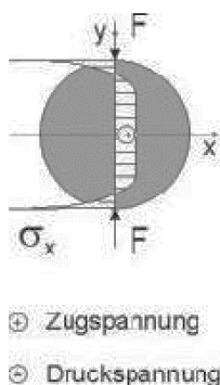
Abbildung 3.16: Horizontaler Spannungsverlauf im zylindrischen Probekörper beim Spaltzug-Schwellversuch nach AL Sp-Asphalt 09
