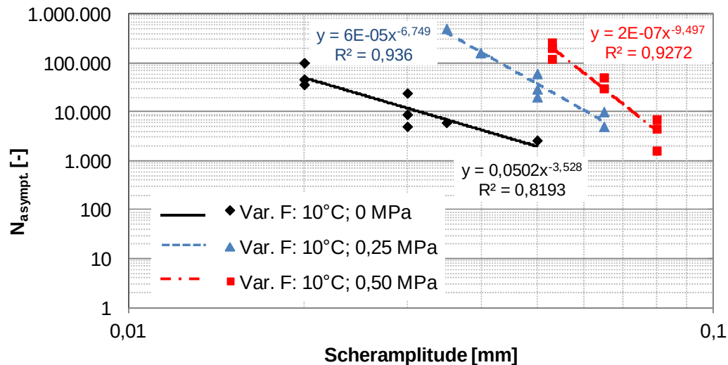
Abbildung 46. Wöhler-Linien für Verbundvariante F bei einer Prüftemperatur von 10 °C und bei drei verschiedenen Normalspannungen (0 MPa, 0,25 MPa und 0,50 MPa).
