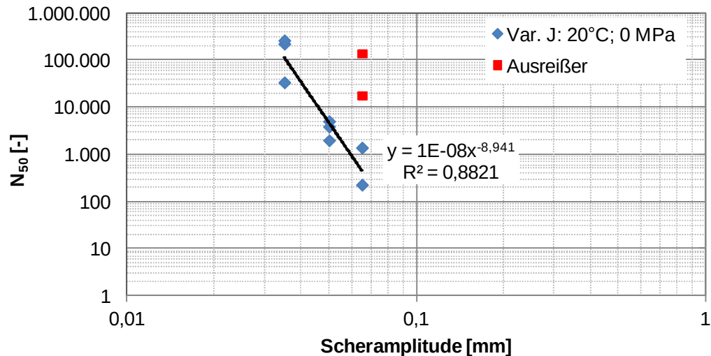
Abbildung 42. Verbundvariante J: Ermüdungspotenzfunktion (Wöhler-Linie) bei 20 °C und 0 MPa Normalspannung.
