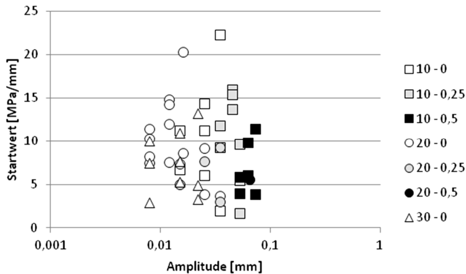
Abbildung 84. Verbundvariante E: Darstellung der Werte des Parameters a_1 über die Scher-amplitude.
