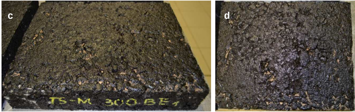
Abbildung 5.51: Beispiel einer mittel verschmutzten Oberfläche. a – 15 g/Platte aufgestreuter Schluff, b – mit 10 g Wasser angefeuchtete Oberfläche, c und d – mittelverschmutzte Oberfläche mit aufgetragener Bitumenemulsion (300 g/m 2 )
