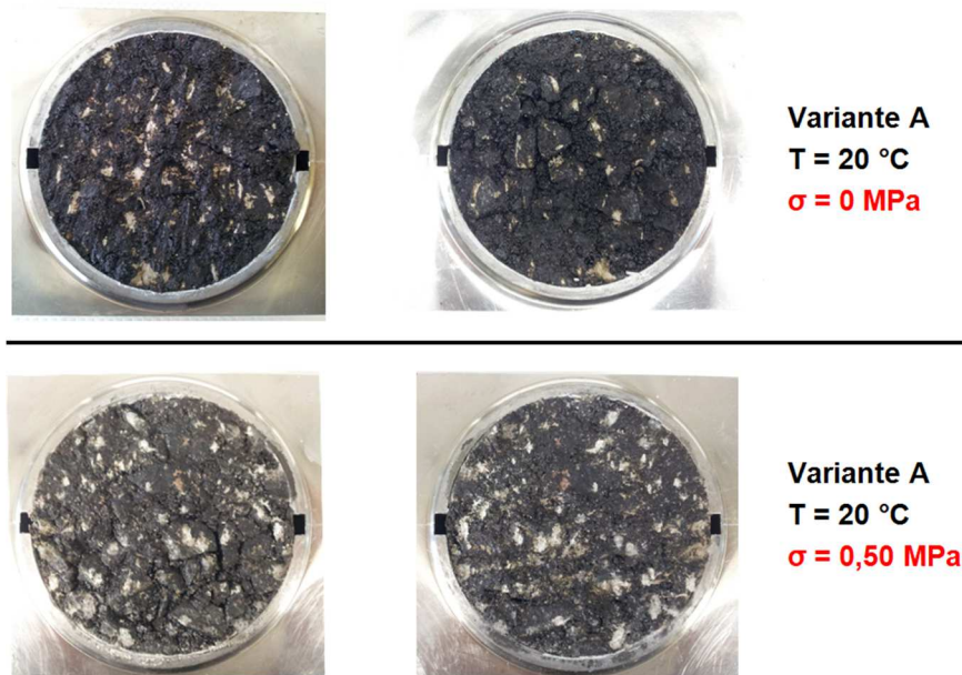
Abbildung 44. Verbundvariante A: Zwei Seiten der Schichtgrenze nach der Scherermüdungsprüfung bei 20 °C, ohne Normalspannung (oben) und bei einer Normalspannung von 0,50 MPa (unten).
