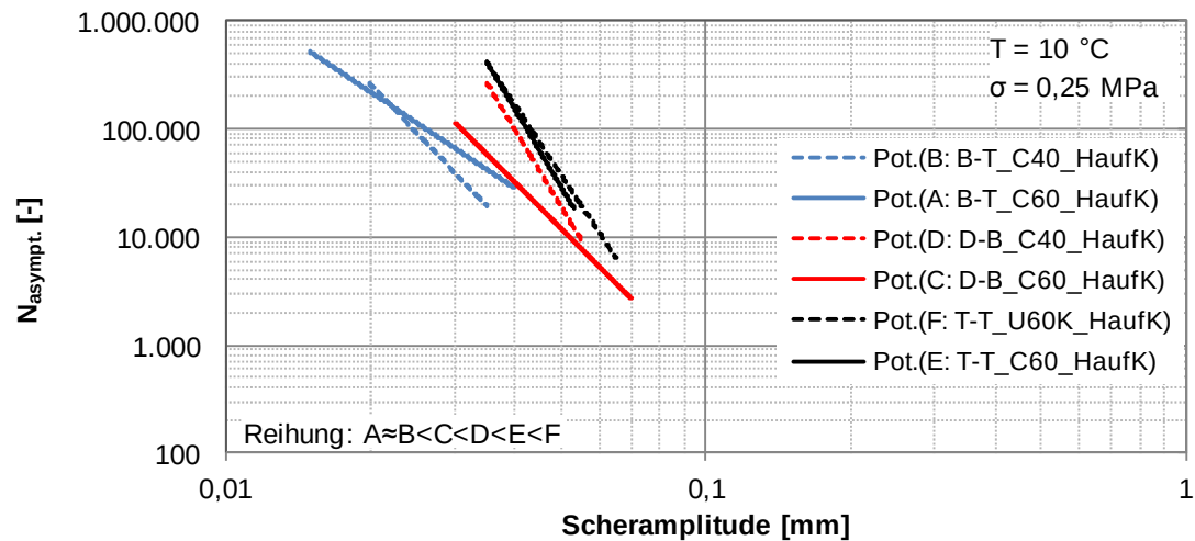
Abbildung 99. Wöhler-Linien für die Verbundvarianten A bis F bei einer Prüftemperatur von 10 °C und bei einer Normalspannung 0,25 MPa mit einer Reihung der Verbundvarianten bezüglich der Scherermüdungsbeständigkeit.
