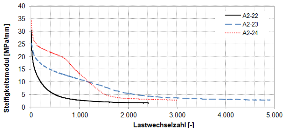
Abbildung 61: Exemplarische Schersteifigkeitsverläufe von drei Probekörpern der Verbundvariante A bei den Prüfparametern T = 20\text{ °C} , \sigma = 0\text{ MPa} und \epsilon = 0,05\text{ mm} .
