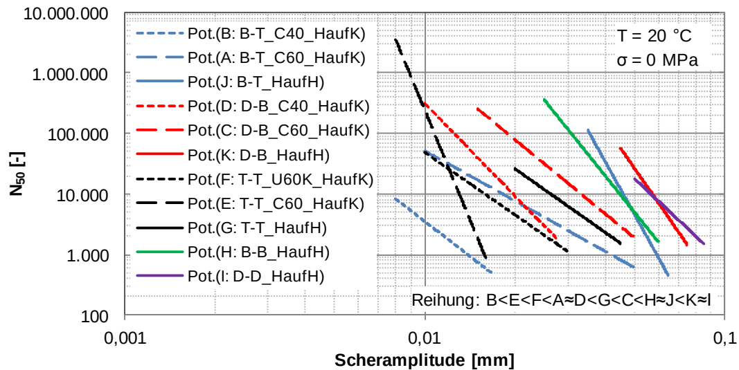
Abbildung 94. Wöhler-Linien für die Verbundvarianten A bis K bei einer Prüftemperatur von 20 °C und ohne Normalspannung mit einer Reihung der Verbundvarianten bezüglich der Scherermüdungsbeständigkeit.
