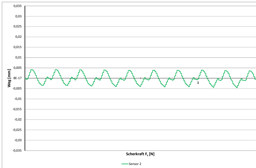
Abbildung 5.3: Wiederholung der statisch aufgetragenen Scherlast von 5000 N bis -5000 N zur Bestimmung der Bewegungen der Bauteile der Prüfvorrichtung
