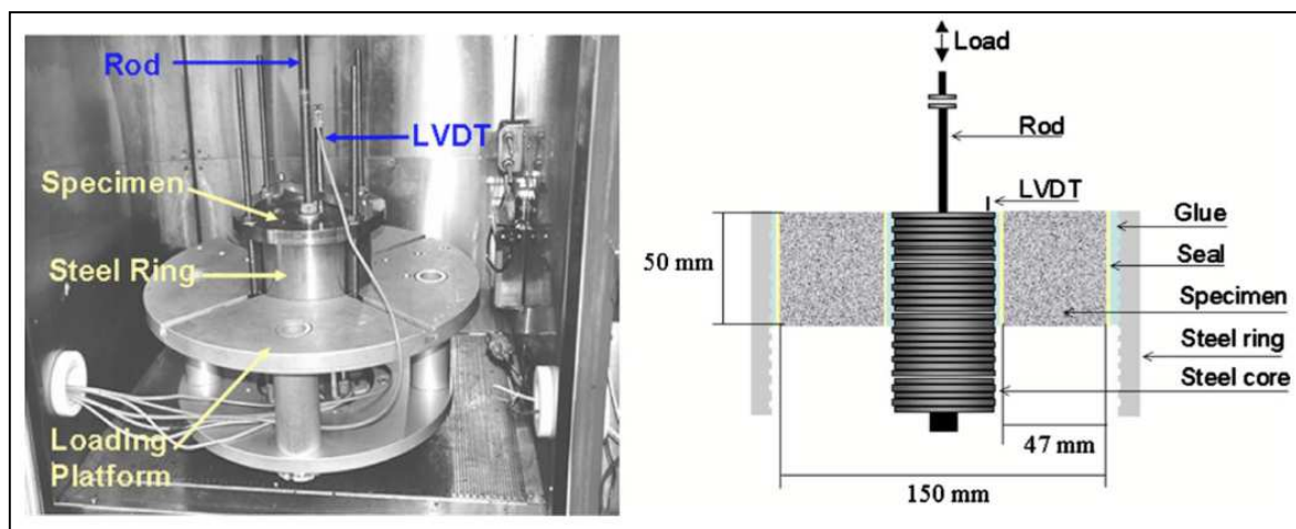
Abbildung 2.27: Prüfgerät CAST (links) und Dimensionen (rechts) nach Sokolov u.a. (2005) und Kim u.a. (2011)
