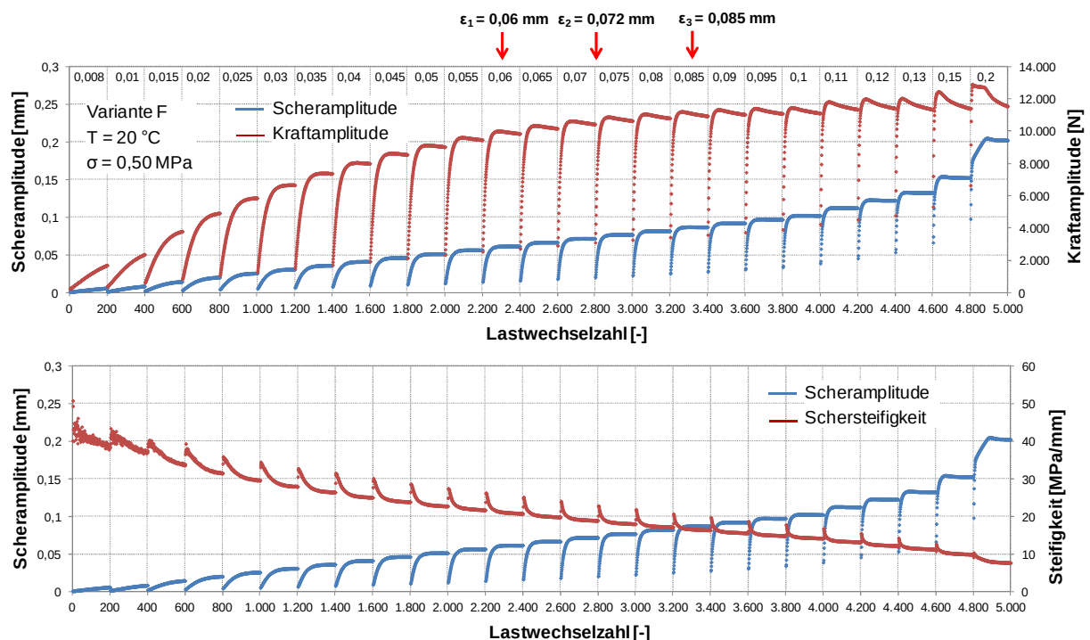
Abbildung 30. Verbundvariante F: Verläufe der Kraft (oben) und der Schersteifigkeit (unten) während des Amplitudensweeps bei 20 °C und 0,50 MPa Normalspannung.
