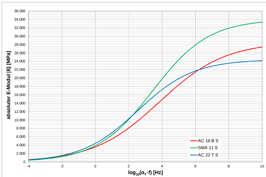
Abbildung 5.71: Masterfunktionen der drei Materialien
