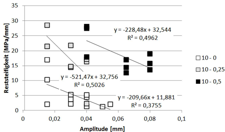
Abbildung 64. Verbundvariante A: Lineare Regressionen der Restschersteifigkeit a_0 in Abhängigkeit von der Scheramplitude für eine Prüftemperatur von T = +10\text{ °C} .
