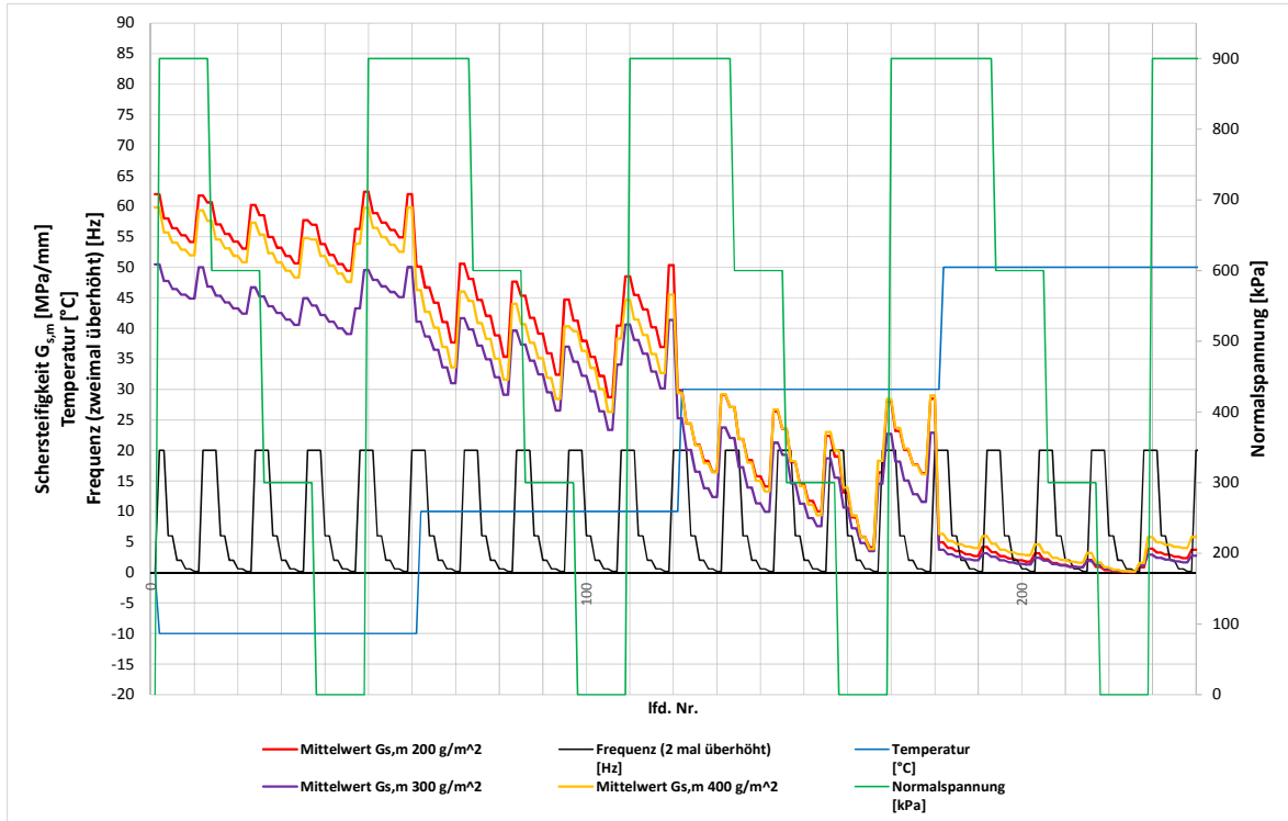
Abbildung 5.28: Mittelwerte der versuchstechnisch ermittelten Schersteifigkeiten des normal hergestellten Schichtenverbundes bei 200 g/m 2 , 300 g/m 2 und 400 g/m 2
