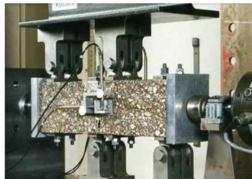
Abbildung 13. Ermittlung der Schersteifigkeit unter zyklischer Vier-Punkt-Biegung (de Bondt, 1999).
