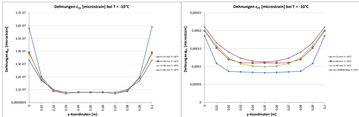
Abbildung 5.19: Dehnungen \varepsilon_{zy} bei fehlendem (links) und vollem (rechts) Verbund, T = -10^\circ\text{C}
