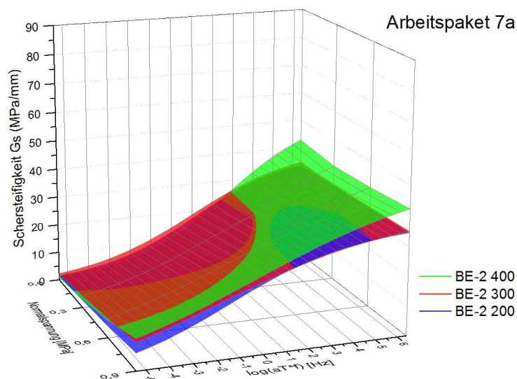
Abbildung 5.42: Flächenfunktionen der berechneten Schersteifigkeiten bei Anwendung der Bitumenemulsion C60 BP1-S von dem Hersteller Nr. 2 auf fein geschliffenen Oberflächen
