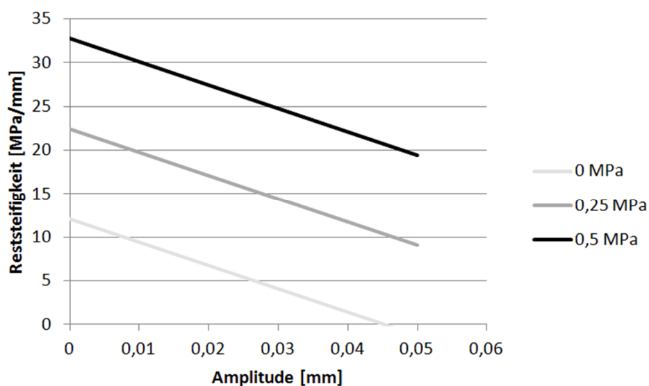
Abbildung 66. Verbundvariante A: Abhängigkeit der Restschersteifigkeit a_0 von der Normalspannung und der Scheramplitude.
