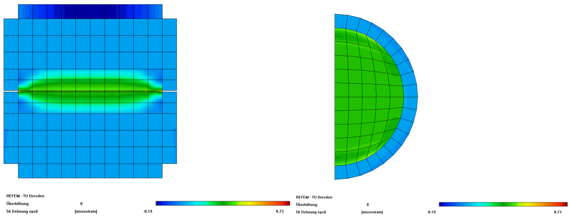
Abbildung 5.17: Dehnungen \epsilon_{zy} bei G_s = 100 MPa/mm, T = -10^\circ\text{C} bei einer Schichtdicke von 15 mm
