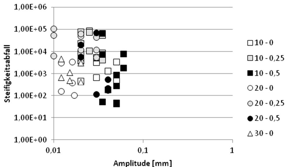
Abbildung 86. Verbundvariante B: Alle Werte des Schersteifigkeitsabfalls a_3 in Abhängigkeit von der Scheramplitude.
