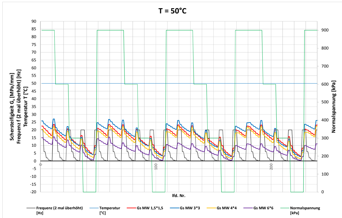
Abbildung 5.23: Schersteifigkeitsverläufe für die vier untersuchten Schichtdicken bei 50°C
