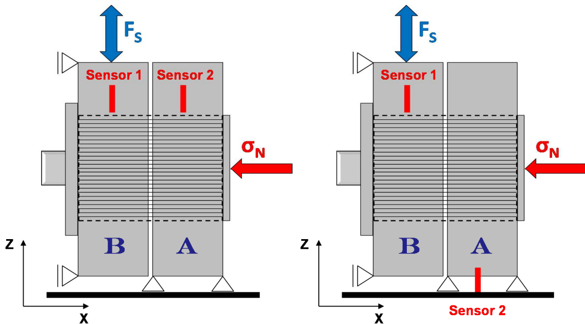
Abbildung 5.2: Anordnung der Wegsensoren zur Überprüfung der Bewegungen der Bauteile der Prüfvorrichtung während der Versuchsdurchführung
