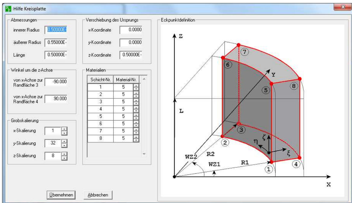
Abbildung 3.24: Element Kreisplatte für die Stahlschalen
