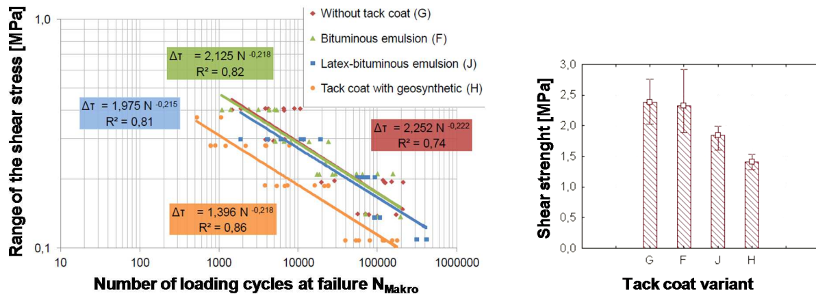
Abbildung 18. Ermüdungsfunktionen aus zyklischen Scherversuchen für verschiedene Verbundvarianten an Schichtenverbund (links); Scherfestigkeiten aus statischen Abscherversuchen für die gleichen Verbundvarianten (rechts) (Górszczyk & Malicki, 2012).
