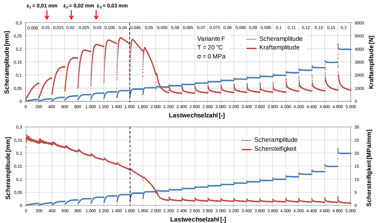
Abbildung 28. Verbundvariante F: Verläufe der Kraft (oben) und der Schersteifigkeit (unten) während des Amplitudensweeps bei 20 °C und 0 MPa Normalspannung.
