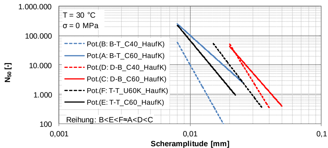
Abbildung 97. Wöhler-Linien für die Verbundvarianten A bis F bei einer Prüftemperatur von 30 °C und ohne Normalspannung mit einer Reihung der Verbundvarianten bezüglich der Scherermüdungsbeständigkeit.
