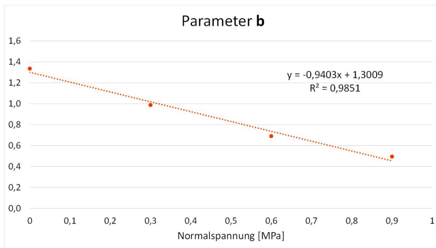
Abbildung 4.7: Funktionale Abhängigkeit der Parameter a und b von der Normalspannung
