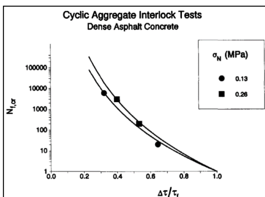
Abbildung 2.21: Effekt des relativen Belastungsgrades auf die Lebensdauer des Probekörpers (de Bondt 1999)
