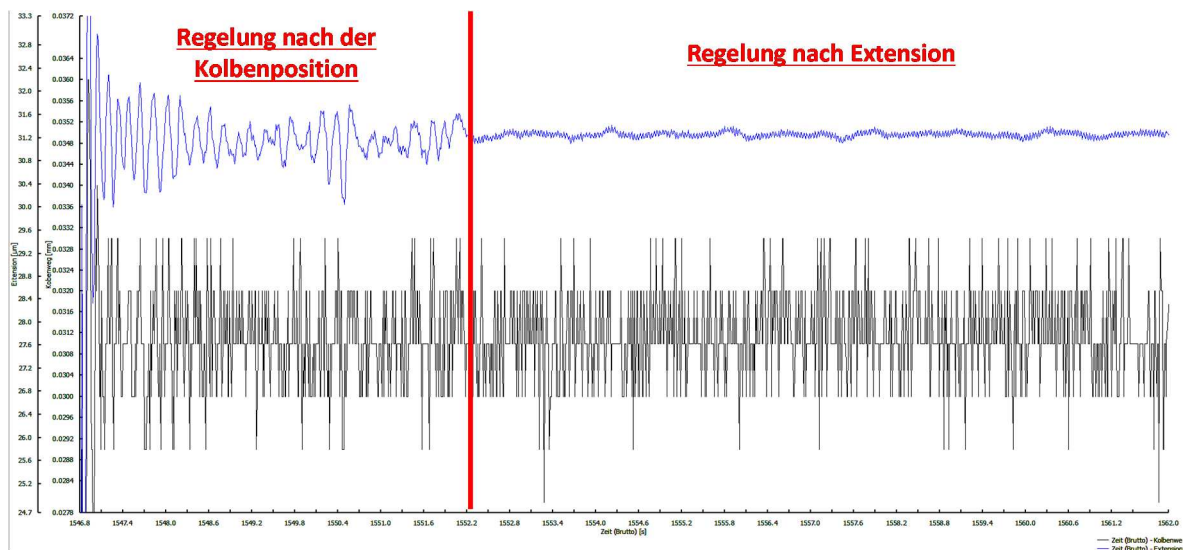
Abbildung 5.1: Verbesserte Präzision der Regelung bei der neu entwickelten Prüfvorrichtung
