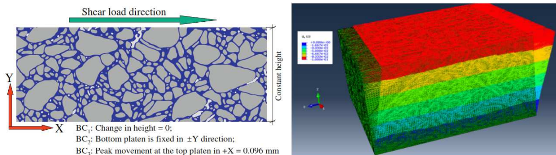
Abbildung 2.32: Schematische Darstellung des Versuches (links) und 3D-Modell in ABAQUS (rechts) nach Coleri u.a. (2011)
