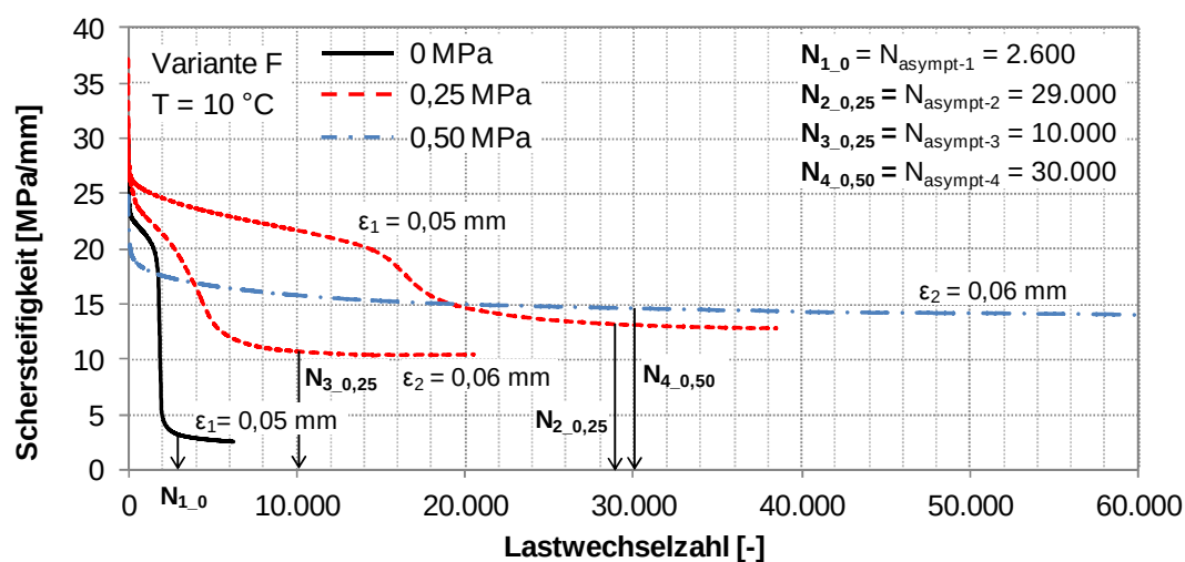
Abbildung 45. Verbundvariante F: Schersteifigkeitsverläufe bei einer Prüftemperatur von 10 °C, bei verschiedenen Normalspannungen (0 MPa, 0,25 MPa und 0,50 MPa) und bei zwei Scheramplituden (0,05 mm und 0,06 mm).
