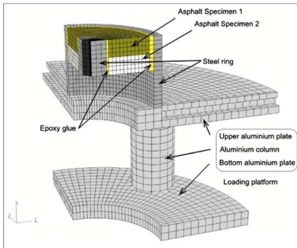
Abbildung 2.28: FE-Modell nach Sokolov u.a. (2005) und Kim u.a. (2011)
