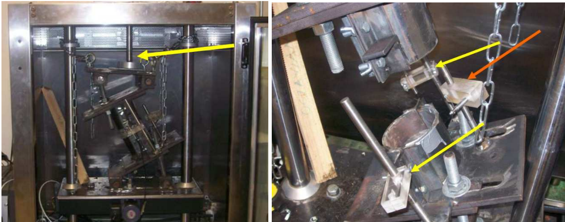
Abbildung 2.18: UTM Prüfvorrichtung nach Wheat (2007) in der Prüfmaschine (links) und Platzierung der induktiven Wegaufnehmer (rechts)
