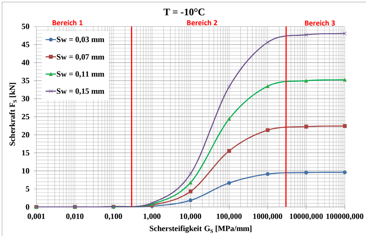
Abbildung 4.10: Funktionaler Zusammenhang zwischen Scherkraft und Schersteifigkeit für alle vier untersuchten maximalen Scherwege bei -10°C
