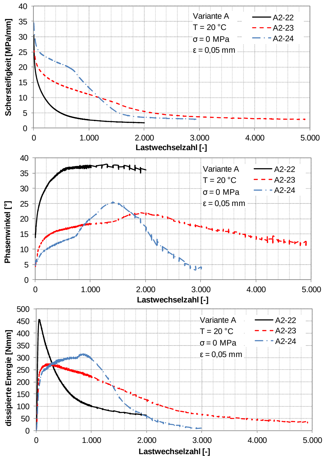
Abbildung 36. Verbundvariante A: Verläufe der Schersteifigkeit (oben), Phasenwinkel (Mitte) und dissipierten Energie pro Lastwechsel (unten) während des zyklischen Scherversuchs bei 0 MPa Normalspannung, 20 °C Prüftemperatur und 0,05 mm Scheramplitude.
