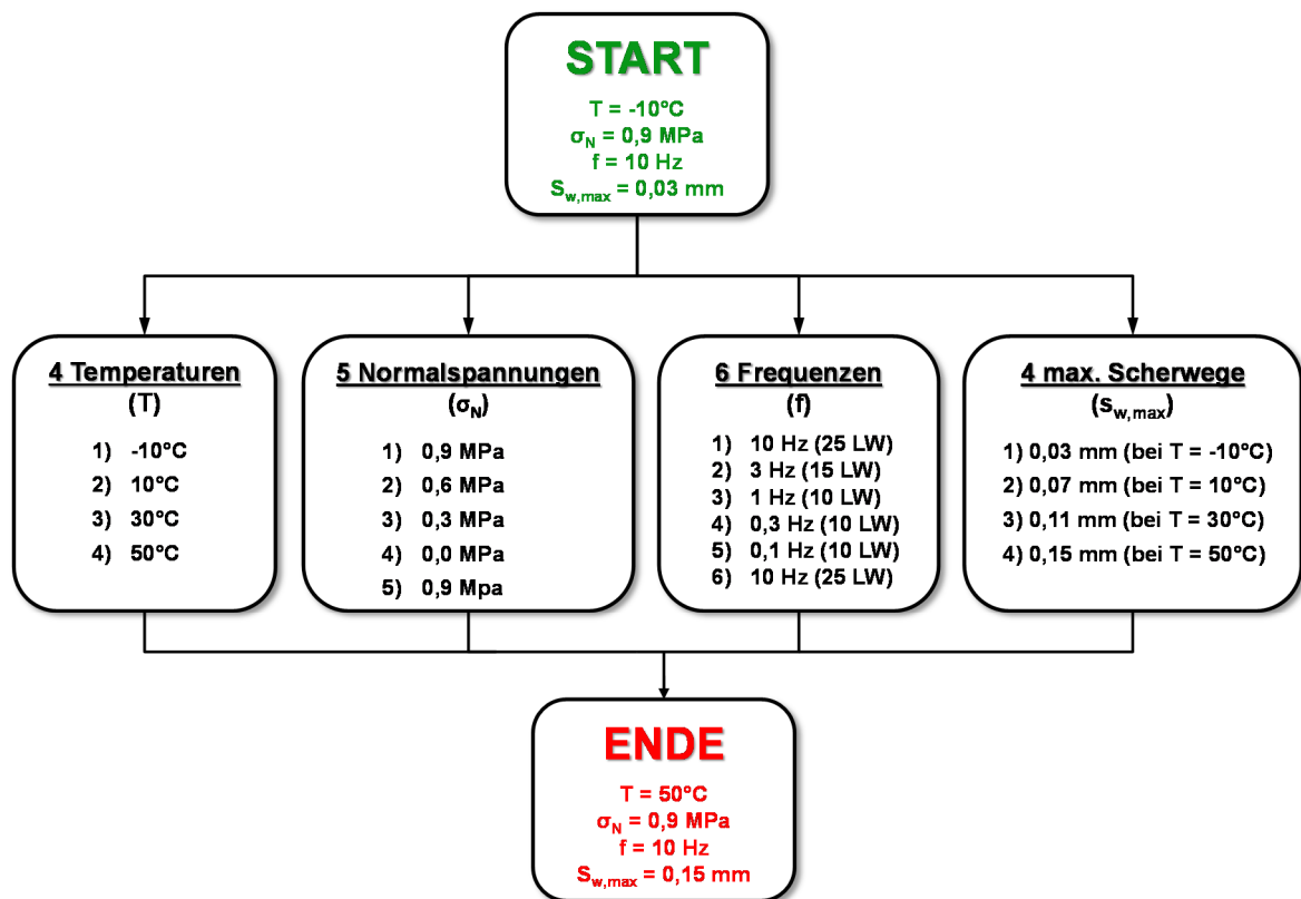
Abbildung 3.15: Prüfprogramm für die zyklischen Schersteifigkeitsversuche
