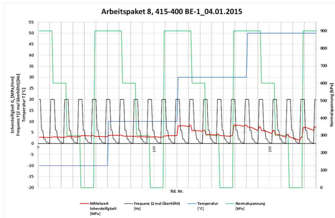
Abbildung 4.3: Beispiel einer konstant bleibenden Schersteifigkeit bei -10°C und 10°C
