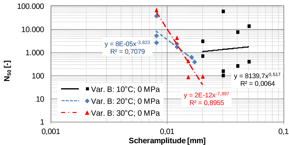
Abbildung 58. Wöhler-Linien für Verbundvariante B bei 0 MPa Normalspannung und bei den Prüftemperaturen 30 °C, 20 °C und 10 °C.
