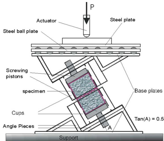
Abbildung 12. Indirekter zyklischer Abscherversuch von Romanoschi und Metcalf (2000).
