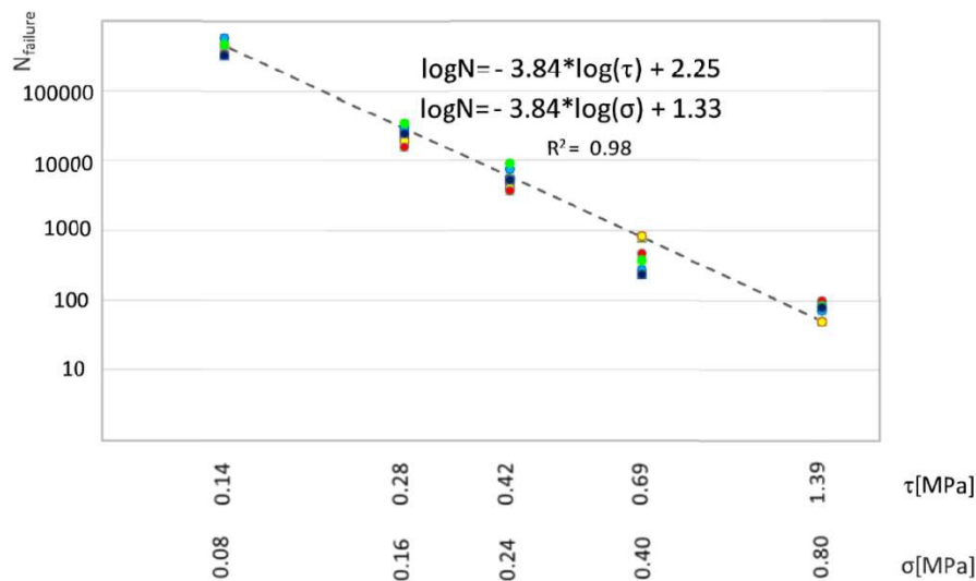
Abbildung 20. Ermüdungswiderstand des Schichtenverbundes im kraftgeregelten, indirekten, zyklischen Scherversuch bei verschiedenen Normalspannungen und bei 20 °C (Tozzo et al. 2014).
