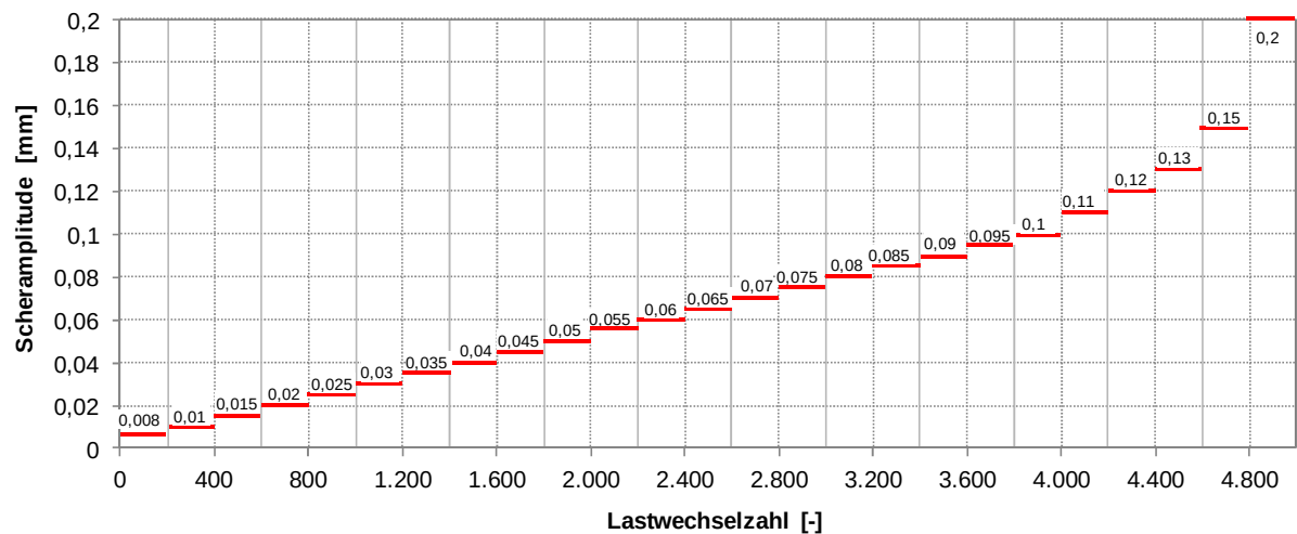
Abbildung 107. Steifigkeitsversuch in Form eines Amplitudensweeps mit dem zyklischen Scherversuch. Stufenweise Erhöhung der Scheramplitude, mit insgesamt 25 Stufen und jeweils 200 Lastwechseln (exemplarisch).
