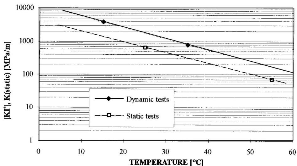
Abbildung 15. Temperaturabhängigkeit der Schersteifigkeiten ermittelt mit dem statischen Abscherversuch (gestrichelte Linie) und mit dem zyklischen Scherversuch (durchgehende Linie) (Crispino et al., 1997).
