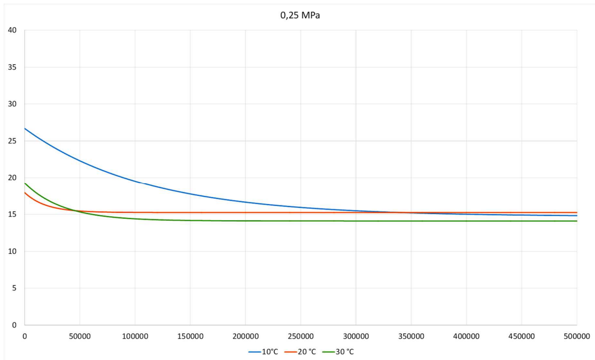
Abbildung 5.61: Ermüdungsfunktionen des Schichtenverbundes für die Temperaturen 10°C, 20°C und 30°C bei einer Normalspannung von 0,25 MPa
