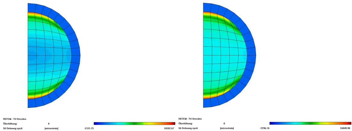
Abbildung 5.16: Dehnungen \epsilon_{zy} bei G_s = 100\,000 MPa/mm, T = 50^\circ\text{C} bei einer Schichtdicke von 15 mm (links) und 30 mm (rechts)
