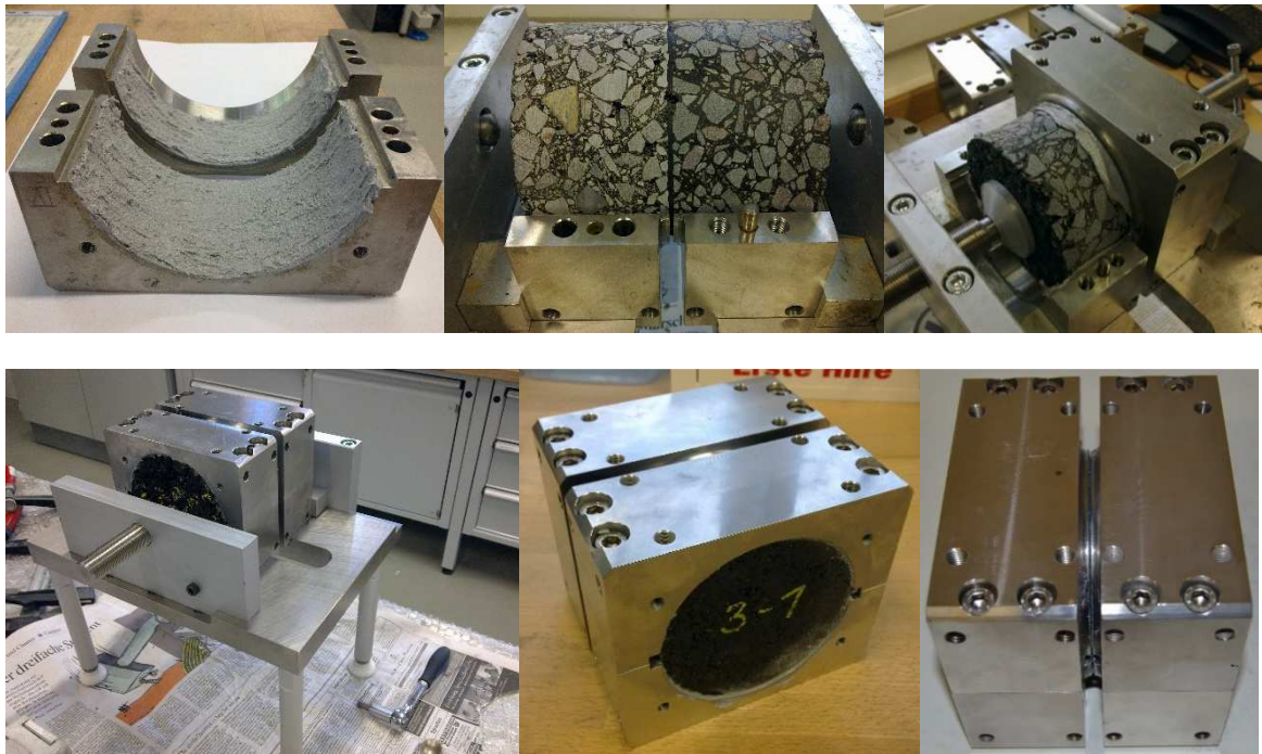
Abbildung 3.3: Einkleben des Asphaltprobekörpers in der Klebevorrichtung
