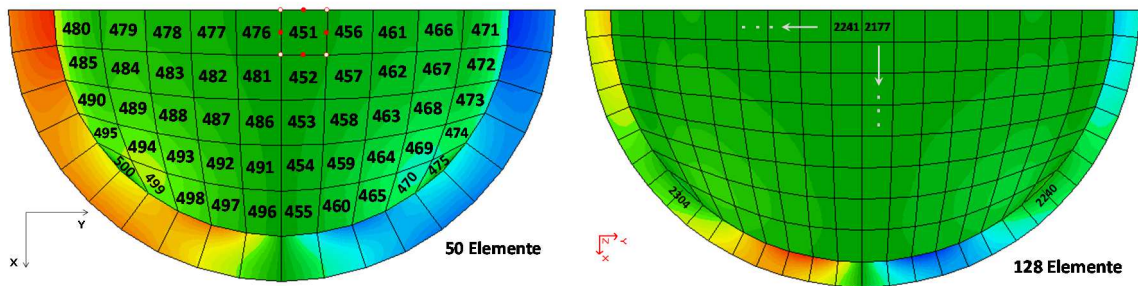
Abbildung 3.30: Zuordnung der Elemente und der Knoten im Interface
