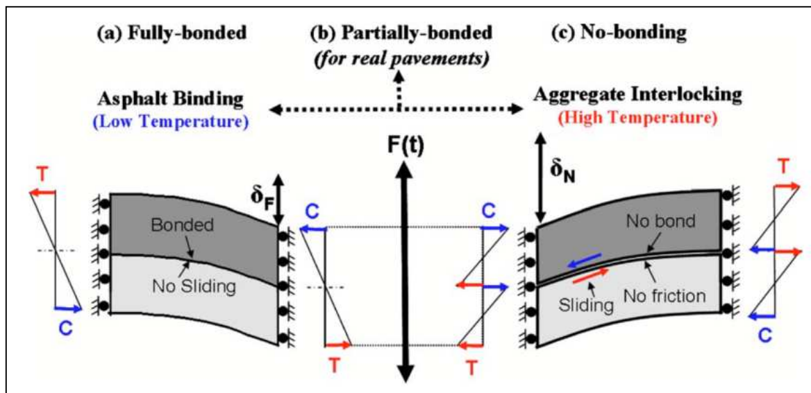
Abbildung 2.26: Schematische Darstellung des Zug-Druck Verhaltens von zweischichtigen Probekörpern für den Fall einer Biegung zwischen zwei parallelen Platten
