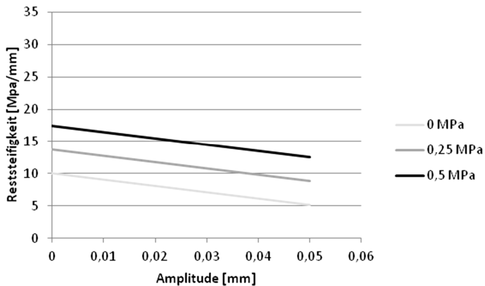
Abbildung 77. Verbundvariante C: Abhängigkeit der Restschersteifigkeit a_0 von der Normalspannung und der Scheramplitude.
