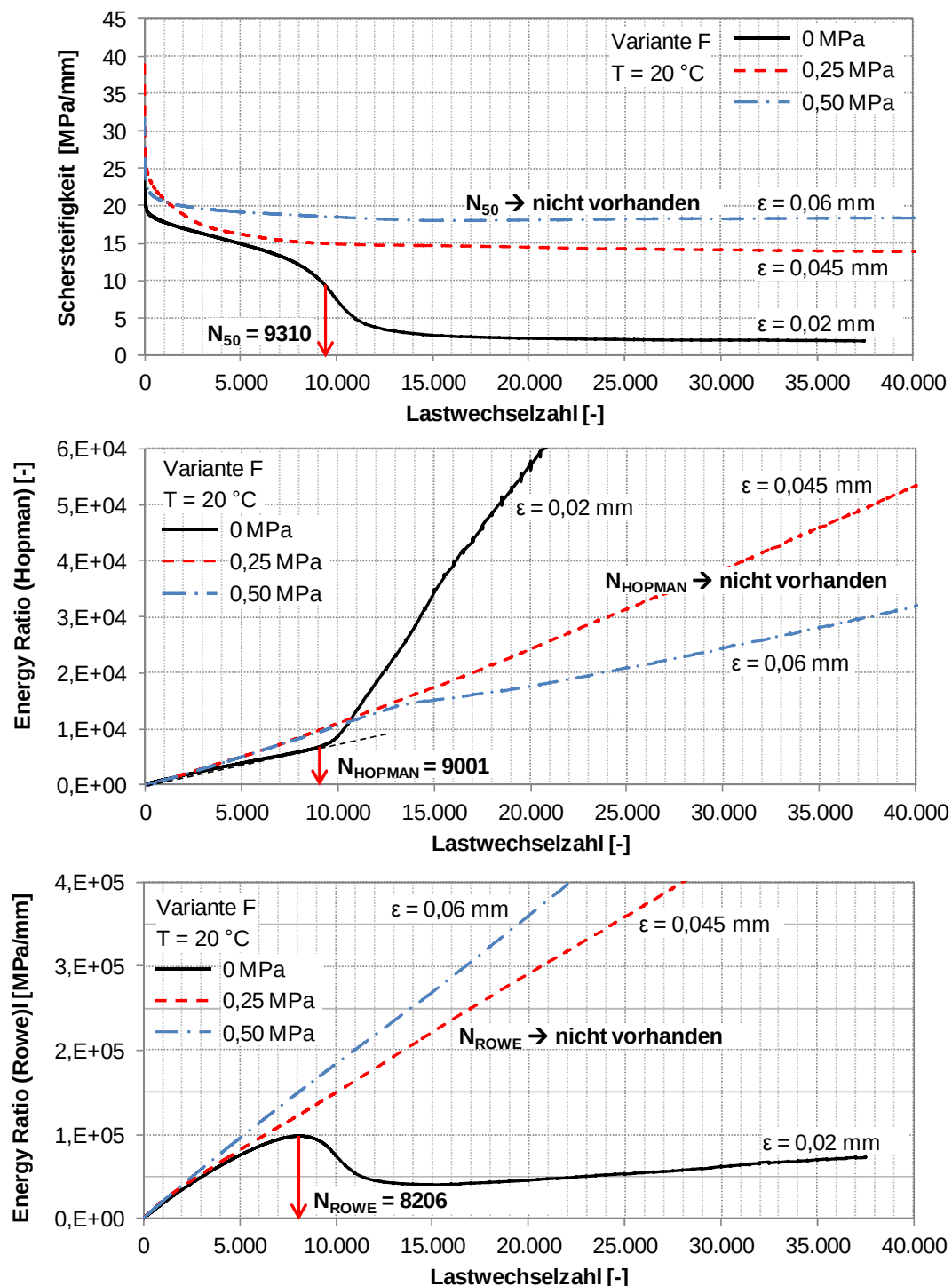
Abbildung 38. Verbundvariante F: Verläufe der Schersteifigkeit (oben), Energierate nach Hopman (Mitte) und Energierate nach Rowe (unten) während des zyklischen Scherversuchs bei 20 °C und 0 MPa, 0,25 MPa und 0,50 MPa Normalspannung.
