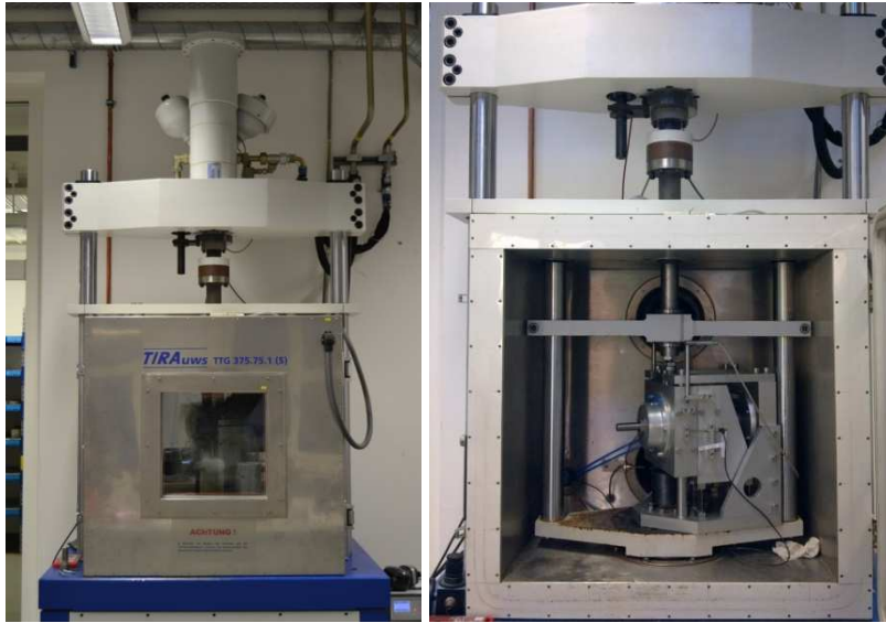
Abbildung 3.5: Prüfmaschine SHM 63 mit Temperierkammer der TU Dresden
