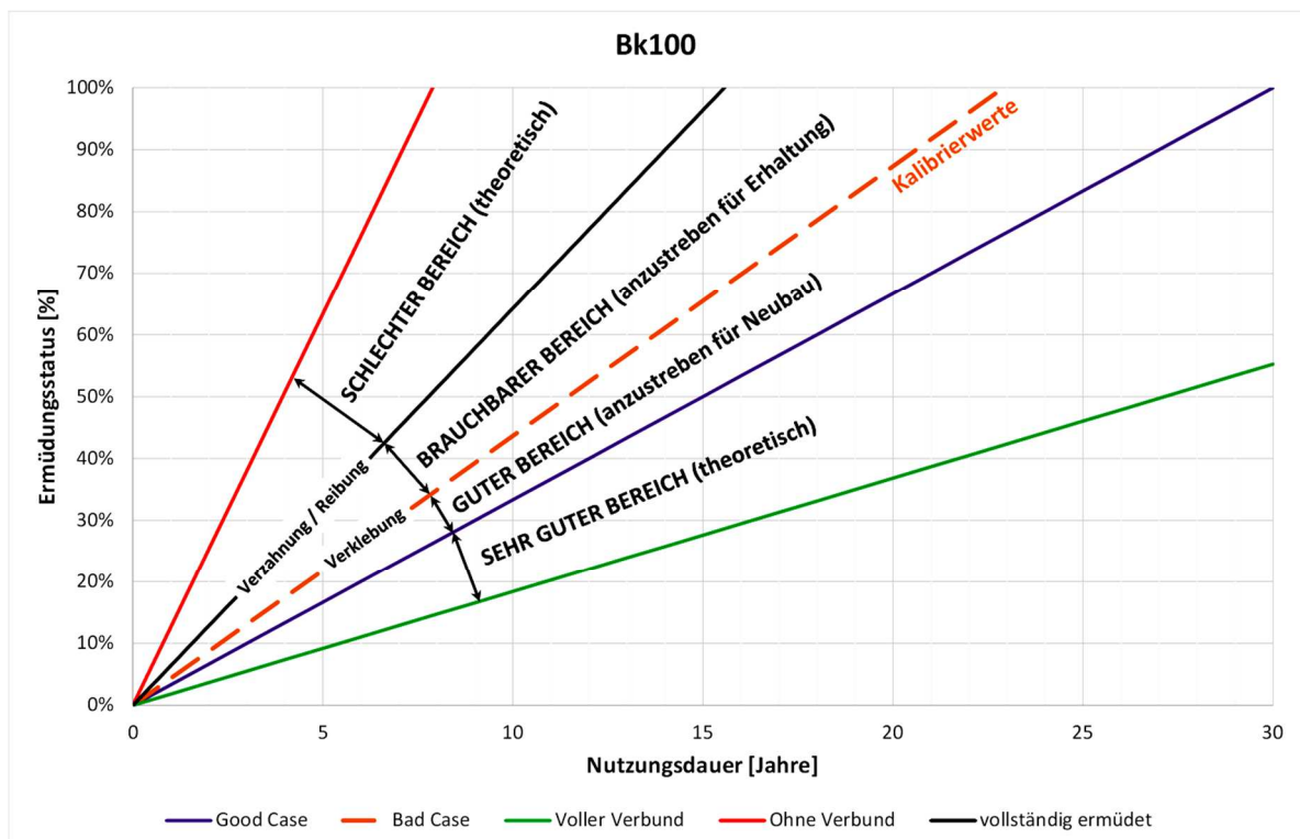
Abbildung 5.67: Qualitätsbereiche des Schichtenverbundes für Neubau und Erhaltung (Bk100)
