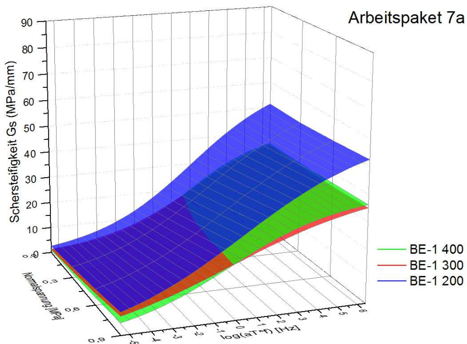
Abbildung 5.40: Flächenfunktionen der berechneten Schersteifigkeiten bei Anwendung der Bitumenemulsion C60 BP1-S von dem Hersteller Nr. 1 auf fein geschliffenen Oberflächen
