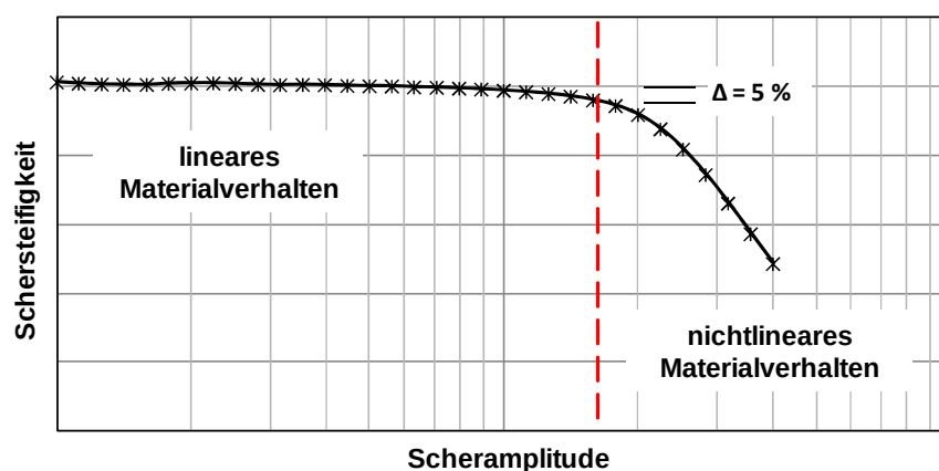
Abbildung 108. Prinzip der Ermittlung des linear-visko-elastischen Bereichs bei einem Amplitudensweep: die rot gestrichelte Linie markiert die Grenze des linearen Materialverhaltens, ab der bei einer konstanten Scheramplitude die Schersteifigkeit um mehr als 5 % vom Startwert abweicht (Anderson et al., 1994).
