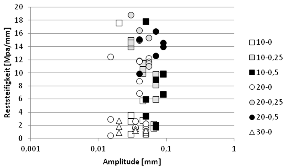
Abbildung 72. Verbundvariante C: Alle Werte der Restschersteifigkeit a_0 in Abhängigkeit von der Scheramplitude.
