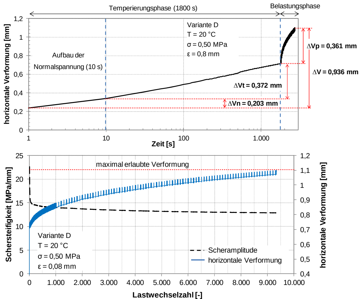
Abbildung 49. Verbundvariante D: Verläufe der horizontalen Verformung und der Schersteifigkeit während der Scherermüdungsprüfung bei 20 °C, 0,50 MPa Normalspannung und 0,08 mm Scheramplitude. \Delta V_n ...Anstieg der Verformung während des Aufbaus der Normalspannung; \Delta V_t ...Anstieg der Verformung während der Temperierung; \Delta V_p ...Anstieg der Verformung während der zyklischen Belastung.
