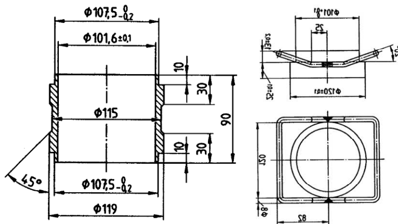
Abbildung 3.18: Formzylinder und Formgrundplatte nach DIN EN 12697-30 (2004)
