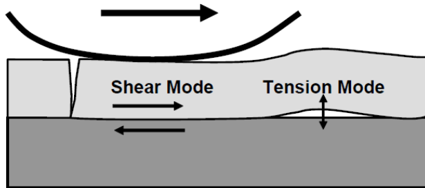
Abbildung 9. Scher- und Zugbeanspruchungen, die durch Achsbelastung an der Schichtgrenze entstehen (Raab & Partl, 2004).
