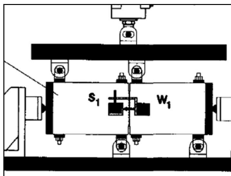
Abbildung 13. Ermittlung der Schersteifigkeit unter zyklischer Vier-Punkt-Biegung (de Bondt, 1999).
