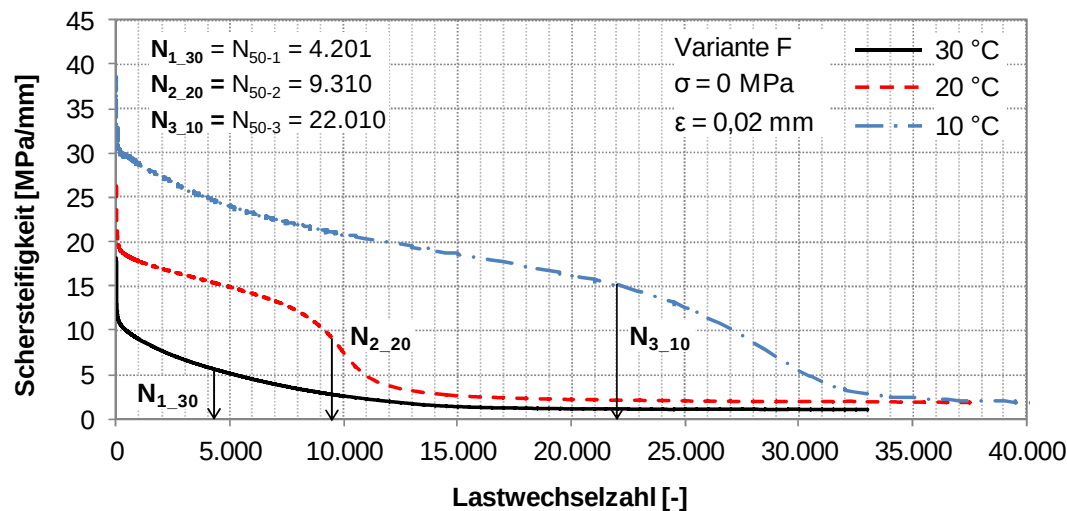
Abbildung 55. Verbundvariante F: Verläufe der Schersteifigkeit während der Scherermüdungsprüfung bei 0 MPa Normalspannung, bei verschiedenen Temperaturen (30 °C, 20 °C und 10 °C) und bei einer Scheramplitude (0,02 mm).
