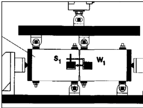
Abbildung 2.20: Position der induktiven Wegaufnehmer, die an dem Probekörper befestigt sind (de Bondt, 1999)
