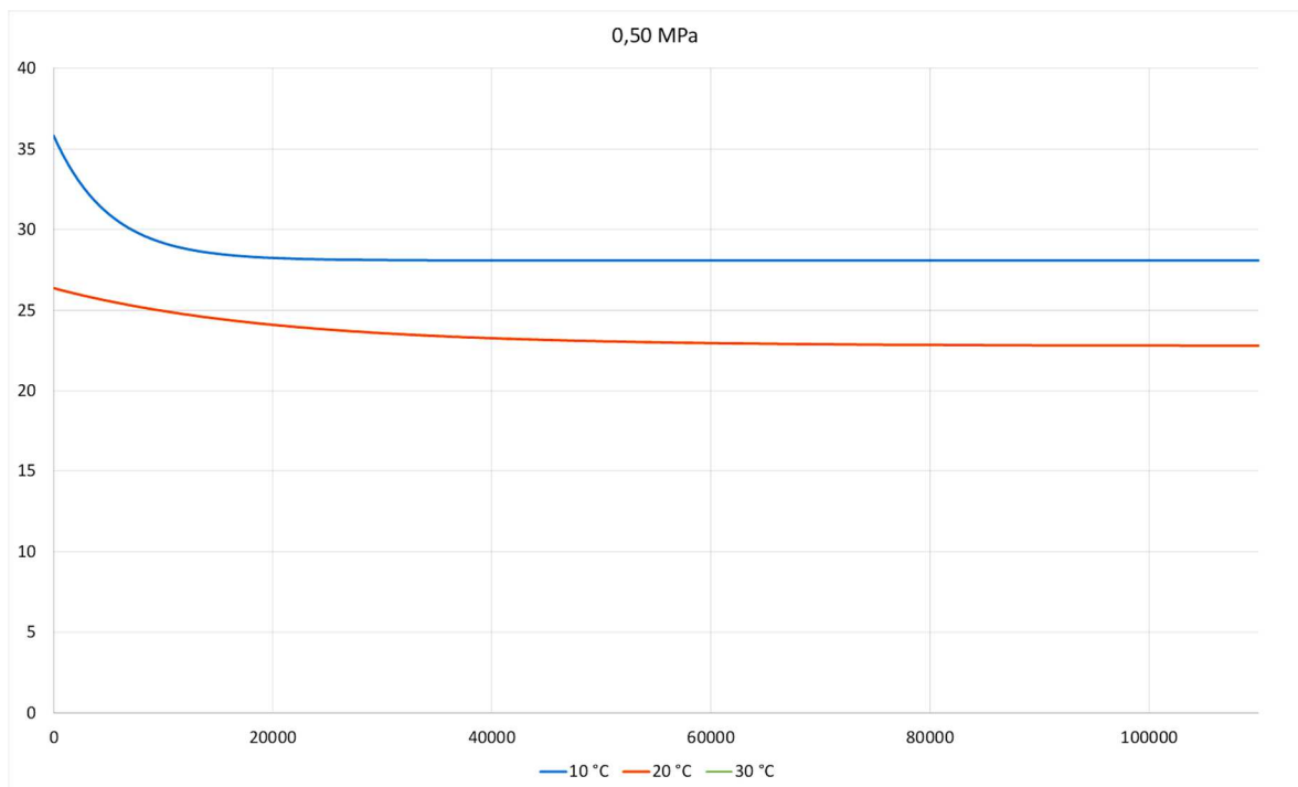
Abbildung 5.62: Ermüdungsfunktionen des Schichtenverbundes für die Temperaturen 10°C und 20°C bei einer Normalspannung von 0,50 MPa
