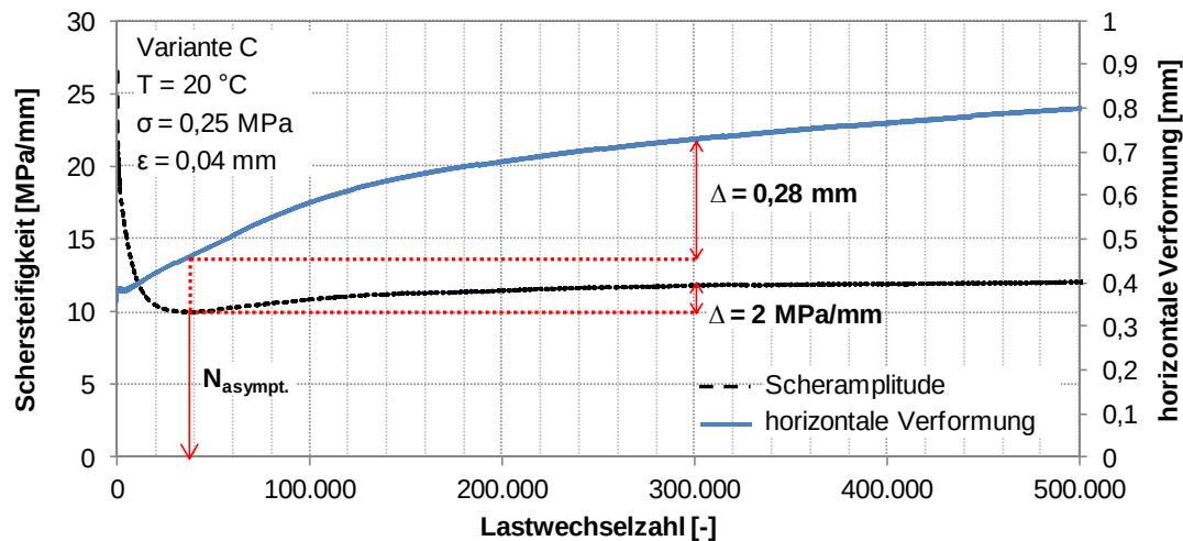
Abbildung 51. Verbundvariante C: Verläufe der Schersteifigkeit und der horizontalen Verformung während der Scherermüdungsprüfung bei 20 °C, 0,25 MPa Normalspannung und 0,04 mm Scheramplitude.
