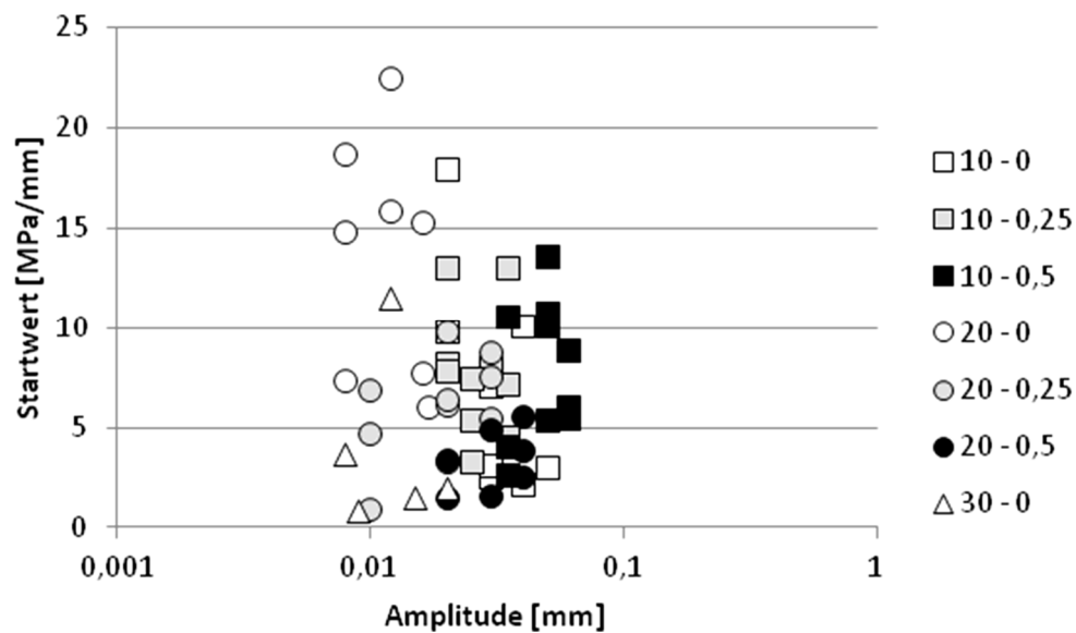
Abbildung 81. Verbundvariante B: Alle Startwerte der Schersteifigkeit a_1 in Abhängigkeit von der Scheramplitude.
