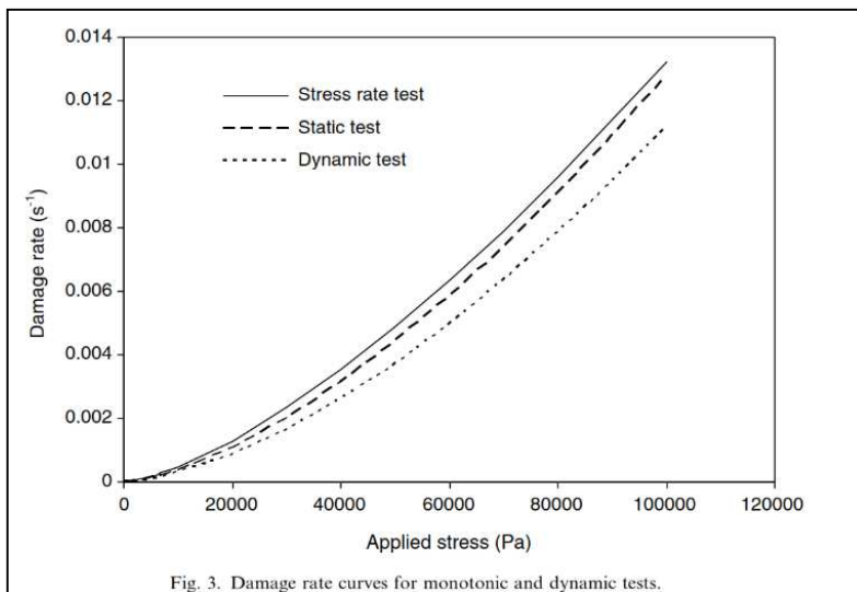
Abbildung 2.35: Zusammenhang zwischen Schadensrate und aufgebrachte Spannung bei statischen und zyklischen Versuchen nach Mo u.a. (2006)
