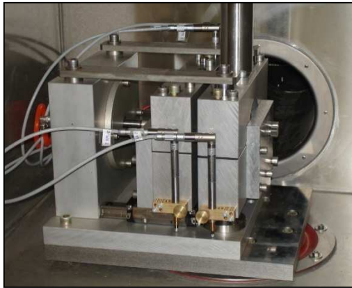
Abbildung 2.23: Prüfvorrichtung nach Wellner / Ascher (2007)
