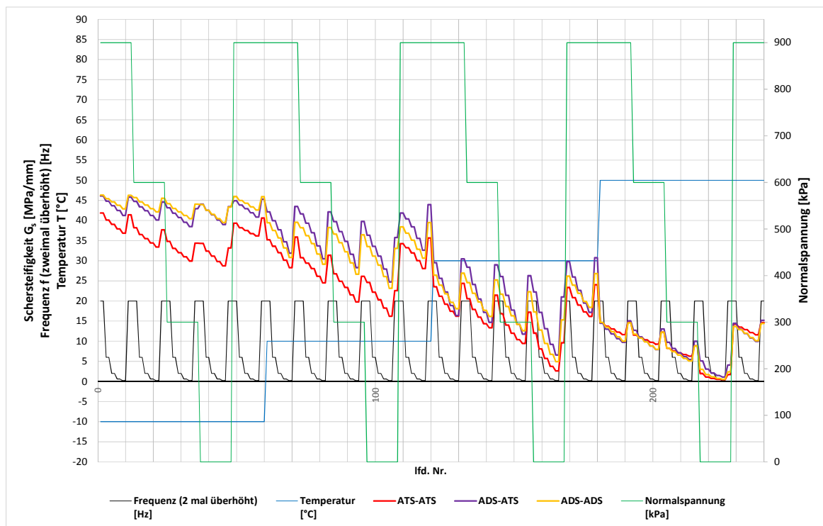
Abbildung 5.47: Mittelwerte der versuchstechnisch ermittelten Schersteifigkeiten bei Verbundkombinationen (1), (2) und (3) ohne Anwendung von Bitumenemulsion
