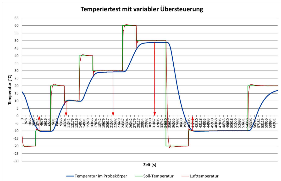
Abbildung 3.14: Verlauf der Temperatur im Asphaltprobekörper, der Soll- und der Lufttemperatur beim Versuch mit variablen Übersteuerungs- und Temperierungsdauer (Temperiertest Nr. 5)
