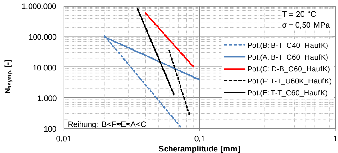
Abbildung 100. Wöhler-Linien für die Verbundvarianten A bis F bei einer Prüftemperatur von 20\text{ °C} und bei einer Normalspannung von 0,50\text{ MPa} mit einer Reihung der Verbundvarianten bezüglich der Scherermüdungsbeständigkeit.
