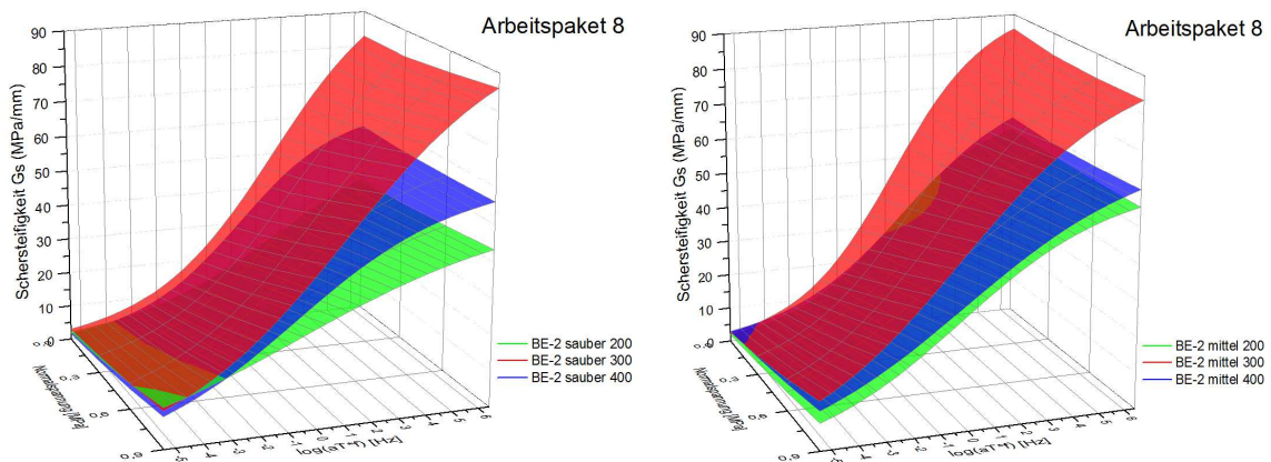
Abbildung 5.56: Vergleich der Flächenfunktionen der berechneten Schersteifigkeiten zwischen den drei Bitumenemulsionsmengen bei sauberer und mittelverschmutzter Oberfläche
