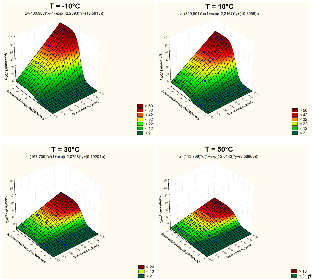
Abbildung 4.15: Flächenfunktionen bei -10°C, 10°C, 30°C und 50°C
