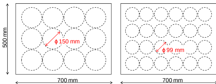
Abbildung 23. Bohrschema für die Probekörperentnahme aus den zweischichtig hergestellten Asphaltprobeplatten für die statischen Abscherversuch (links) und den zyklischen Scherversuch (rechts).
