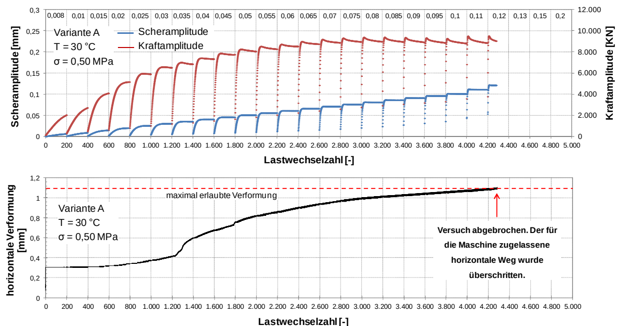
Abbildung 48. Verbundvariante A: Verläufe von Scher- und Kraftamplitude (oben) und Verlauf der horizontalen Verformung (unten) während des Amplitudensweeps bei 30 °C und 0,50 MPa Normalspannung.
