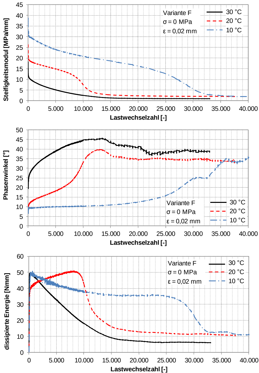
Abbildung 35. Verbundvariante F: Verläufe der Schersteifigkeit (oben), Phasenwinkel (Mitte) und dissipierten Energie pro Lastwechsel (unten) während des zyklischen Scherversuchs bei 0 MPa Normalspannung und 30 °C, 20 °C und 10 °C.
