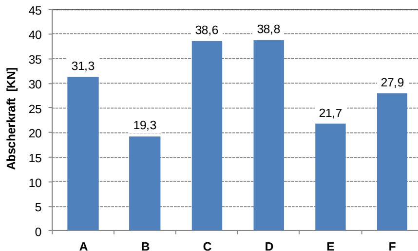
Abbildung 102. Verbundvarianten A bis F (gem. Tabelle 2): Abscherfestigkeiten [kN] ermittelt mit dem statischen Abscherversuch nach den TP Asphalt-StB Teil 80.
