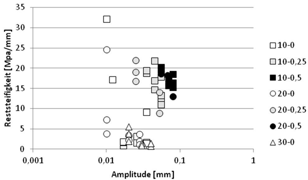
Abbildung 73. Verbundvariante D: Alle Werte der Restschersteifigkeit a_0 in Abhängigkeit von der Scheramplitude.
