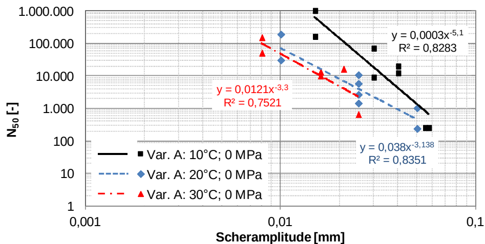
Abbildung 57. Wöhler-Linien für Verbundvariante A bei 0 MPa Normalspannung und bei den Prüftemperaturen 30 °C, 20 °C und 10 °C.
