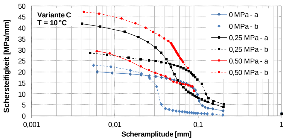
Abbildung 31. Verbundvariante C: Verläufe der Schersteifigkeiten bei drei Normalspannungen (0 MPa, 0,25 MPa und 0,50 MPa) während des Amplitudensweeps bei 10 °C.
