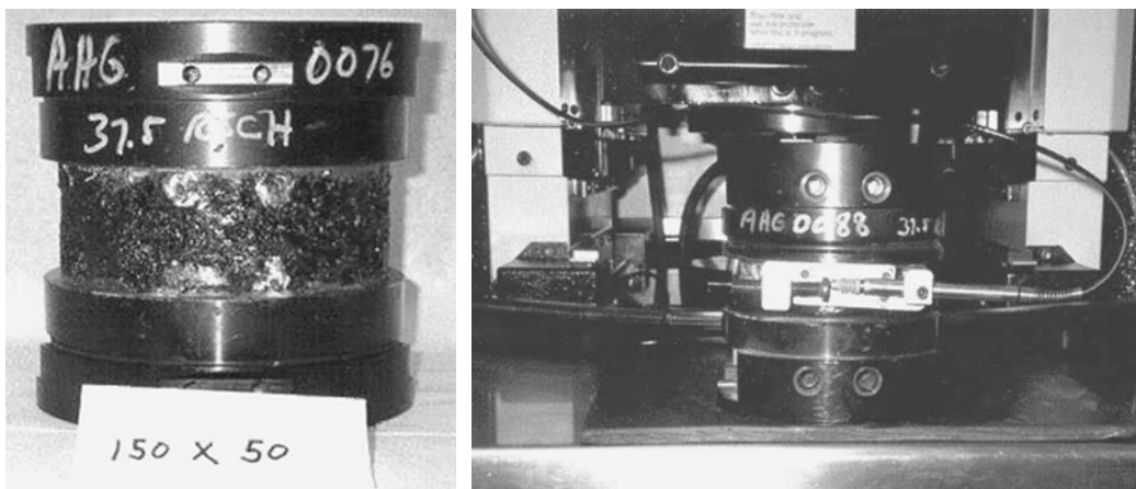
Abbildung 2.10: Probekörper und Prüfvorrichtung SST nach Witzak u.a. (2002)
