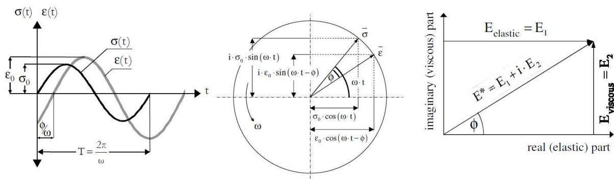
Abbildung 3. Spannungs- und Dehnungsdiagramm als Funktion der Zeit: Die resultierende Dehnung läuft der aufgebrachten konstanten Spannung zeitlich hinterher. Legende: \sigma(t) ...Spannung; \varepsilon(t) ...Dehnung, \phi ...Phasenverschiebung, T ...Periodendauer einer Oszillation, \omega ...Winkelgeschwindigkeit.
