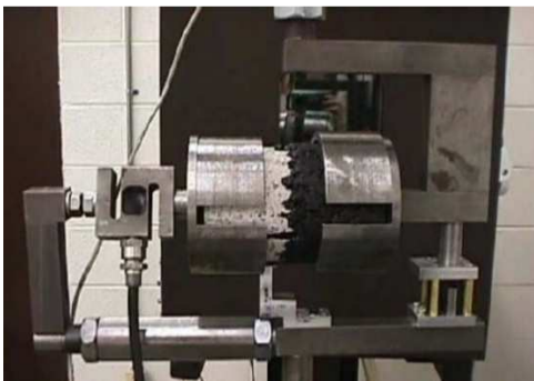
Abbildung 2.14: Virginia Tech Prüfvorrichtung nach Donovan u.a. (2000)
