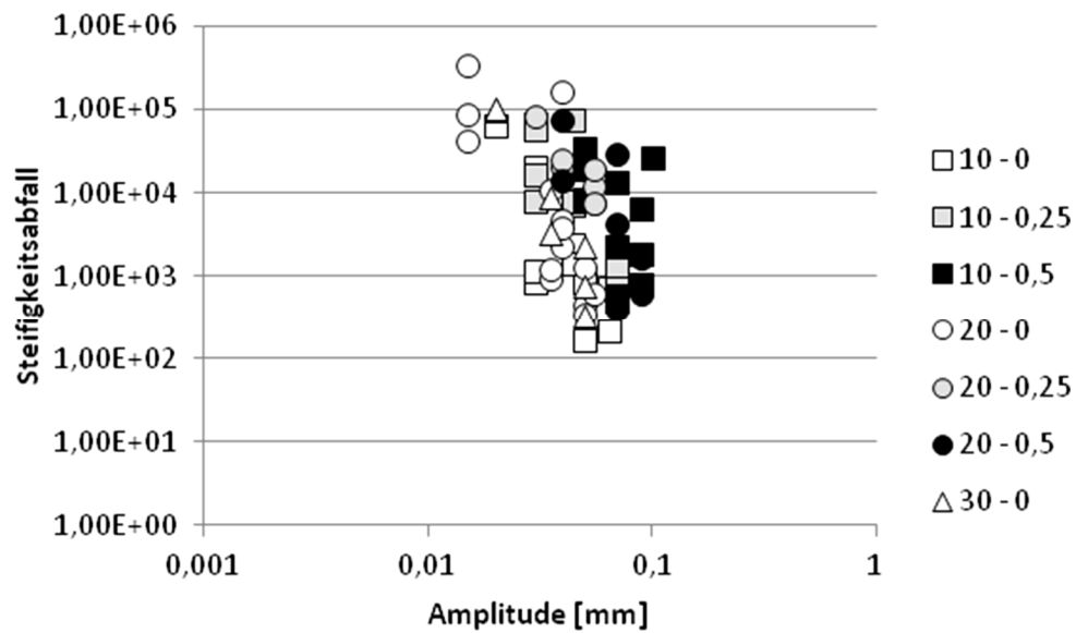
Abbildung 87. Verbundvariante C: Alle Werte des Schersteifigkeitsabfalls a_3 in Abhängigkeit von der Scheramplitude.
