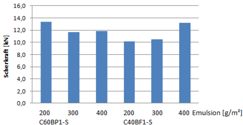
Abbildung 104. Abscherfestigkeiten [kN] ermittelt mit dem statischen Abscherversuch nach den TP Asphalt-StB Teil 80 für die Schicht-Kombination Deckschicht auf Tragschicht (D-T), kalt auf heiß eingebaut, bei geschliffenen Oberflächen und bei Variation der Art der Bitumenemulsion (C60BP1-S und C40BF1-S) und der jeweiligen Emulsionsmenge (200, 300 und 400 g/m 2 ).
