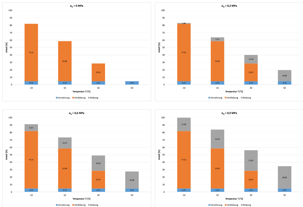
Abbildung 5.45: Anteile von Verklebung (orange), Verzahnung (blau) und Reibung (grau) für Verbundvariante (3) bei den vier Normalspannungen
