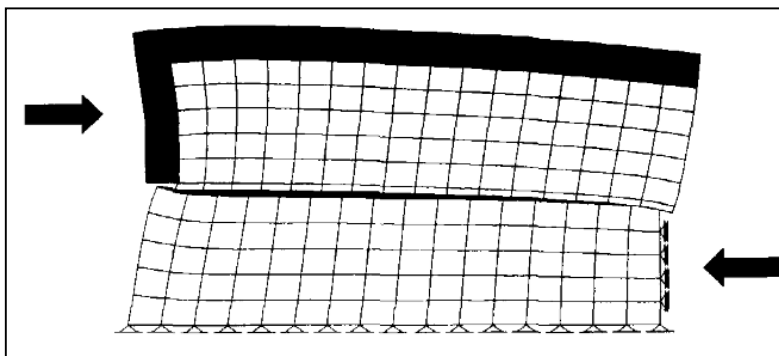
Abbildung 2.5: Typisches Verhalten des Probekörpers beim Versuch mit dem Prüfgerät „Shear Box“ (de Bondt, 1999)
