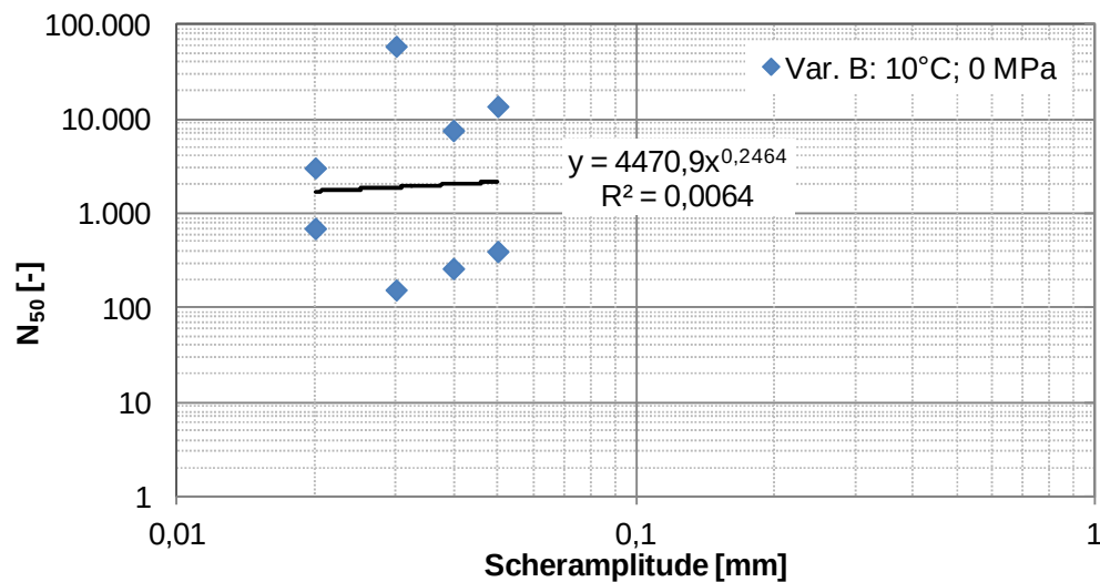
Abbildung 43. Verbundvariante B: Ermüdungspotenzfunktion (Wöhler-Linie) bei 10 °C und 0 MPa Normalspannung; fehlender Zusammenhang zwischen Scheramplitude und resultierender Scherermüdung ( N_{f/50} ).
