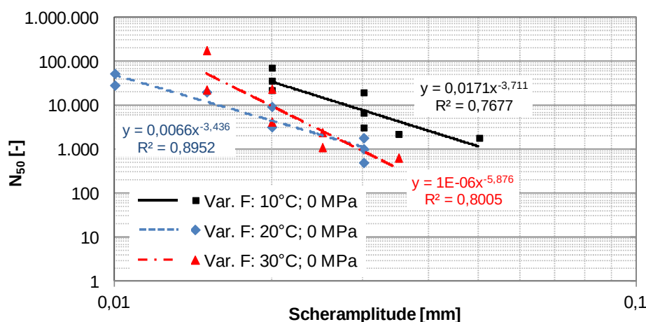
Abbildung 56. Wöhler-Linien für Verbundvariante F bei 0 MPa Normalspannung und bei den Prüftemperaturen 30 °C, 20 °C und 10 °C.
