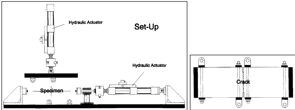
Abbildung 2.19: Schematische Darstellung des Prüfgerätes (links) und des Probekörpers (rechts) nach de Bondt (1999)
