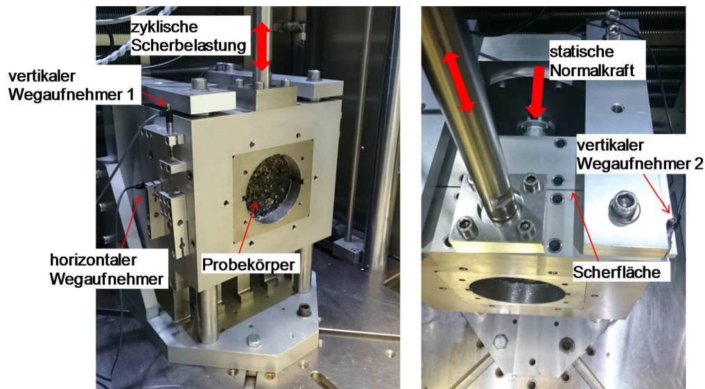
Abbildung 27. Zyklische Schervorrichtung am Institut für Straßenwesen der TU Braunschweig.
