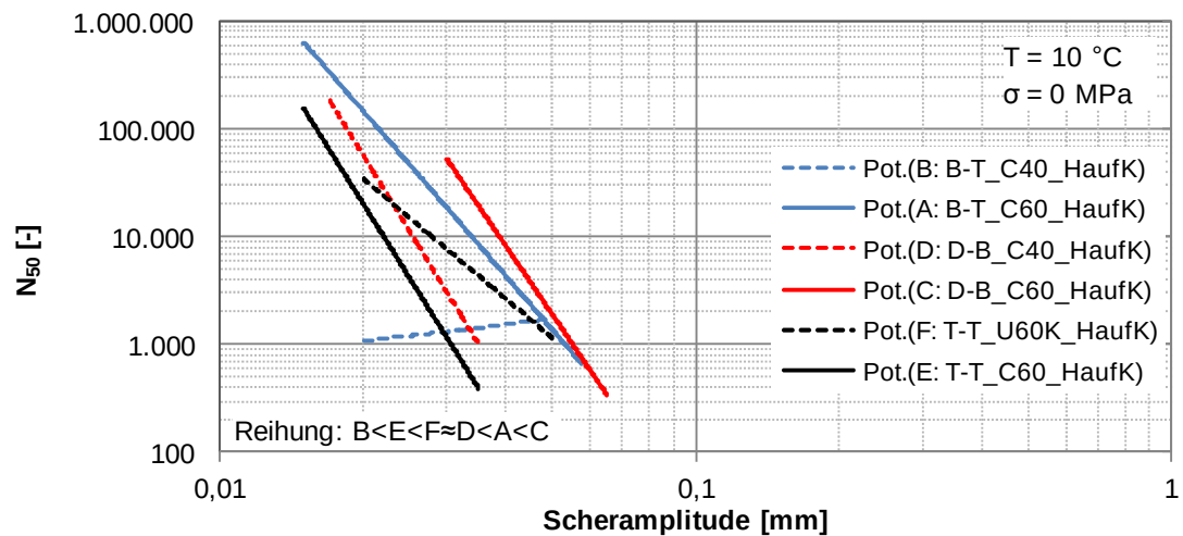
Abbildung 96. Wöhler-Linien für die Verbundvarianten A bis F bei einer Prüftemperatur von 10 °C und ohne Normalspannung mit einer Reihung der Verbundvarianten bezüglich der Scherermüdungsbeständigkeit.
