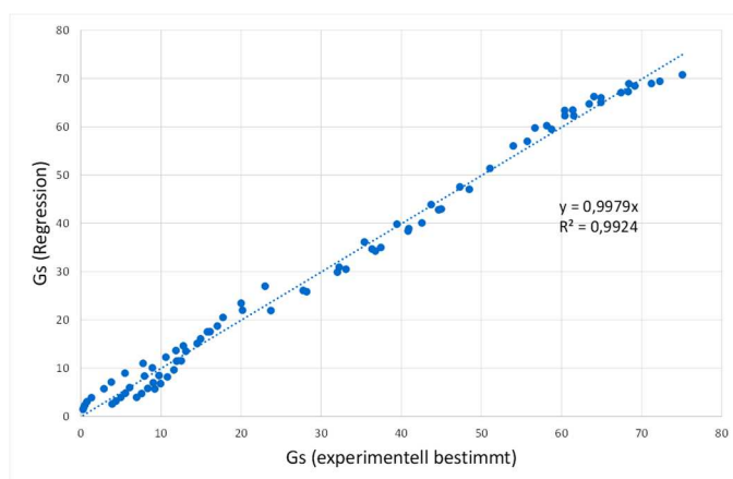
Abbildung 4.9: Vergleich zwischen der versuchstechnisch ermittelten Schersteifigkeit und der nach Gleichung 24 berechneten Schersteifigkeit
