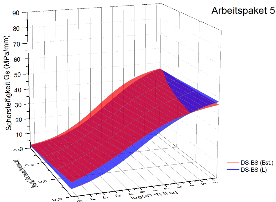
Abbildung 5.35: Vergleich zwischen den Flächenfunktionen der berechneten Schersteifigkeiten für die Kombination ADS-ABS zwischen Baustelle und Laboratorium
