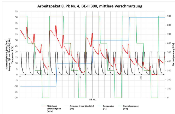
Abbildung 4.5: Beispiel eines gebrochenen Schichtenverbundes
