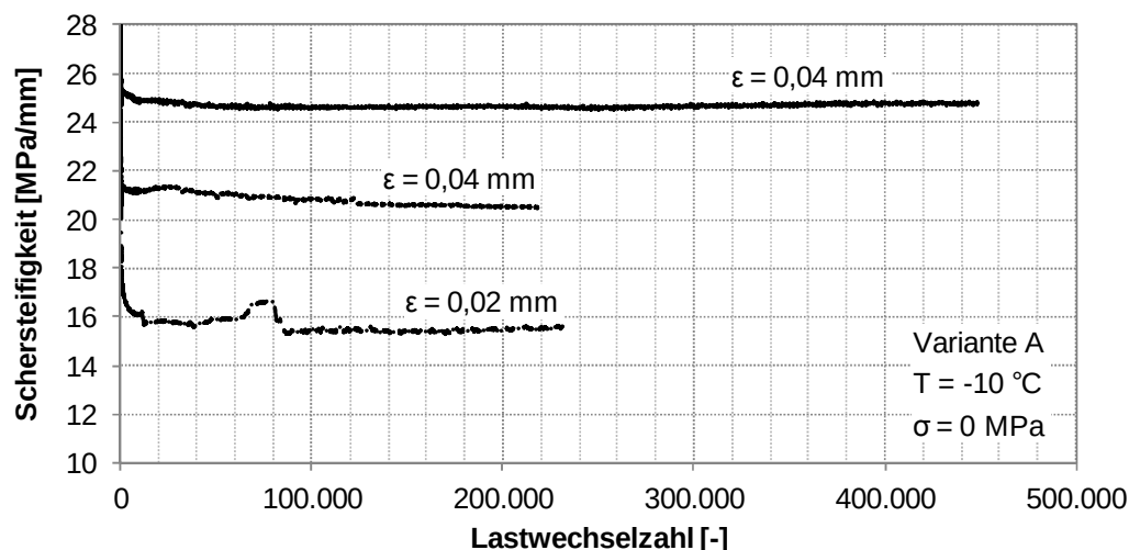
Abbildung 54. Verbundvariante A: Verläufe der Schersteifigkeit während der Scherermüdungsprüfung bei -10 °C, bei 0 MPa Normalspannungen und bei zwei Scheramplituden (0,02 mm und 0,04 mm).
