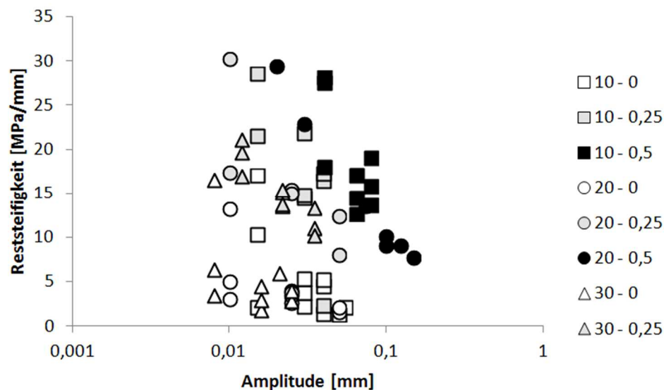
Abbildung 63. Verbundvariante A: Alle Werte der Restschersteifigkeit a_0 in Abhängigkeit von der Scheramplitude.
