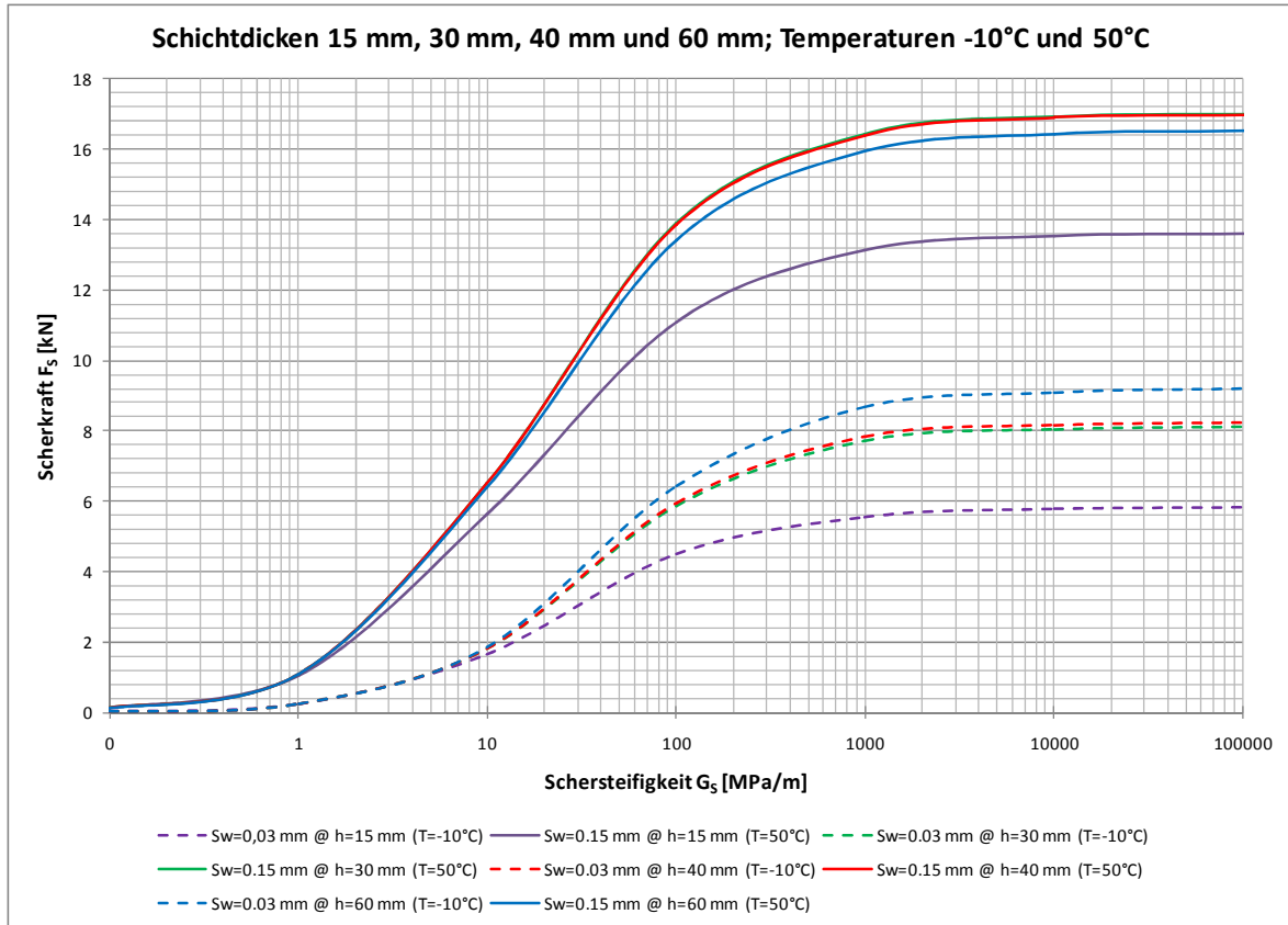
Abbildung 5.11: Funktionaler Zusammenhang zwischen Scherkraft und Schersteifigkeit für der vier Schichtdicken bei -10°C und 50°C
