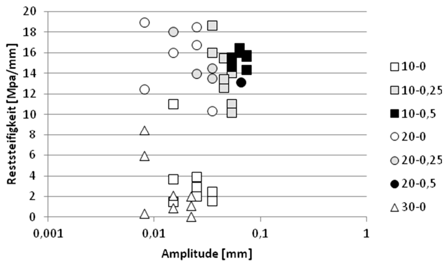
Abbildung 74. Verbundvariante E: Alle Werte der Restschersteifigkeit a_0 in Abhängigkeit von der Scheramplitude.
