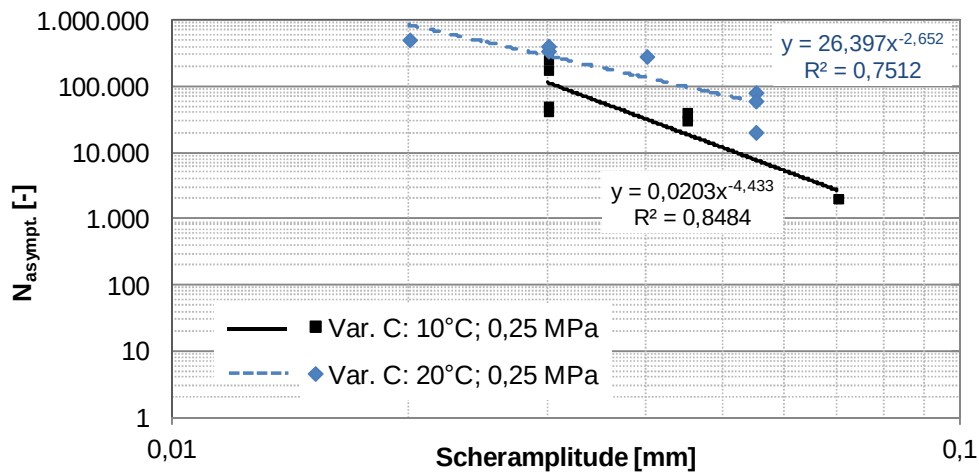
Abbildung 60. Wöhler-Linien für Verbundvariante C bei 0,25 MPa Normalspannung und bei den Prüftemperaturen 20 °C und 10 °C.
