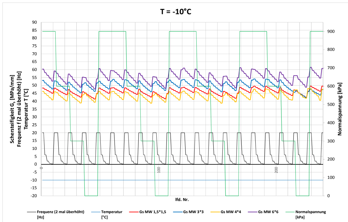
Abbildung 5.22: Schersteifigkeitsverläufe für die vier untersuchten Schichtdicken bei -10°C
