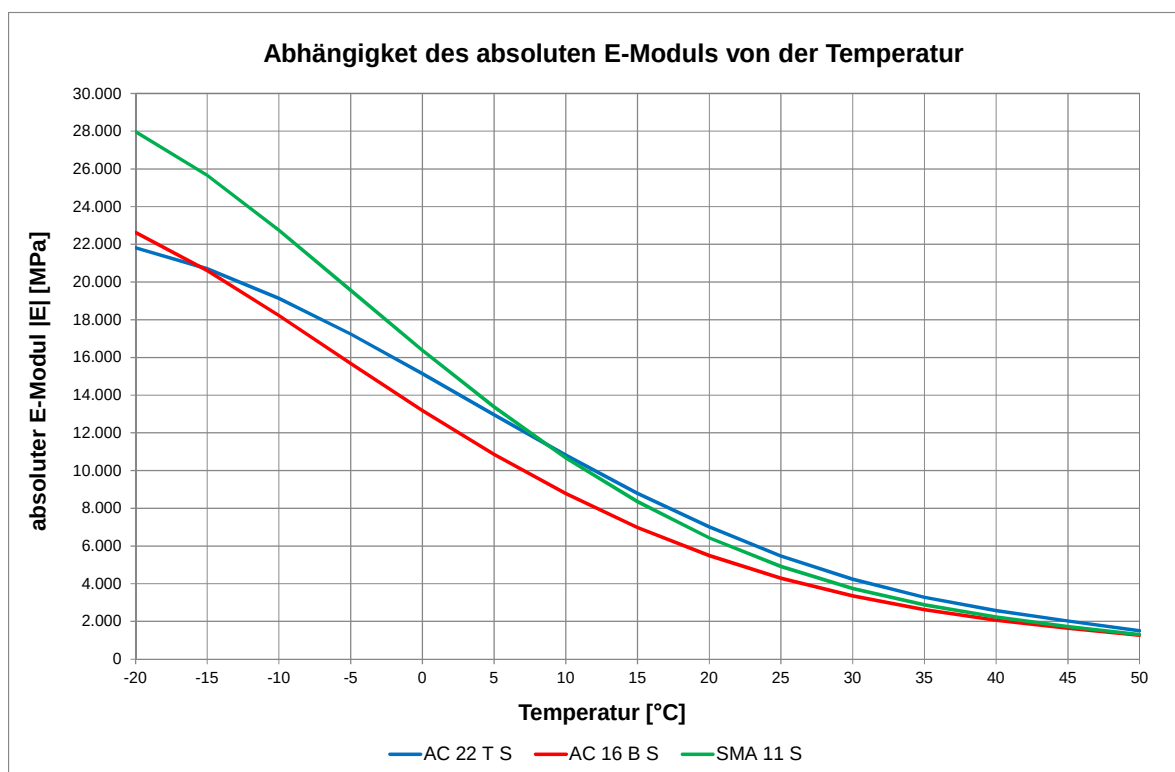
Abbildung 5.72: Steifigkeitsmodul-Temperaturfunktionen für SMA 11 S, AC 16 B S, AC 22 T S
