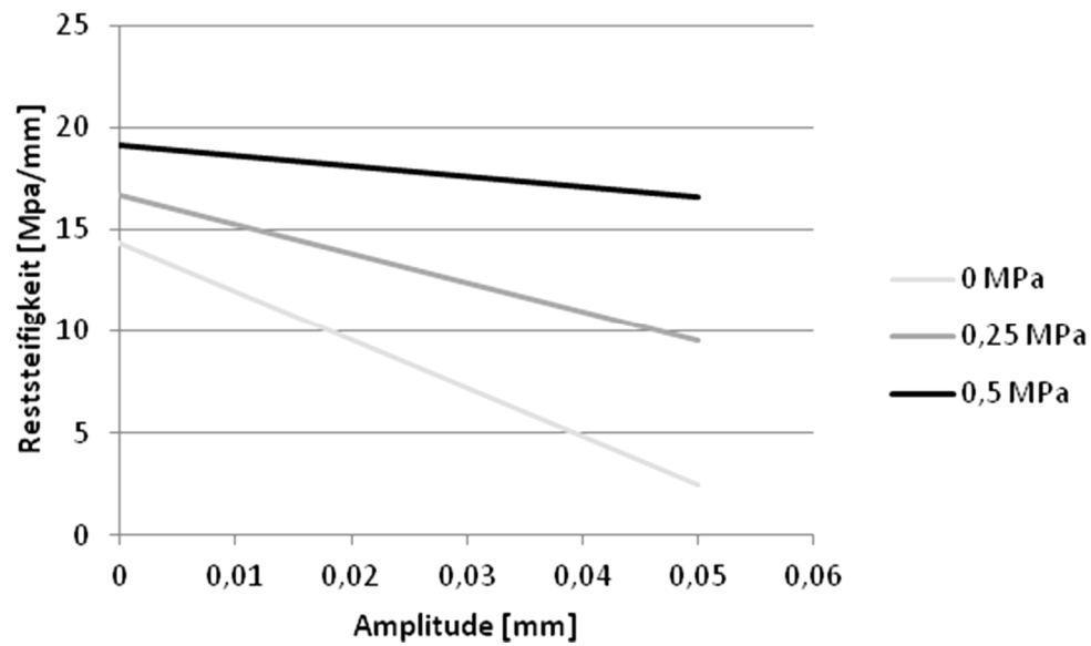
Abbildung 78. Verbundvariante D: Abhängigkeit der Restschersteifigkeit a_0 von der Normalspannung und der Scheramplitude.
