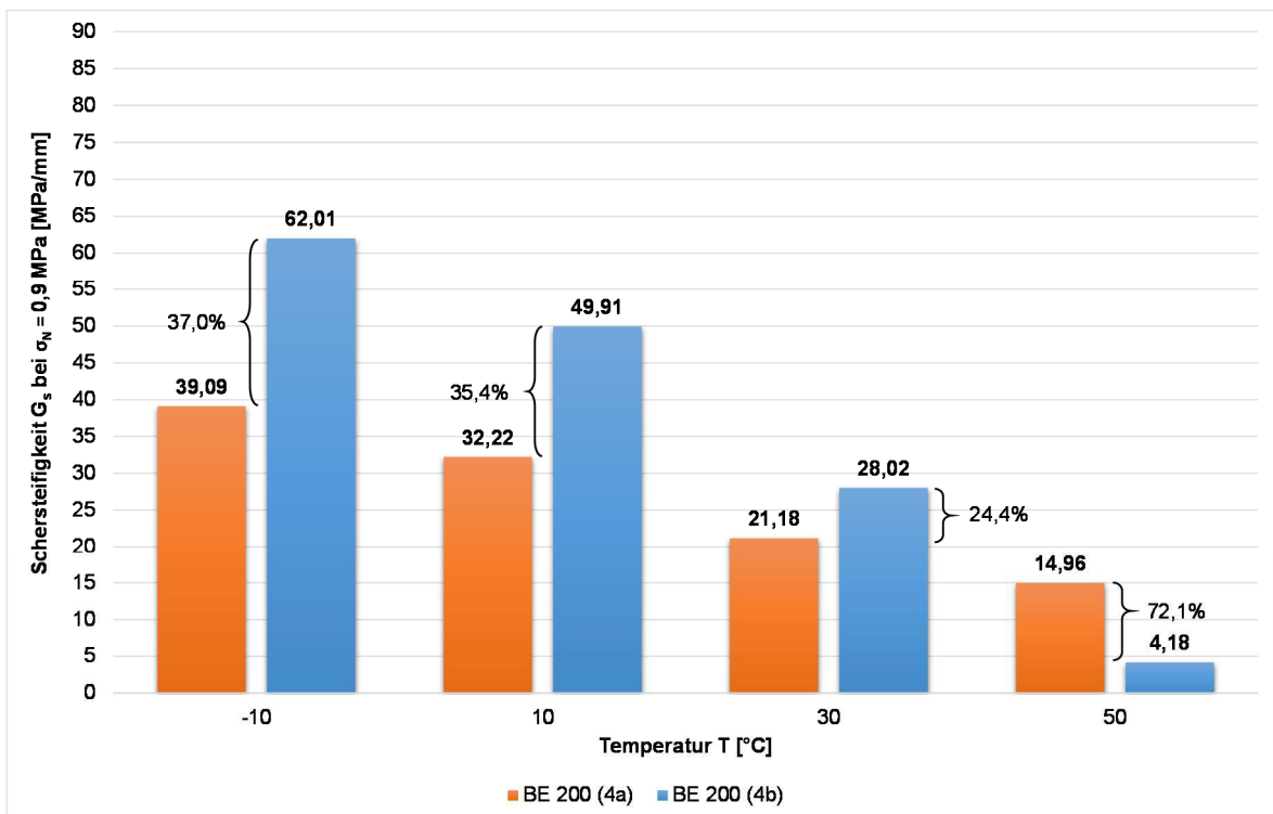
Abbildung 5.33: Vergleich der optimalen Schersteifigkeiten bei reiner Verklebung und bei dem kombinierten Effekt aus Verklebung, Verzahnung und Reibung (200 g/m 2 C60 BP1-S, \sigma_N = 0,9 MPa und f = 10 Hz)
