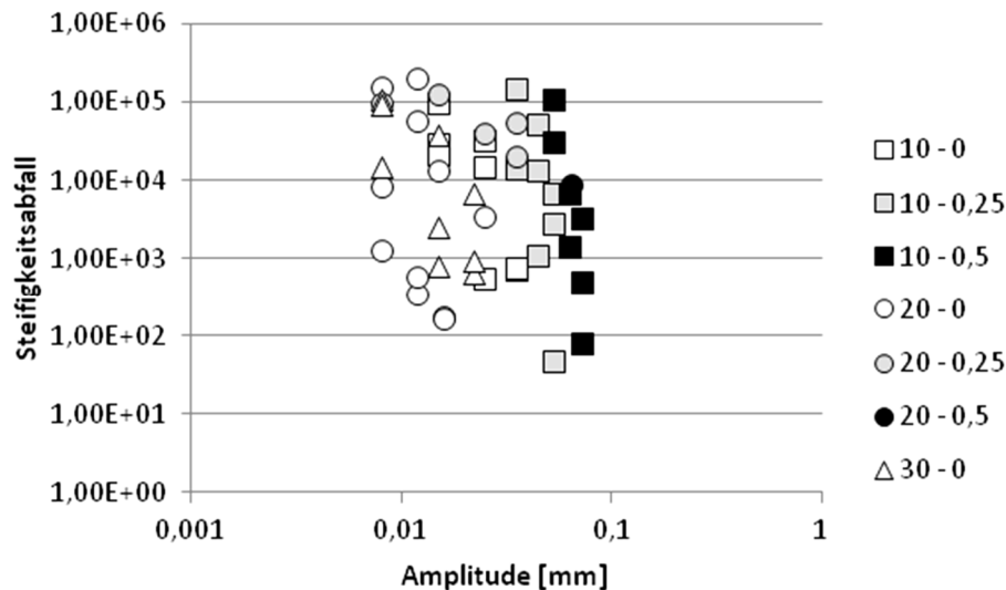
Abbildung 89. Verbundvariante E: Alle Werte des Schersteifigkeitsabfalls a_3 in Abhängigkeit von der Scheramplitude.
