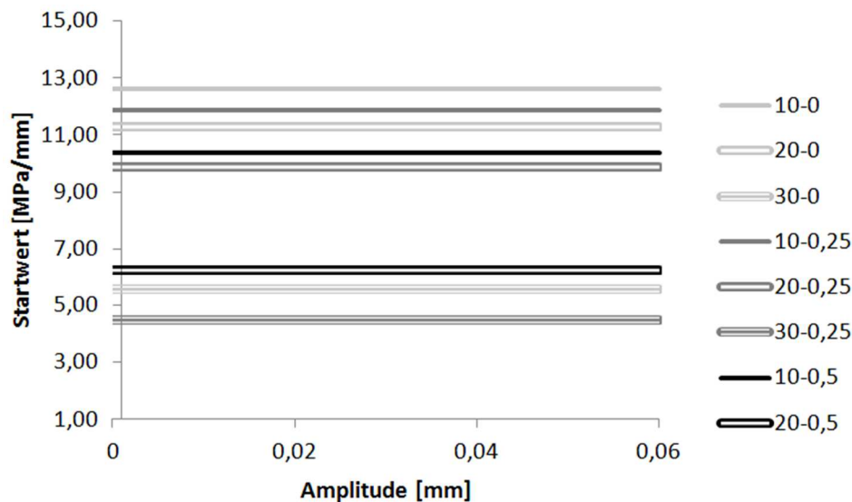
Abbildung 68. Verbundvariante A: Mittlere Startwerte der Schersteifigkeit a_1 .
