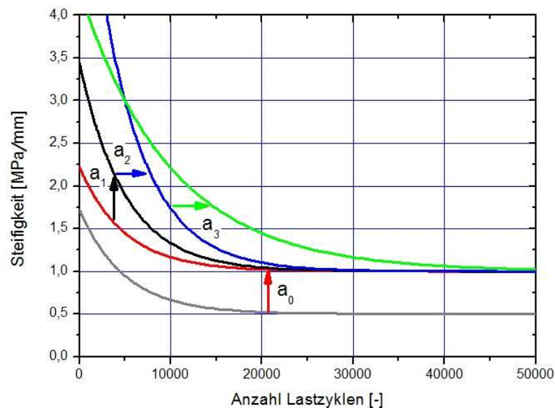
Abbildung 5.59: Ermüdungsfunktionen für den Schichtenverbund
