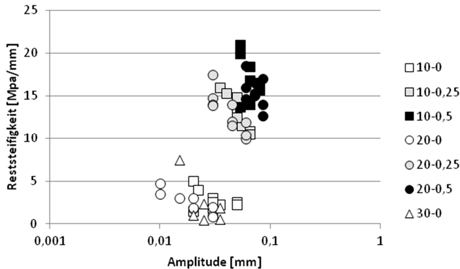
Abbildung 75. Verbundvariante F: Alle Werte der Restschersteifigkeit a_0 in Abhängigkeit von der Scheramplitude.
