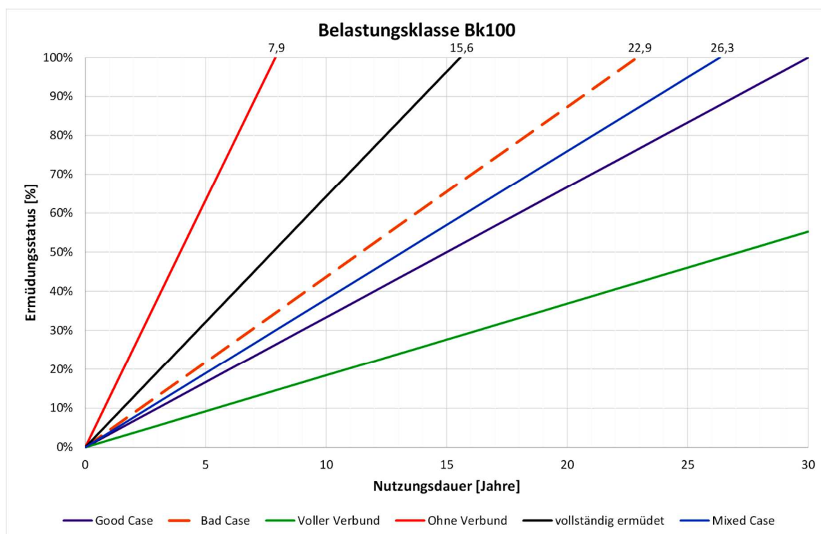
Abbildung 5.65: Verlauf des Ermüdungsstatus bei unterschiedlichen Schichtenverbundfunktionen über die gesamte Nutzungsdauer bei Bk100
