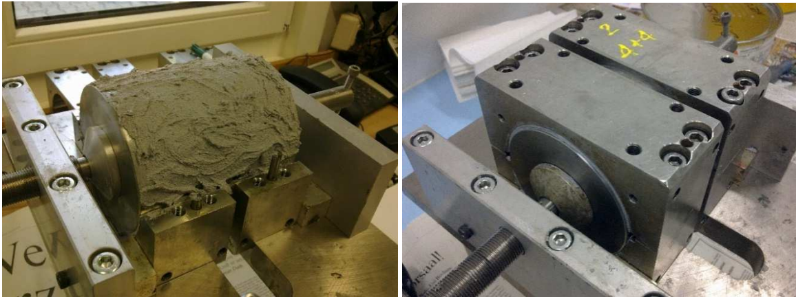
Abbildung 5.8: Einkleben eines 80 mm langen zweischichtigen Asphaltprobekörpers und zwei Stahldummies
